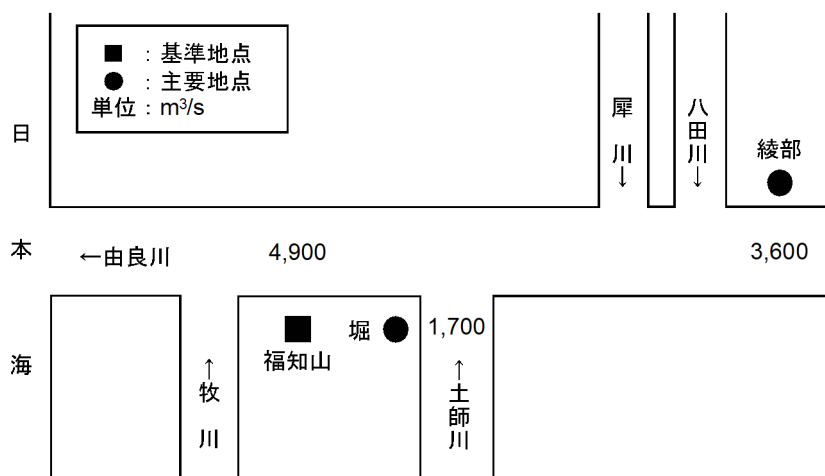
図 4-6 平成25年 由良川水系河川整備計画 流量配分図（河道配分流量）
