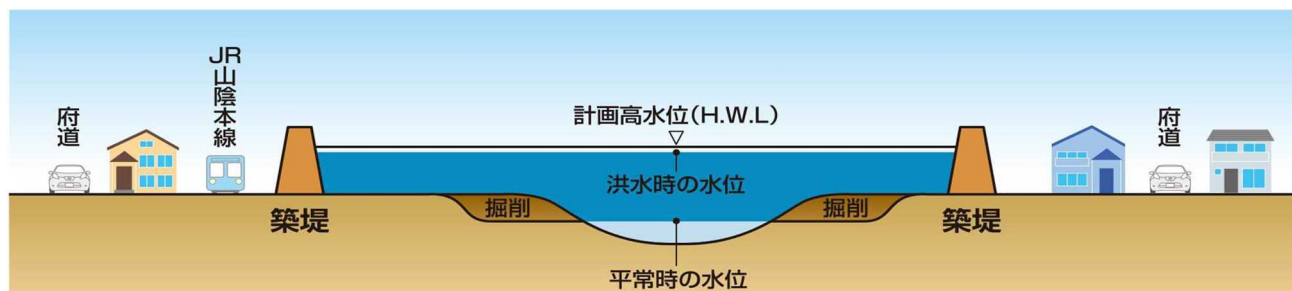
図 4-7 中流部改修事業のイメージ
