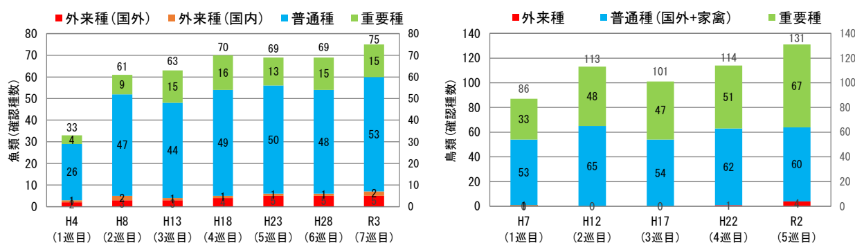
図 2-3 生物相の経年変化（左：魚類、右：鳥類）
