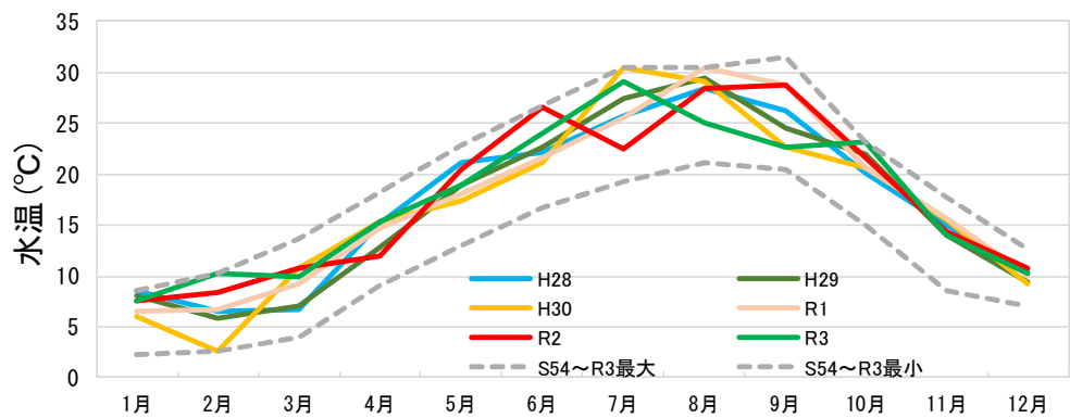
図 2-7 水温（音無瀬橋）の経月変化
