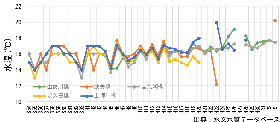
図 2-6 年平均水温の経年変化
