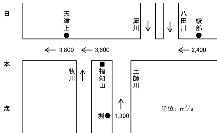
図 4-5 平成15年 由良川水系河川整備計画 流量配分図（河道配分流量）
