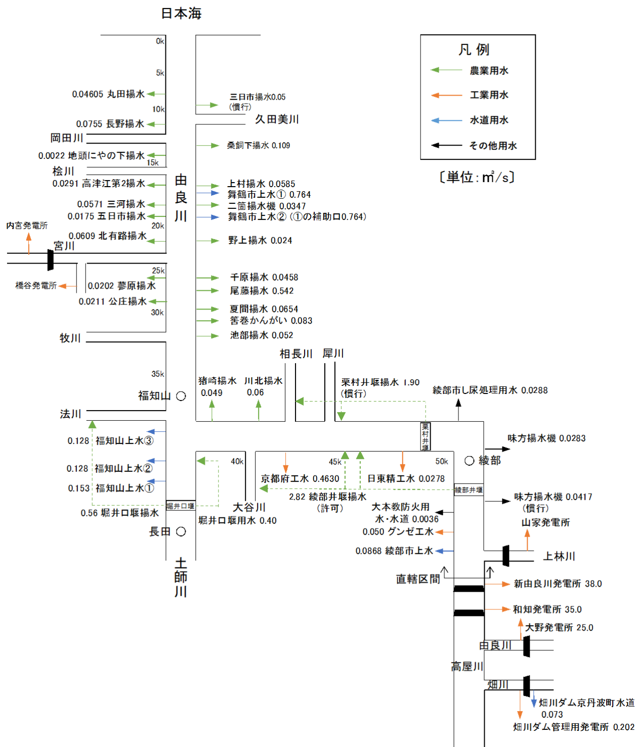
図 5-2 由良川水系の水利模式図
