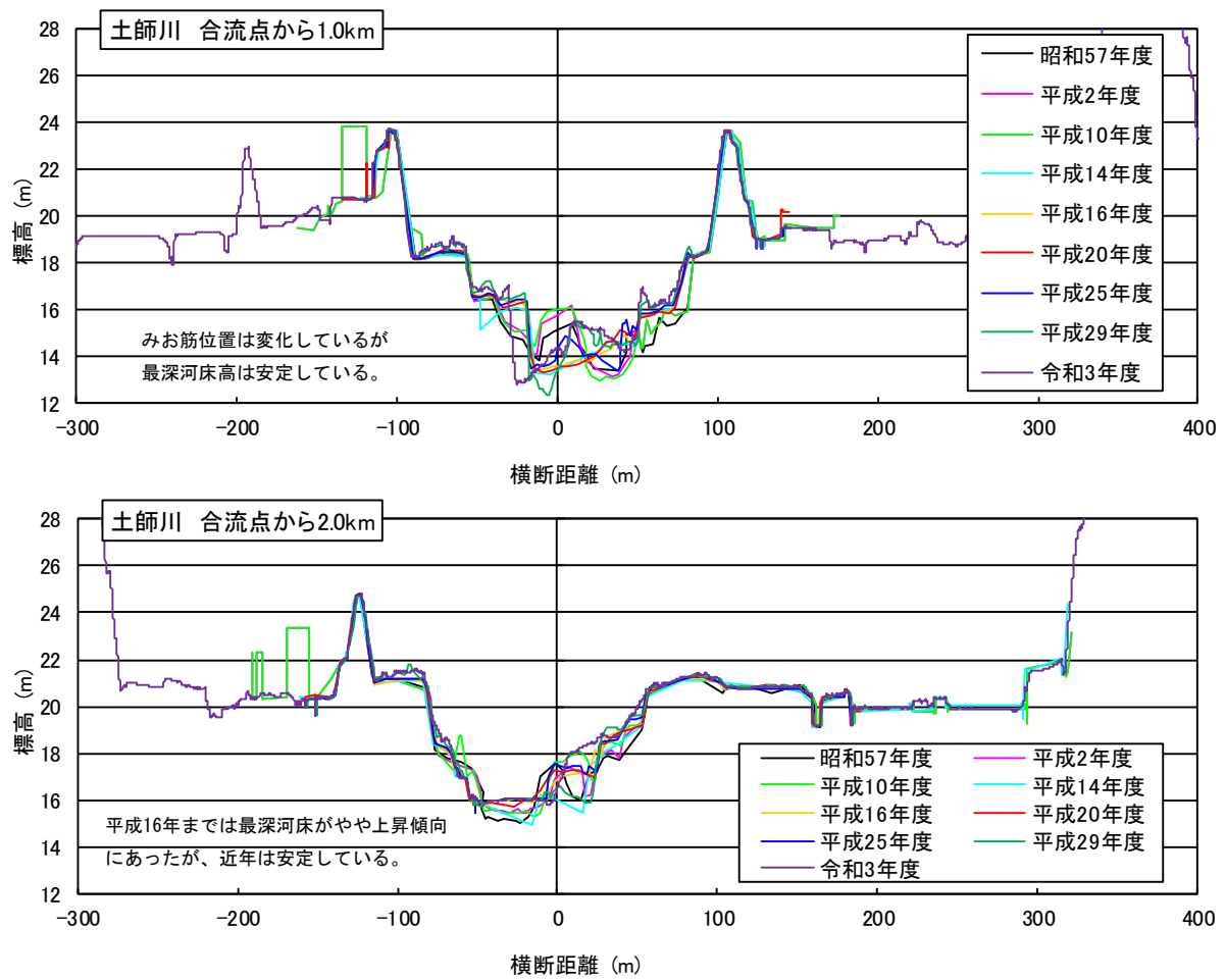
図 8-5 土師川の横断図の経年変化
