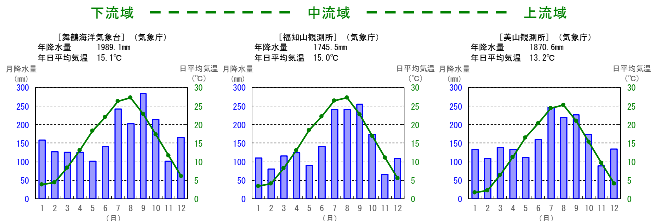
図 1-5 月別の月降水量と日平均気温（2013～2022の平均値）
