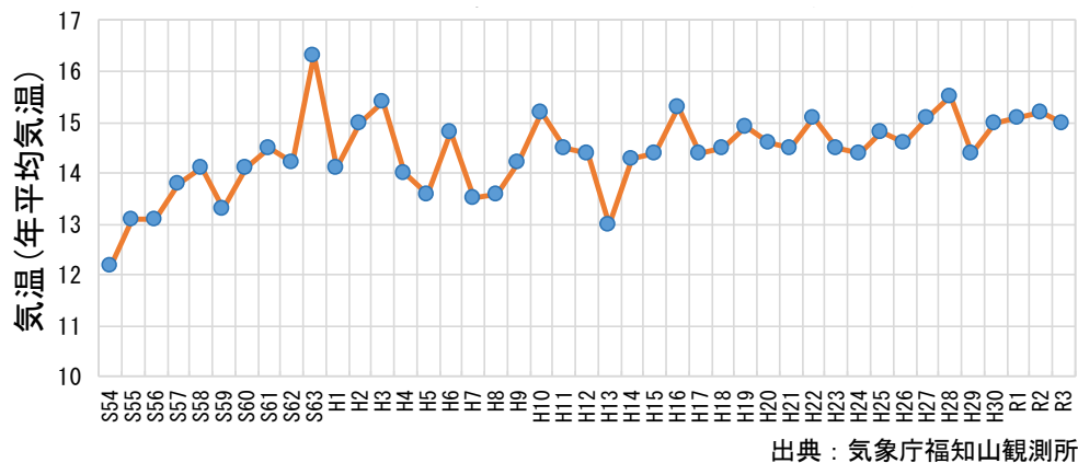
図 2-5 年平均気温の経年変化
