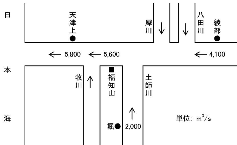
図 4-4 平成11年 由良川水系河川整備基本方針 計画高水流量配分図
