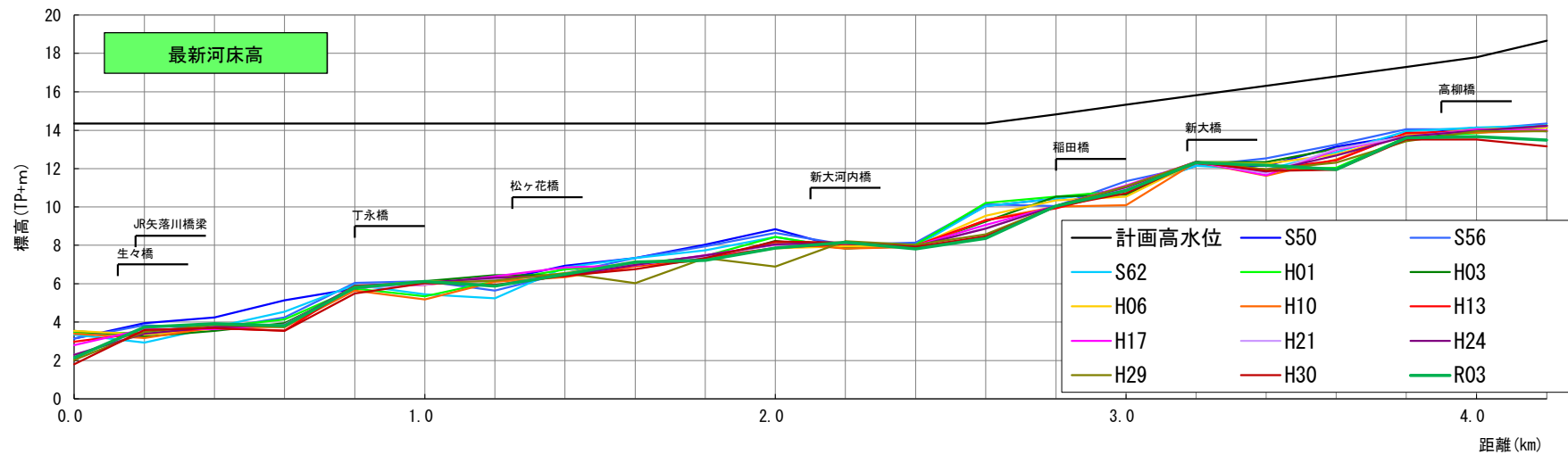
図 4.4 平均河床高・最深河床高縦断図：矢落川
