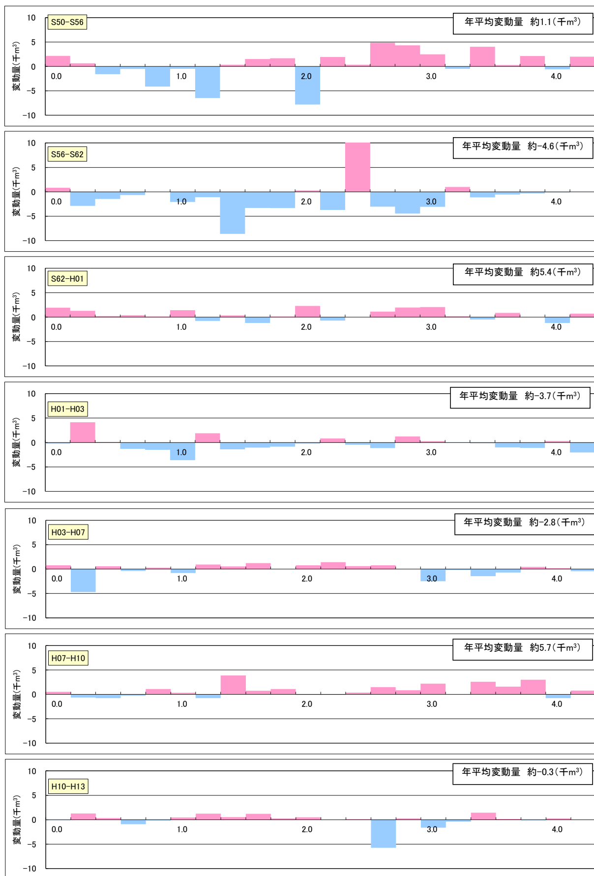
図 4.2 (1/2) 河床変動量：矢落川（昭和 50 年～平成 13 年）
