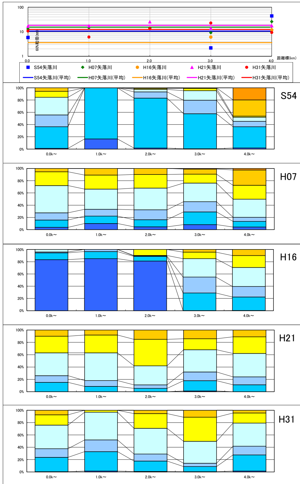
図 4.7 D_{60} 粒径・粒径比率の縦断分布：矢落川
