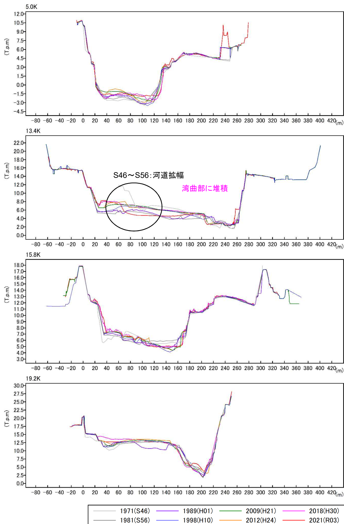
図 4.5 (1) 代表横断面図：肱川
