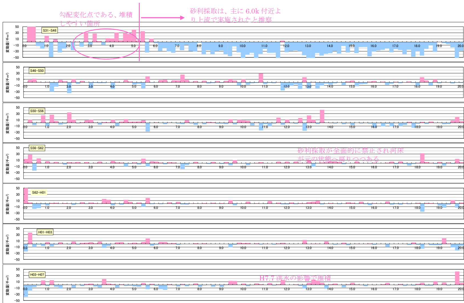
図 4.1 (1/2) 河床変動量：肱川（昭和 31 年～平成 7 年）
