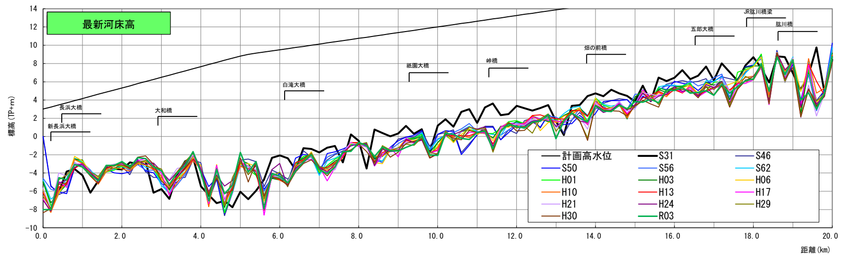
図 4.3 平均河床高・最深河床高縦断面図：肱川
