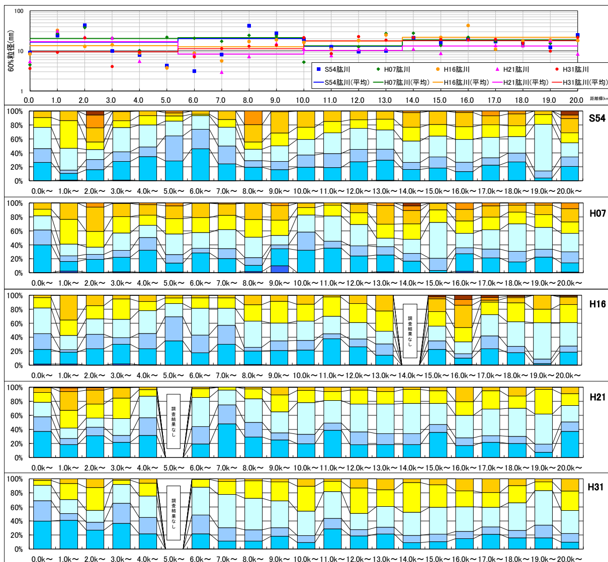
図 4.6 D_{60} 粒径・粒径比率の縦断分布：肱川
