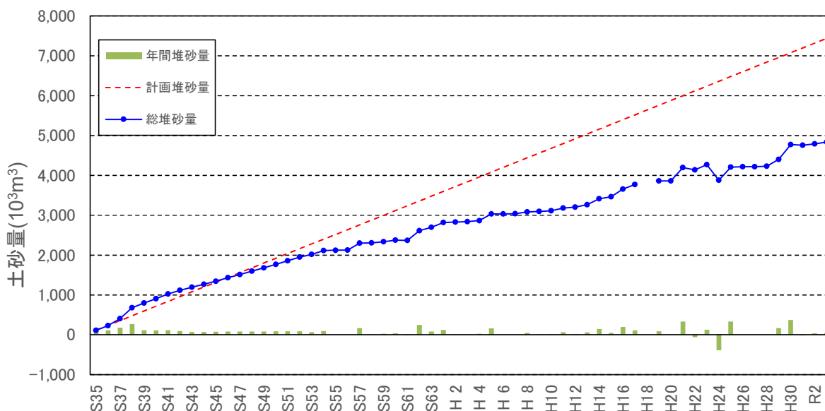
図 3.3 野村ダム堆砂量の経年変化
