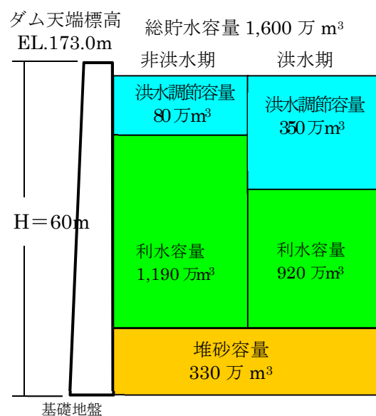
図 3.1 野村ダム容量配分図
