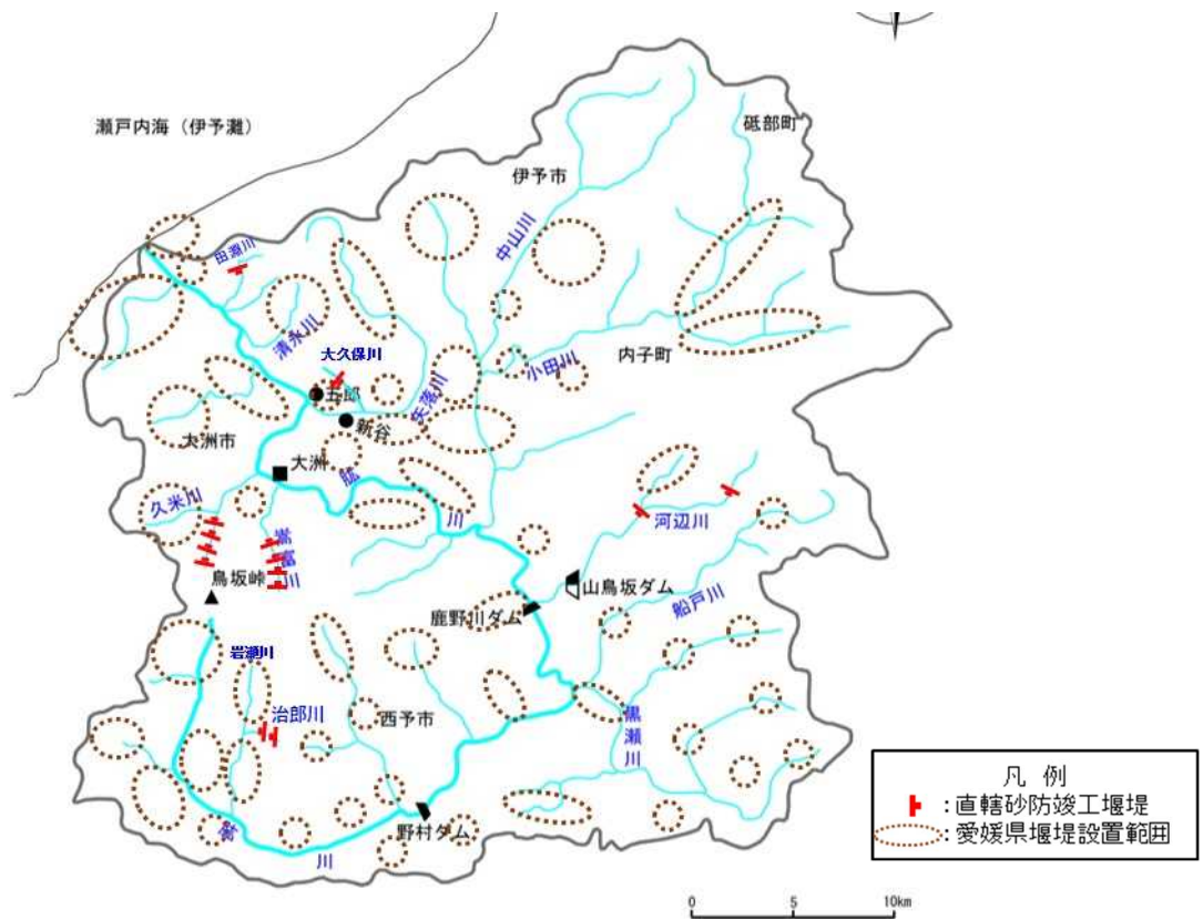
図 2.4 肱川水系の砂防事業位置図
