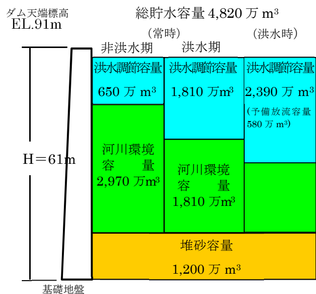
図 3.2 鹿野川ダム容量配分図
