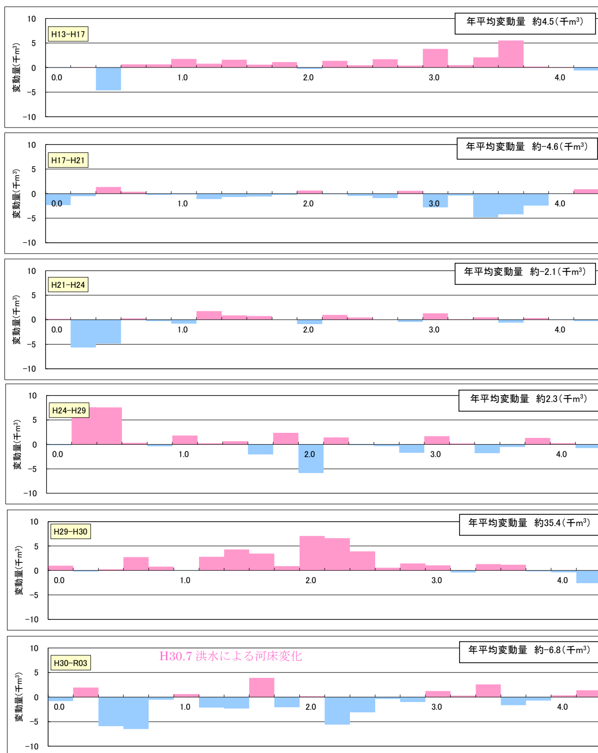
図 4.2 (2/2) 河床変動量：矢落川（平成 10 年～令和 3 年）
