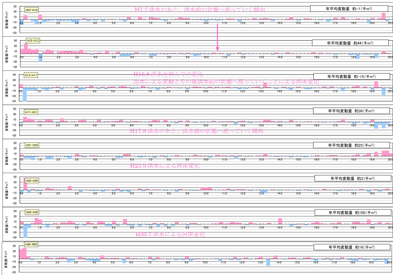
図 4.1 (2/2) 河床変動量：肱川（平成7年～令和3年）
