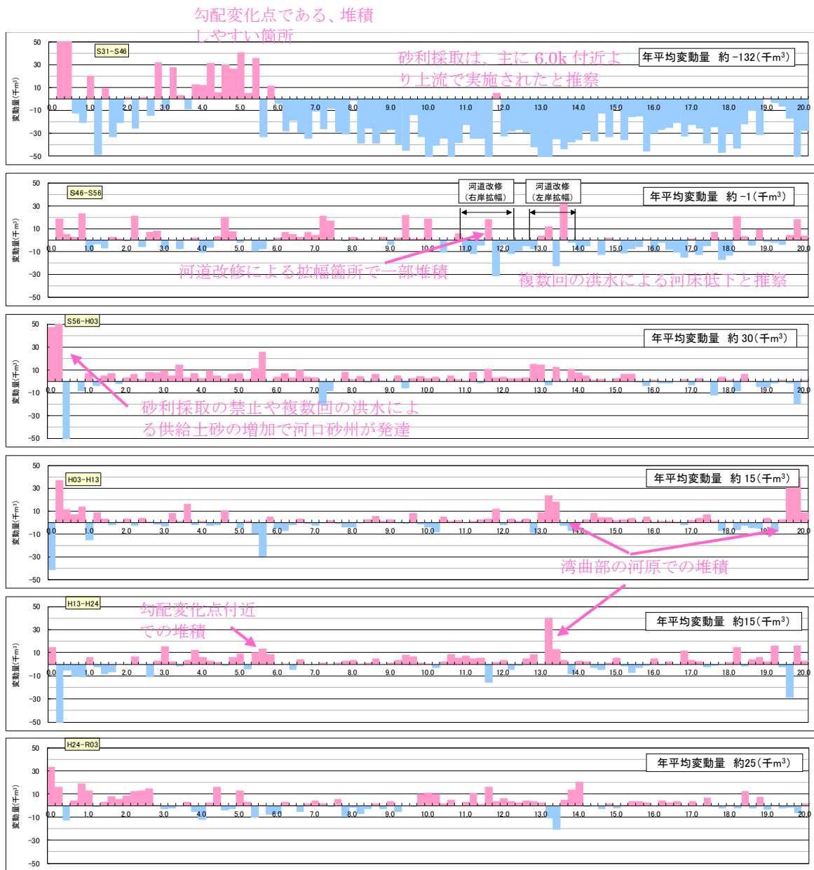
図 4.1 (3/3) 河床変動量：肱川（昭和 31 年～令和 3 年、概ね 10 年間隔）
