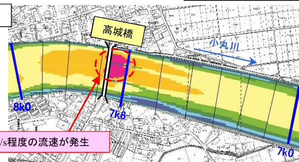
河道掘削+断面拡大
