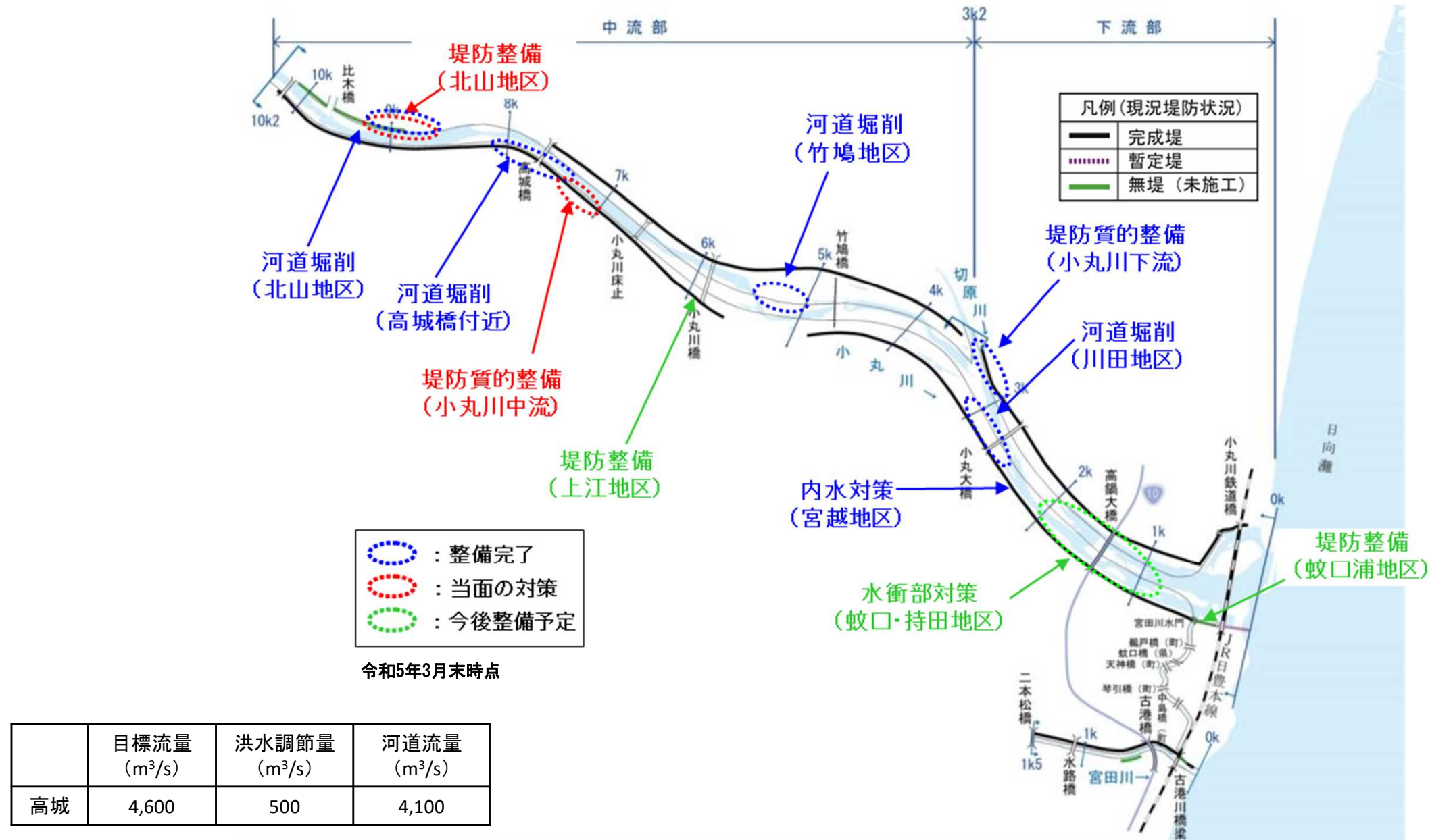
小丸川水系河川整備計画の主要メニュー箇所位置図
