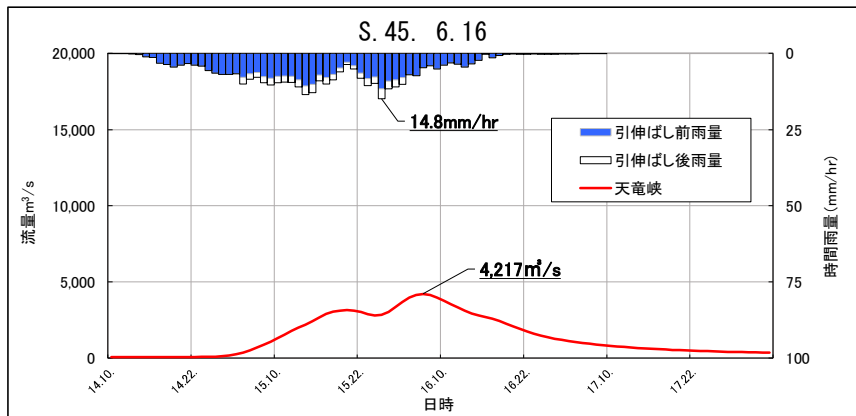
図 1.18 (4) 基本高水ハイドログラフ(昭和 45 年 6 月洪水 天竜峡)
