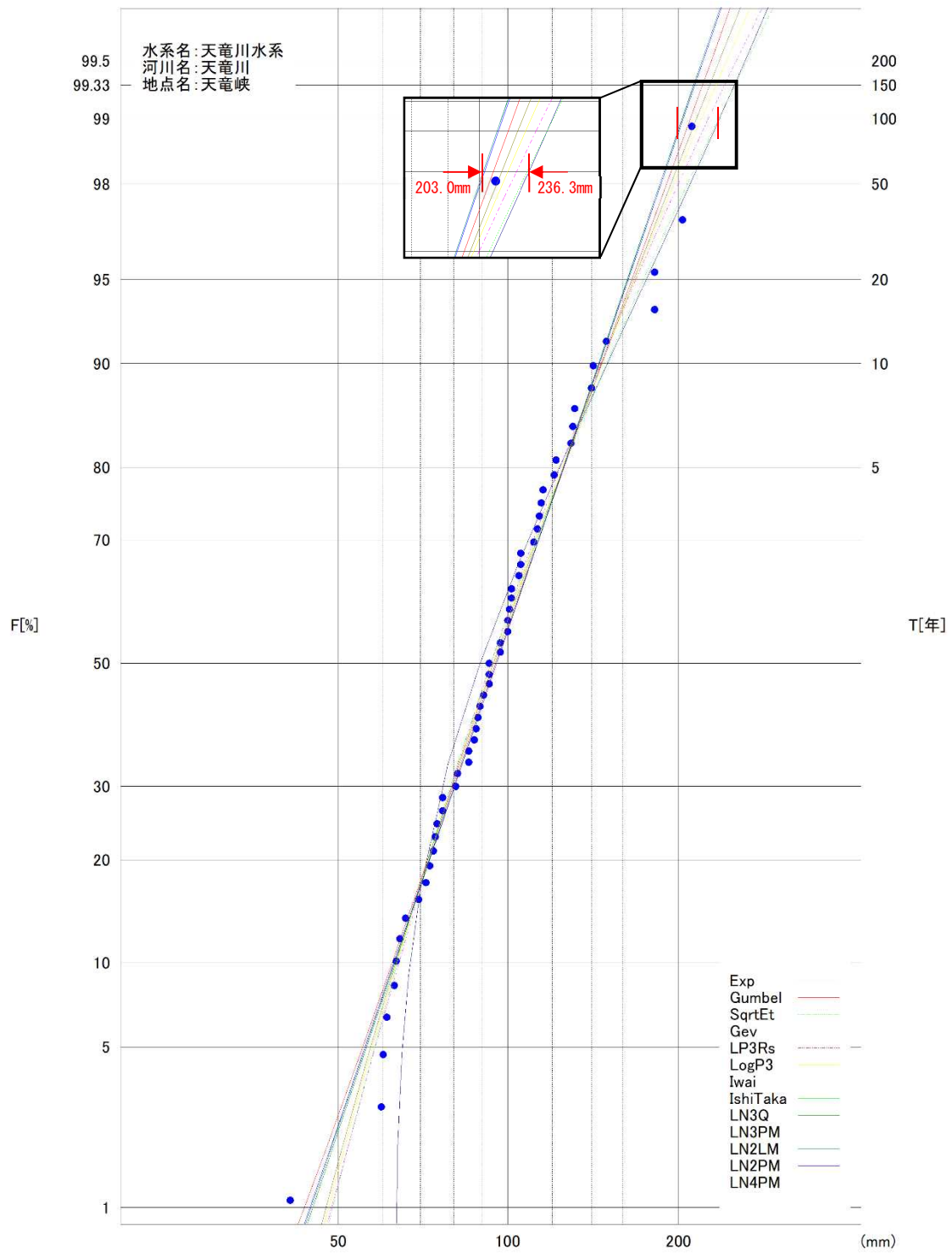
图 1.9 (1) 基準地点天竜峽 24 時間雨量確率図 (昭和 31 年(1956 年)~平成 22 年(2010 年): 55 年)
