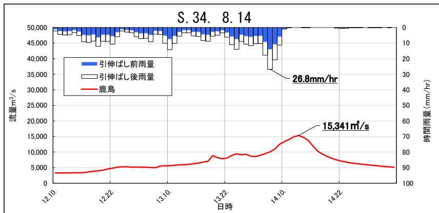
図 1.18 (17) 基本高水ハイドログラフ(昭和 34 年 8 月洪水 鹿島)
