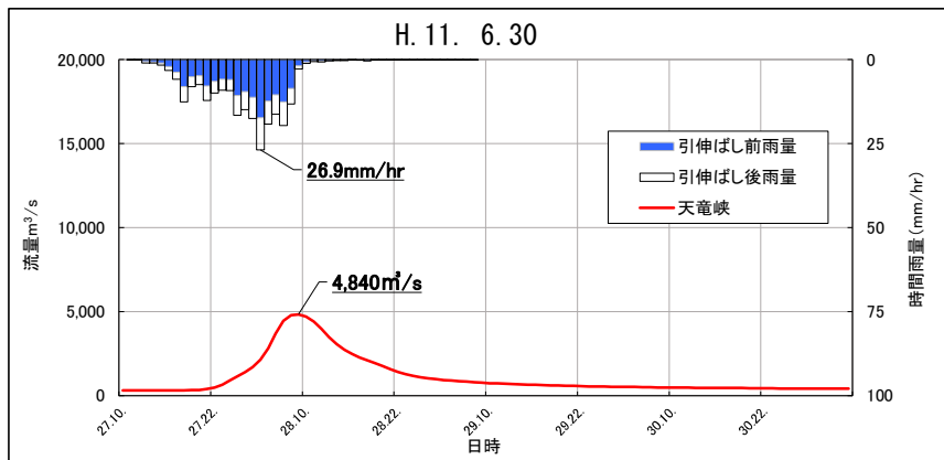
図 1.18 (10) 基本高水ハイドログラフ(平成 11 年 6 月洪水 天竜峡)
