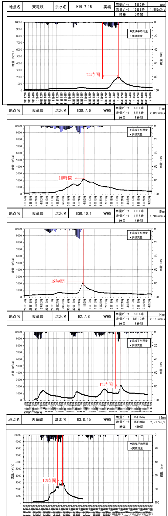
図 1.4 (2) Kinematic Wave 法による洪水到達時間(基準地点天竜峡)
