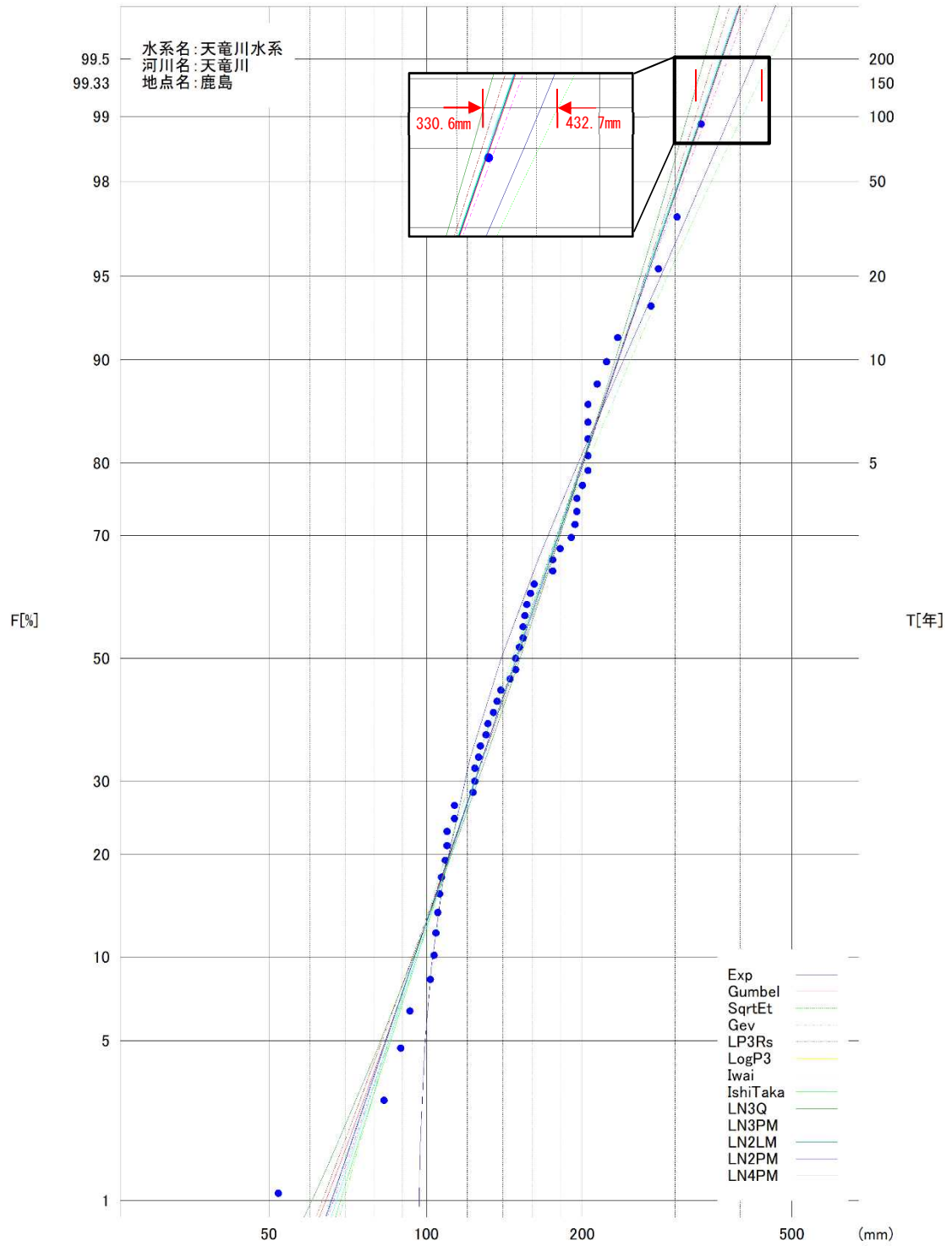
图 1.9 (2) 基準地点鹿島 48 時間雨量確率図 (昭和 31 年(1956 年)~平成 22 年(2010 年): 55 力年)
