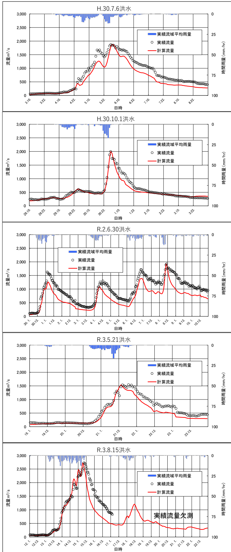
图 1.12 (1) 再現計算結果(宮ヶ瀬)
