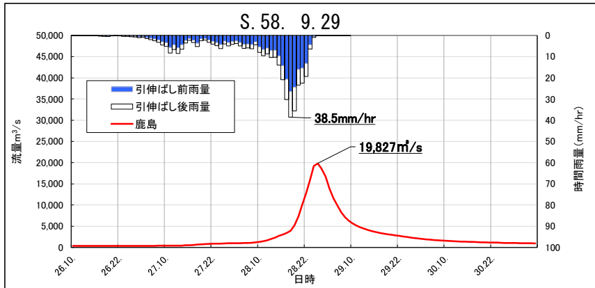
図 1.18 (21) 基本高水ハイドログラフ(昭和 58 年 9 月洪水 鹿島)
