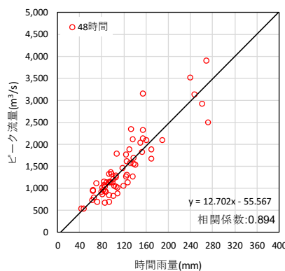
図 1.7 (2) ピーク流量と雨量の相関図
