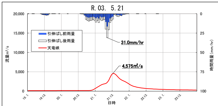
図 1.18 (14) 基本高水ハイドログラフ(令和 3 年 5 月洪水 天竜峡)
