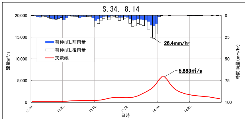
図 1.18 (2) 基本高水ハイドログラフ(昭和 34 年 8 月洪水 天竜峡)
