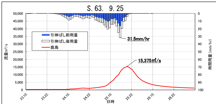
図 1.18 (23) 基本高水ハイドログラフ(昭和 63 年 9 月洪水 鹿島)
