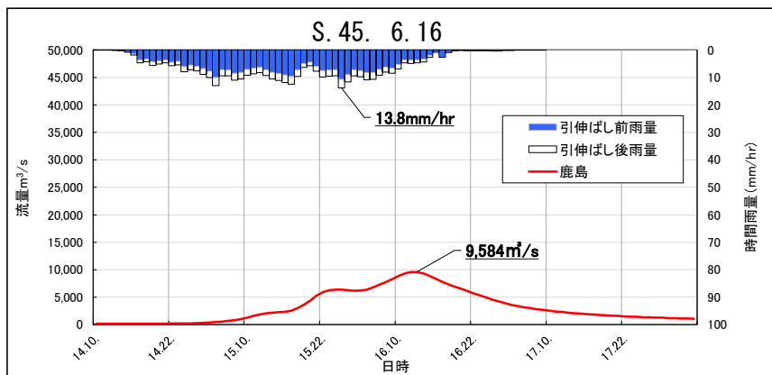
図 1.18 (19) 基本高水ハイドログラフ(昭和 45 年 6 月洪水 鹿島)
