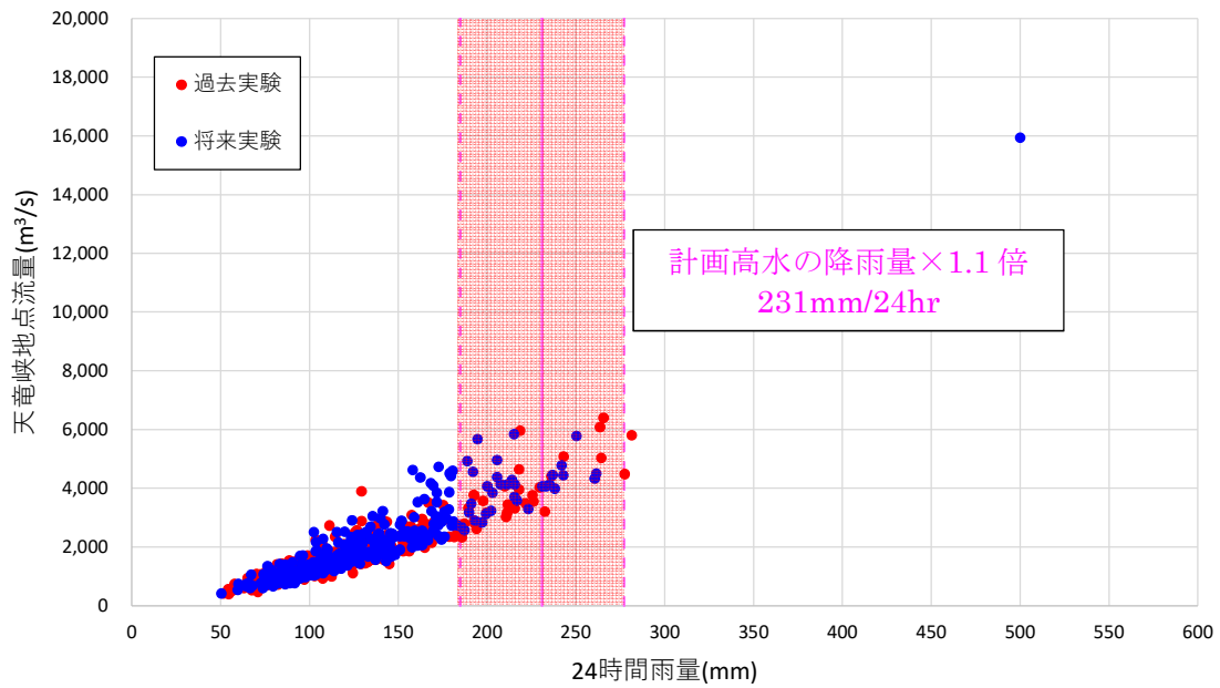
図 1.19 (1) アンサンブル予測降雨からの抽出(基準地点天竜峡)
