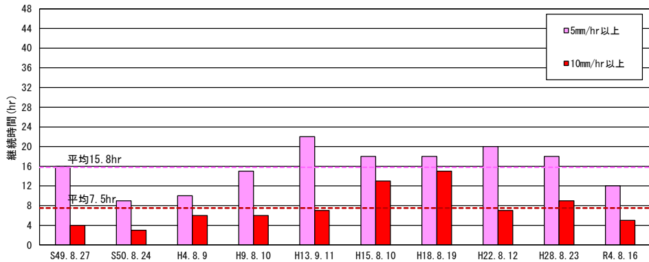
主要洪水における強度の強い降雨時間（平取基準）
