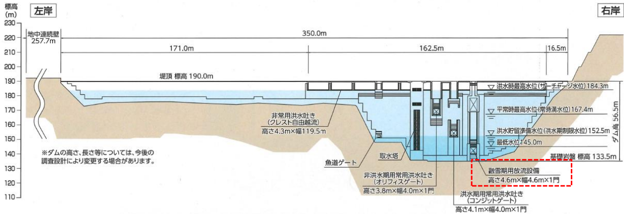
平取ダムの上流から見た概略図
