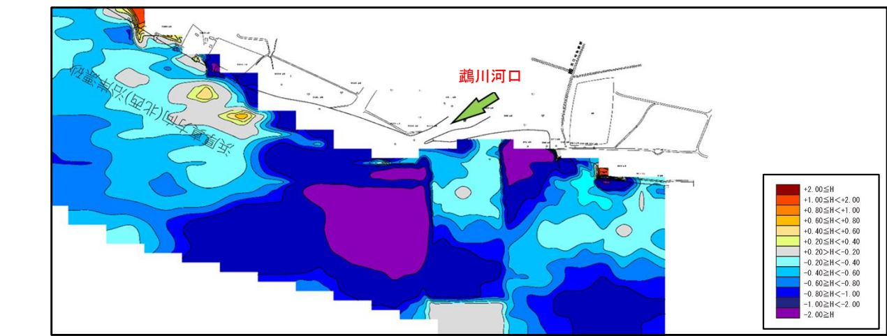
◀海底の高さの変化（平成16年→令和3年）▶
