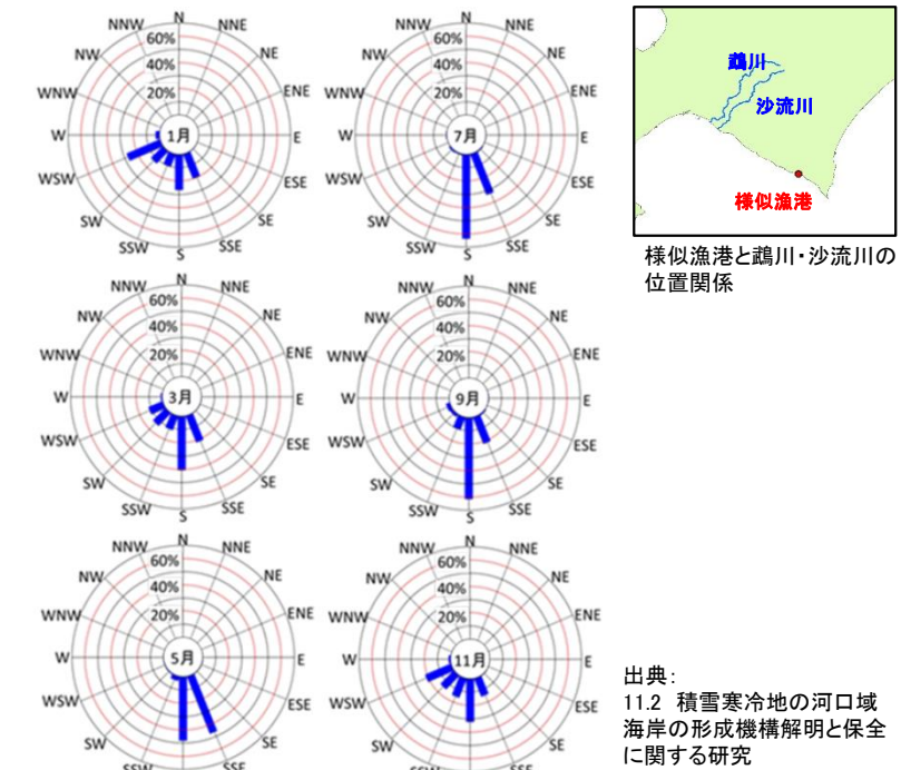
◀様似漁港沖における波向別の波浪エネルギーフラックスの割合▶
