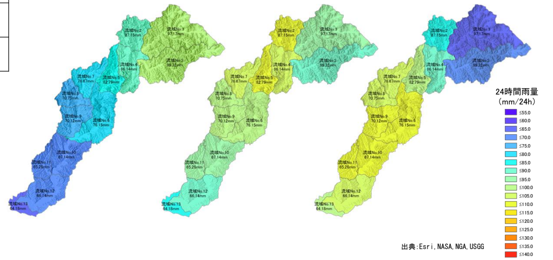
鵜川のアンサンブル予測雨量による降雨分布のクラスター分析結果
