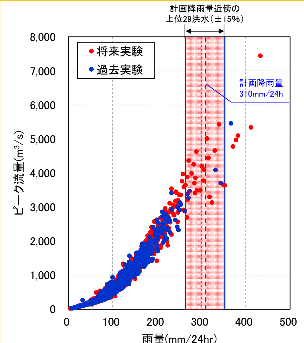
アンサンブル将来予測降雨波形データを用いた検討（鵜川地点）
