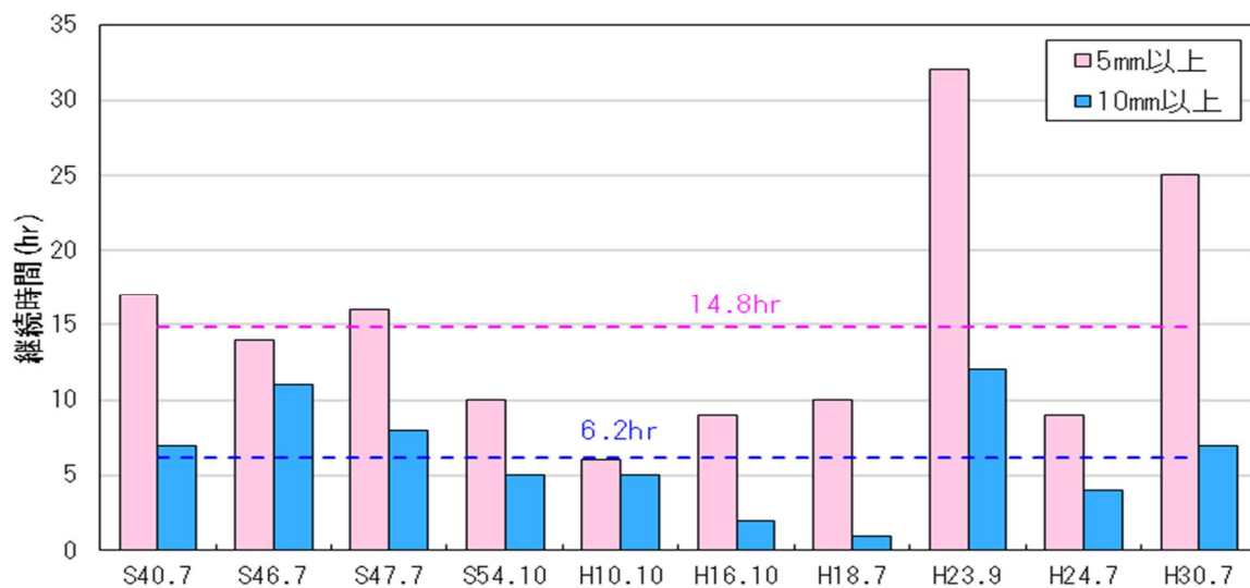
図 1-10 強い降雨強度の継続時間（旭川流域平均雨量）
