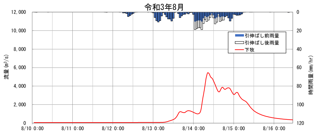
図 1-14 (6) 基本高水ハイドログラフ (基準地点下牧)
