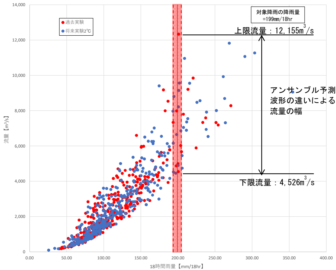
図 1-15(1) アンサンブル予測降雨波形からの抽出（基準地点下牧）
