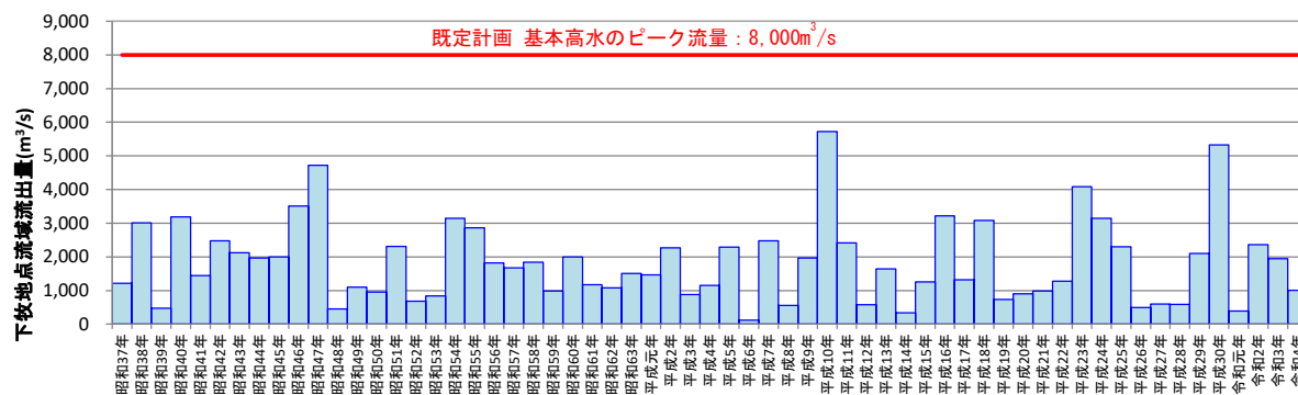
図 1-2 年最大流量（基準地点下牧）
