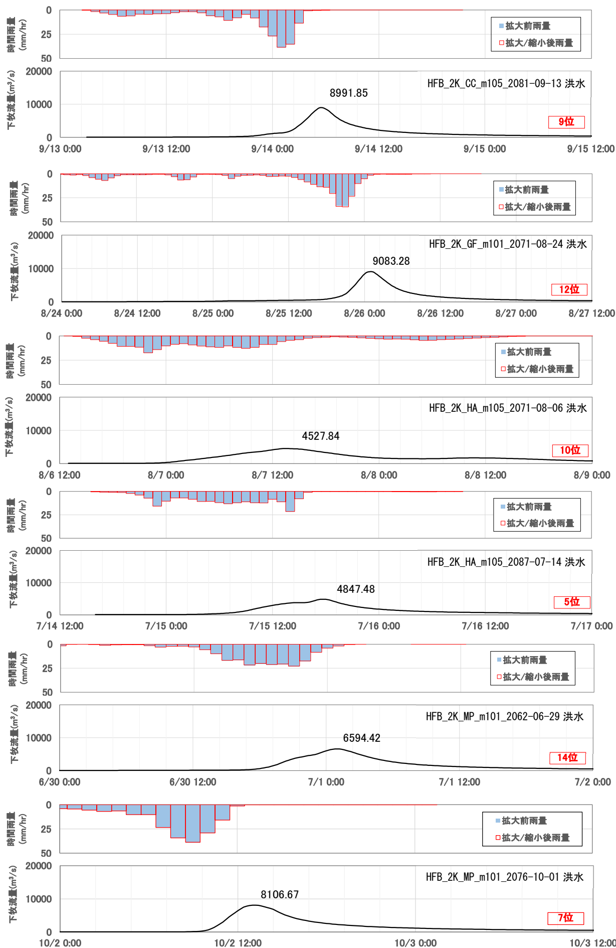
図 1-16(1) 抽出した予測降雨波形のハイドログラフ (基準地点下牧)
