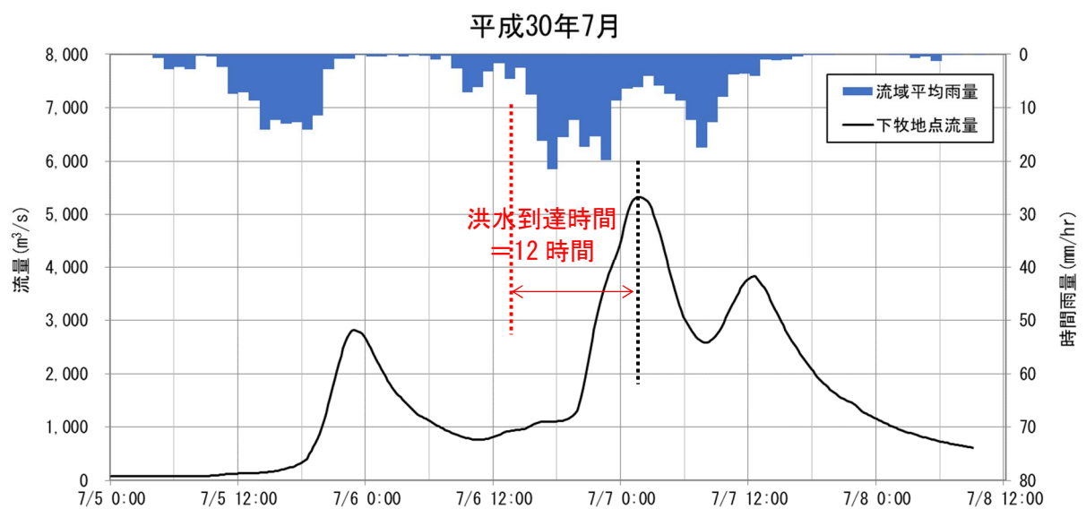
図 1-7(3) Kinematic Wave 法による洪水到達時間
