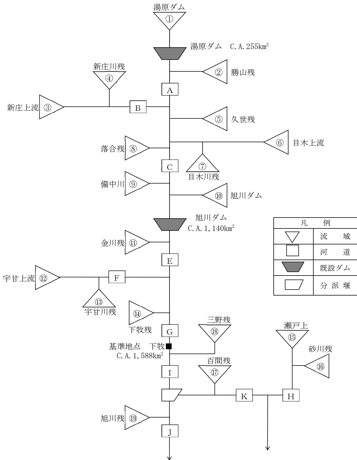
図 1-4 流出モデル模式図
