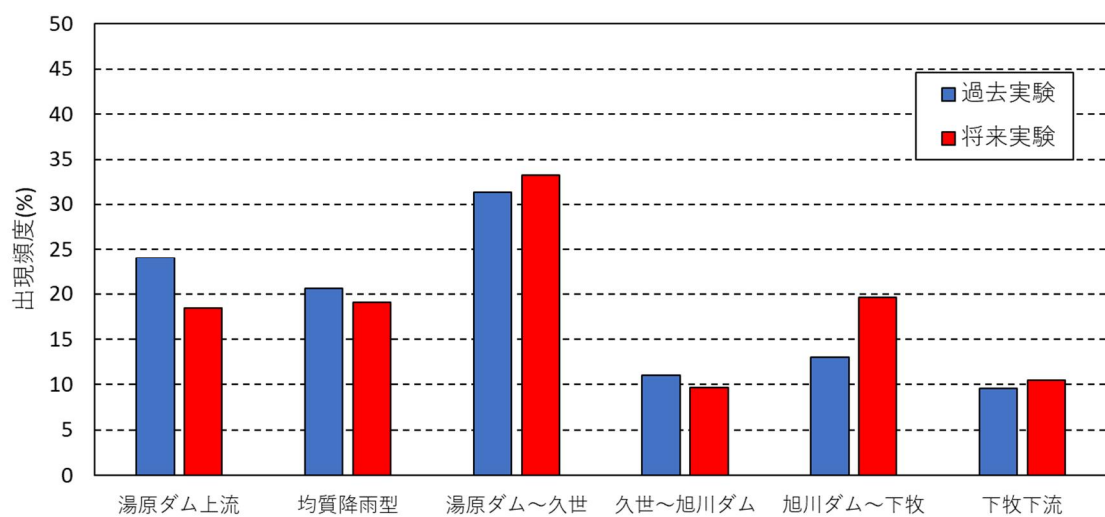
図 1-18 旭川流域のアンサンブル予測降雨の出現頻度（クラスター毎）
