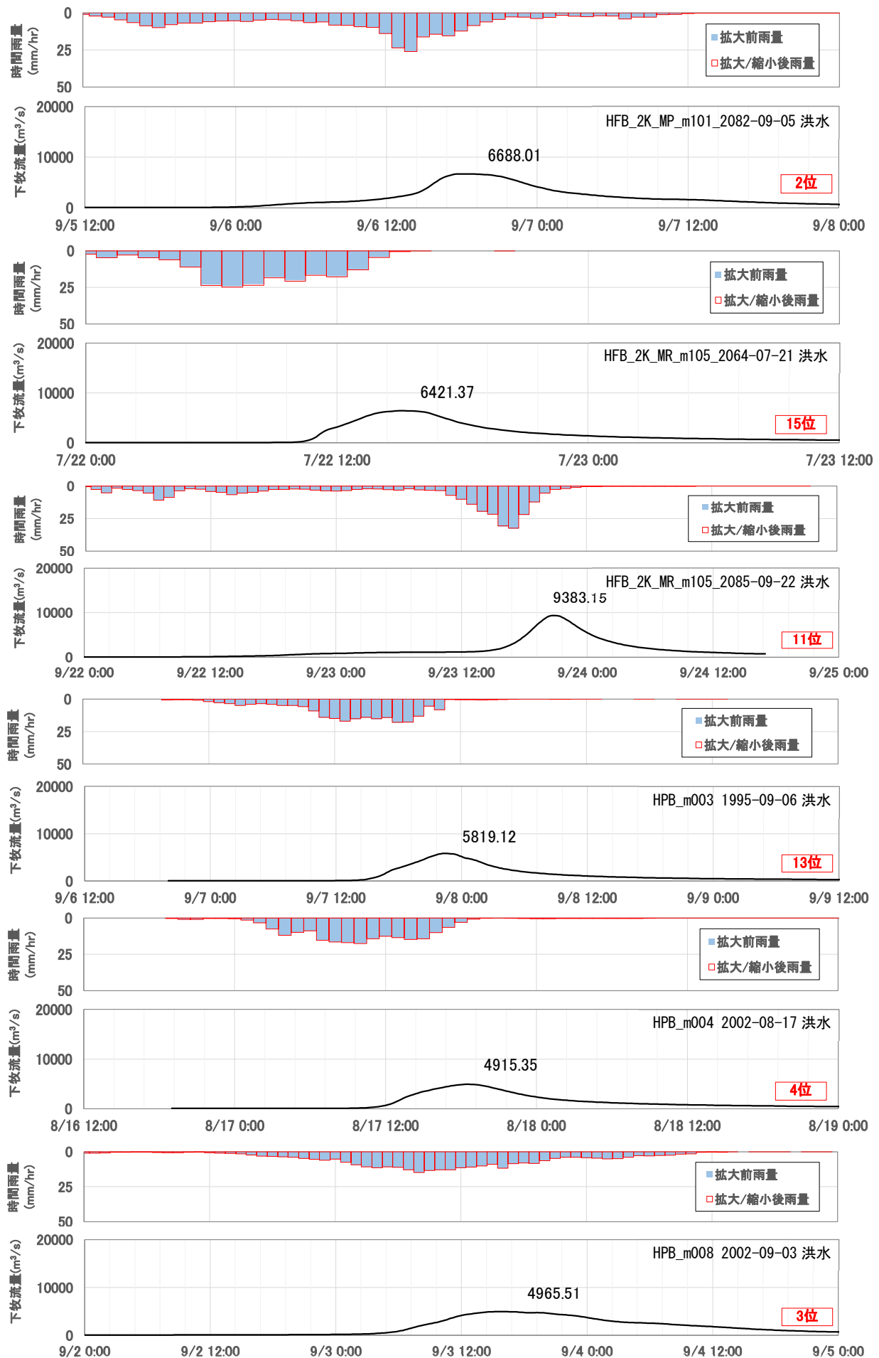
図 1-16(2) 抽出した予測降雨波形のハイドログラフ (基準地点下牧)
