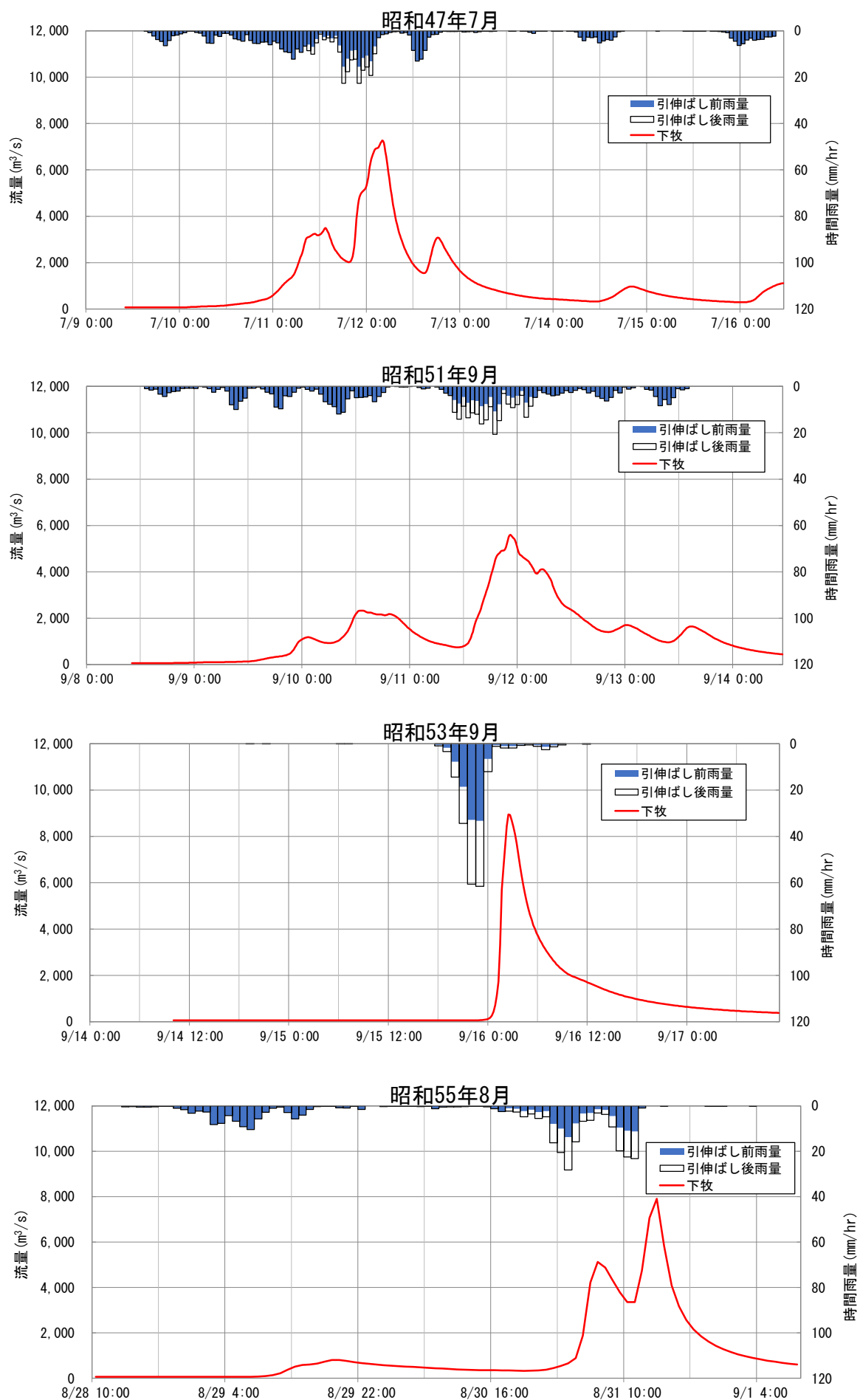
図 1-14 (3) 基本高水ハイドログラフ (基準地点下牧)
