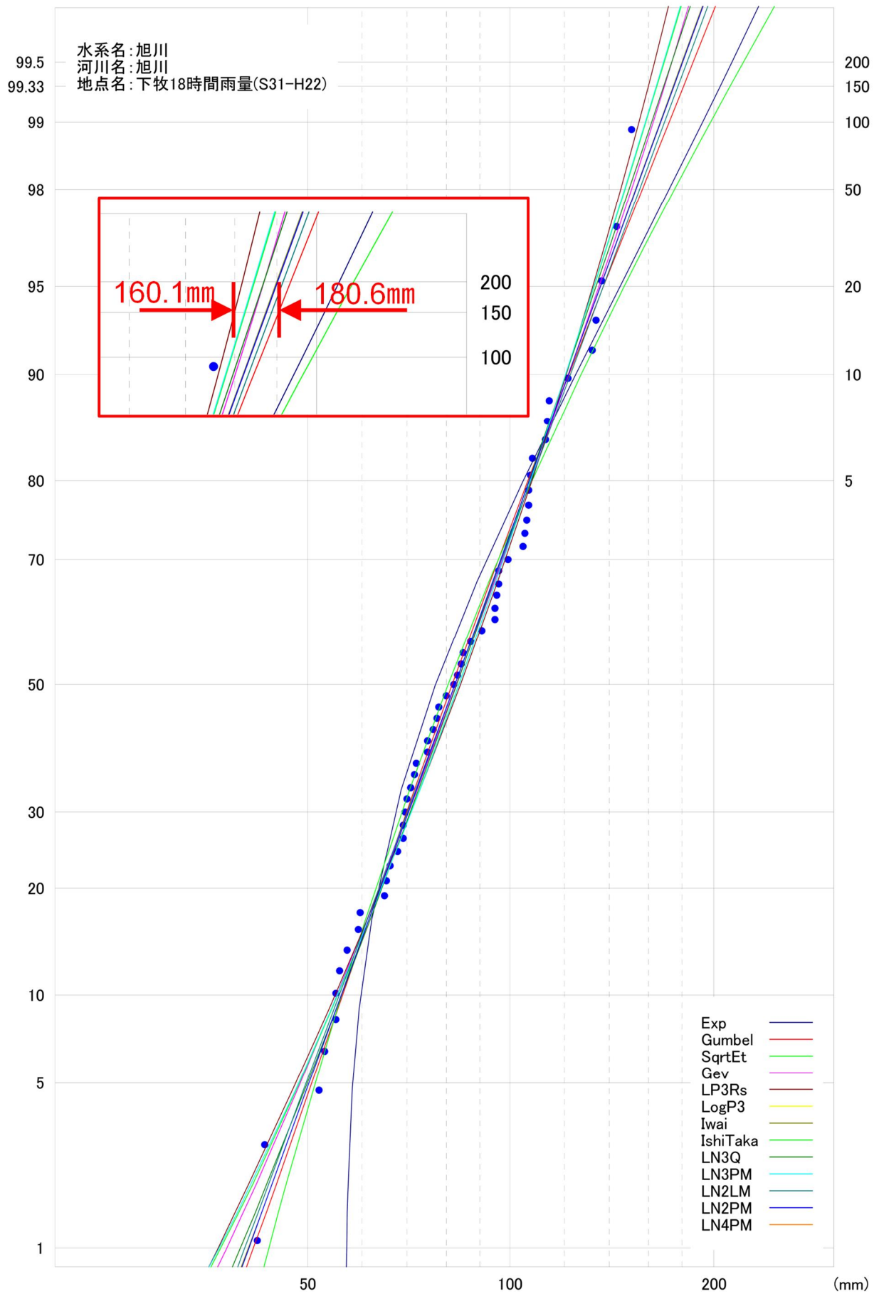
図 1-11 雨量確率計算結果
