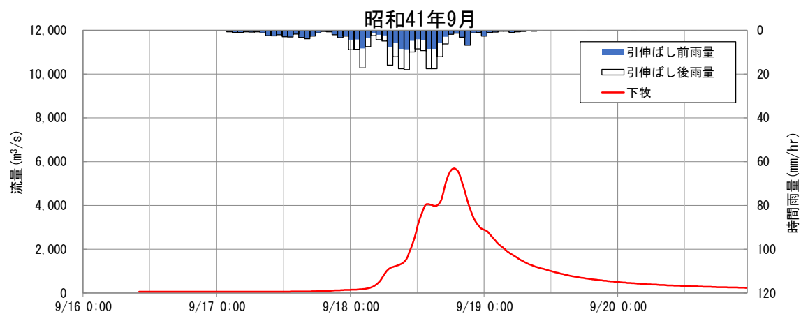
図 1-14(1) 基本高水ハイドログラフ (基準地点下牧)
