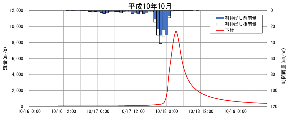
図 1-14 (4) 基本高水ハイドログラフ (基準地点下牧)
