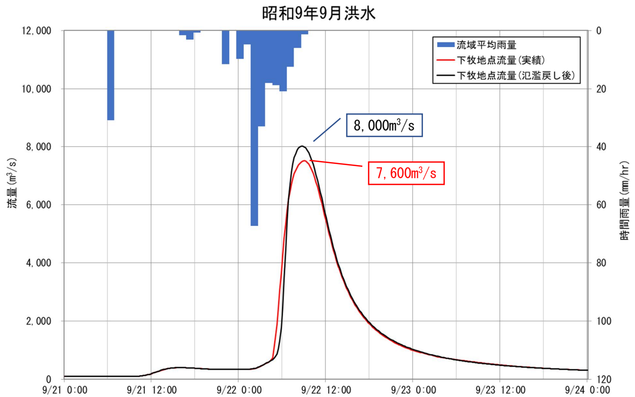
図 1-19 昭和9年（1934年）9月洪水の推定結果（基準地点下牧）
