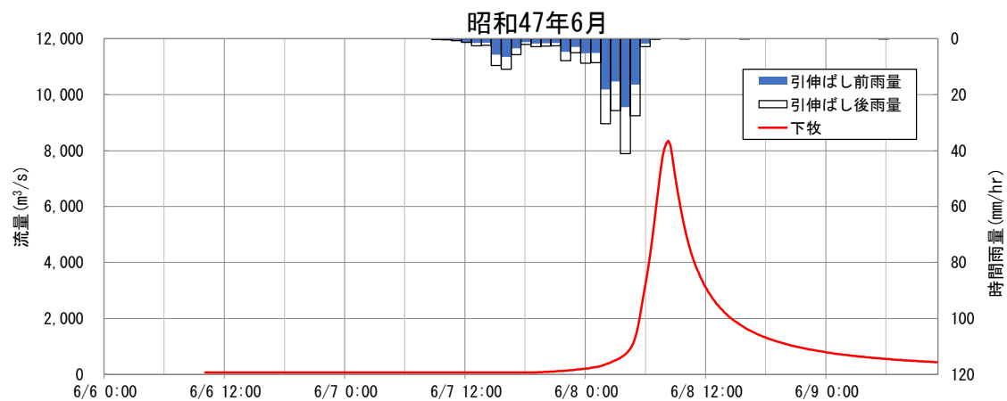
図 1-14 (2) 基本高水ハイドログラフ (基準地点下牧)
