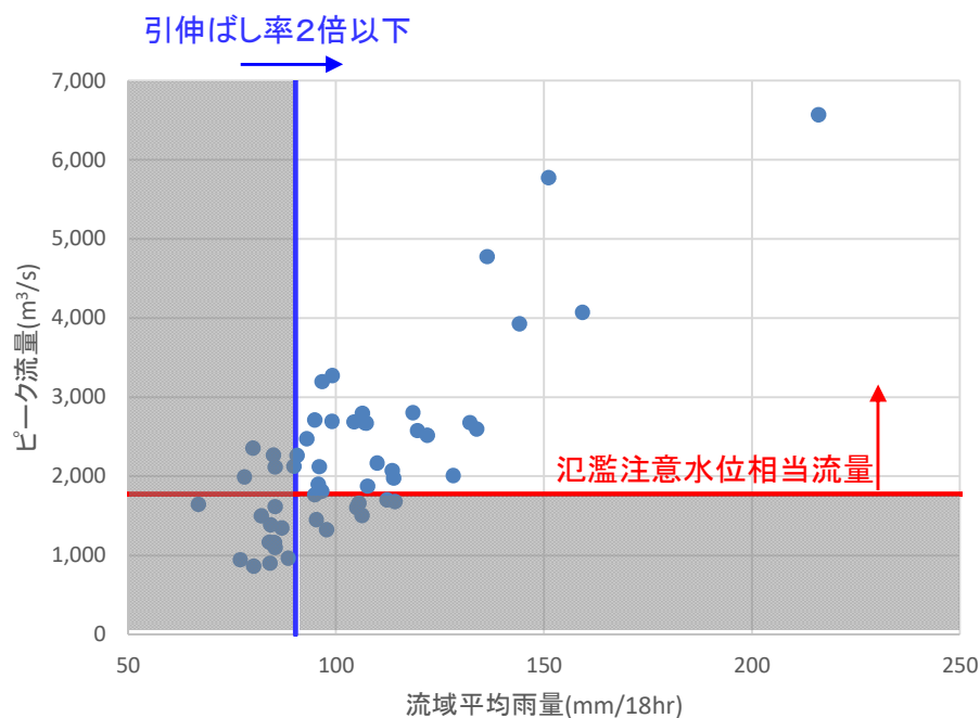
図 1-12 対象洪水の選定（基準地点下牧）
