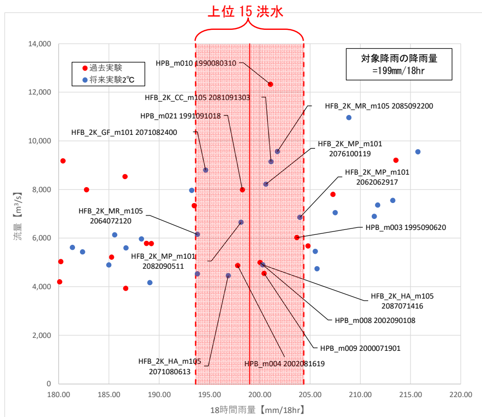
図 1-15(2) アンサンブル予測降雨波形からの抽出（基準地点下牧）【詳細図】
