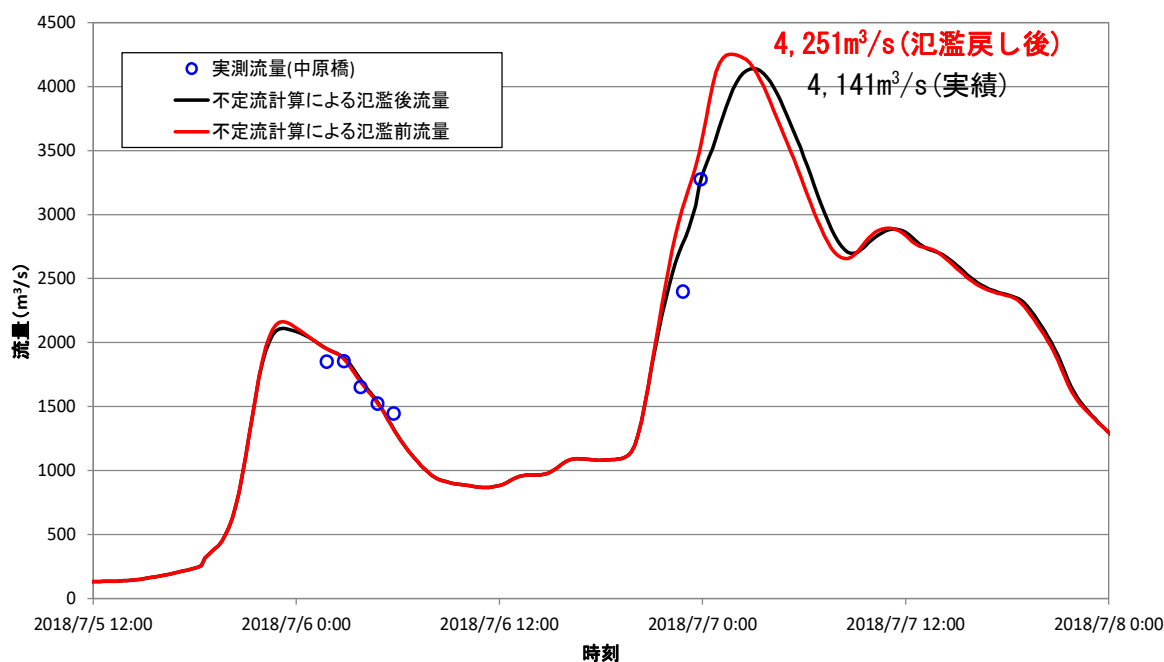
図 1-5 平成 30 年（2018 年）7 月豪雨における不定流計算検証図
