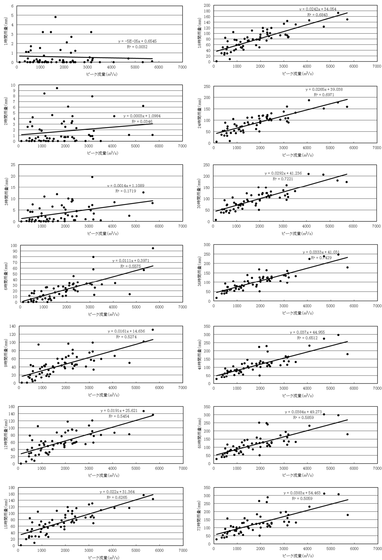
図 1-9 (2) ピーク流量と流域平均時間雨量の相関図【定義②】
