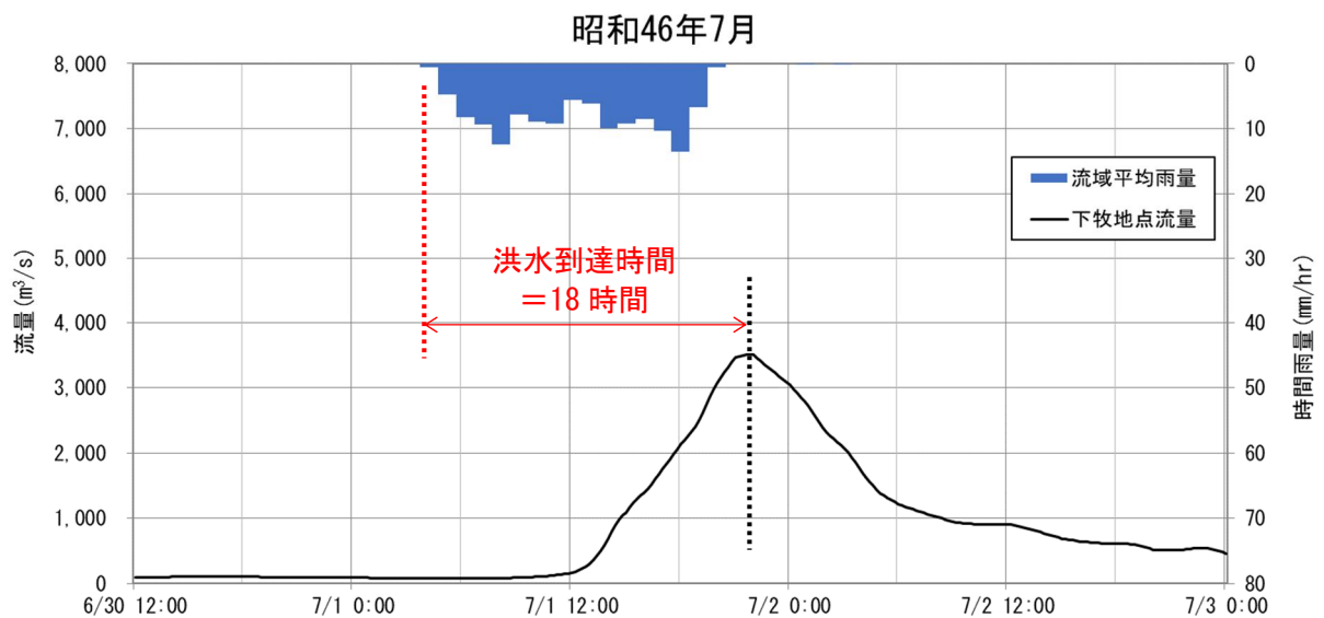
図 1-7(1) Kinematic Wave 法による洪水到達時間
