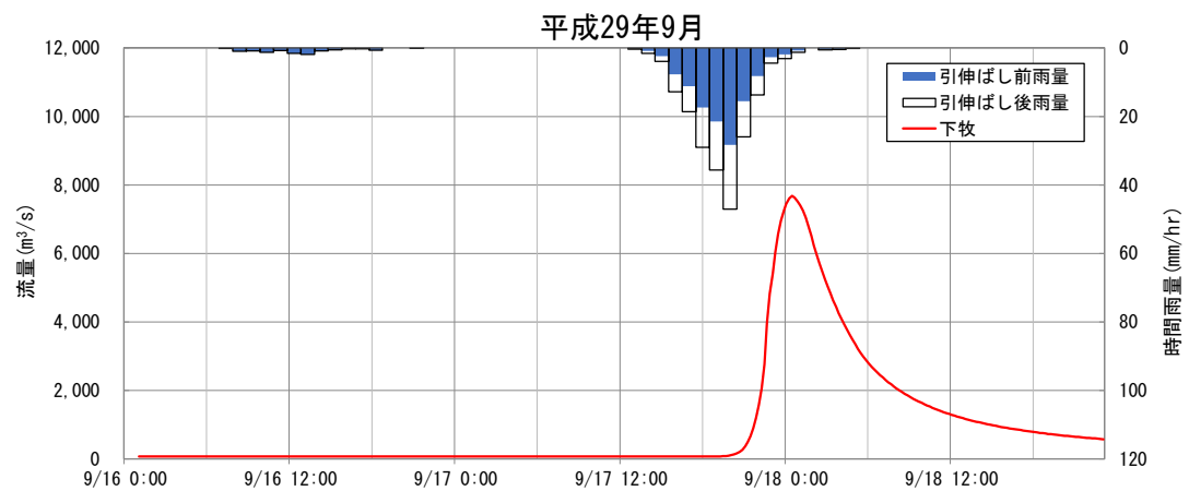
図 1-14 (5) 基本高水ハイドログラフ (基準地点下牧)
