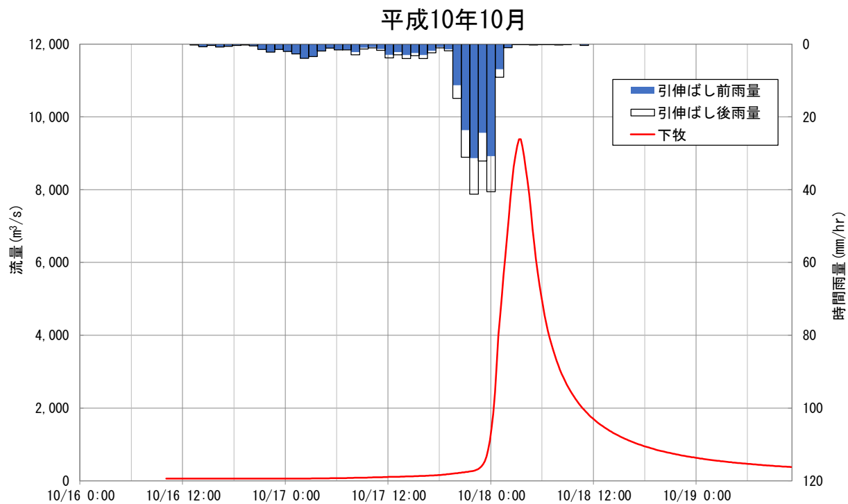
図 1-21 基本高水のピーク流量ハイドログラフ（平成 10 年（1998 年）10 月洪水）
