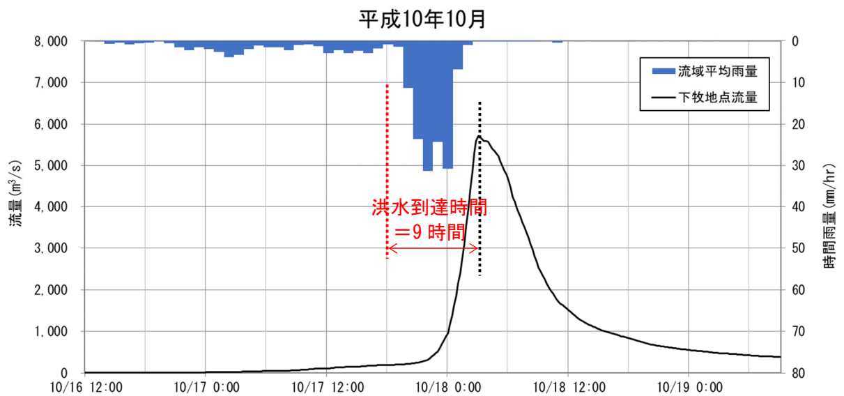
図 1-7(2) Kinematic Wave 法による洪水到達時間
