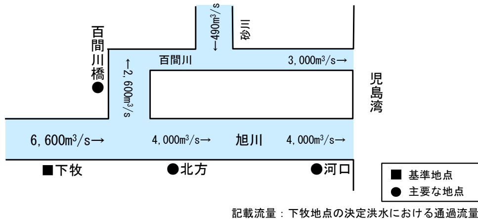
図 3-1 旭川計画高水流量図
