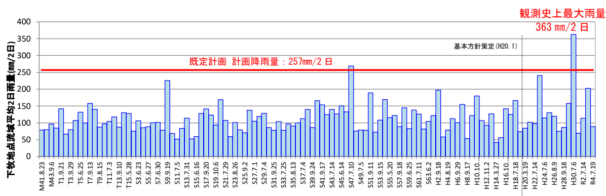
図 1-1 年最大流域平均雨量（基準地点下牧上流域平均雨量）
