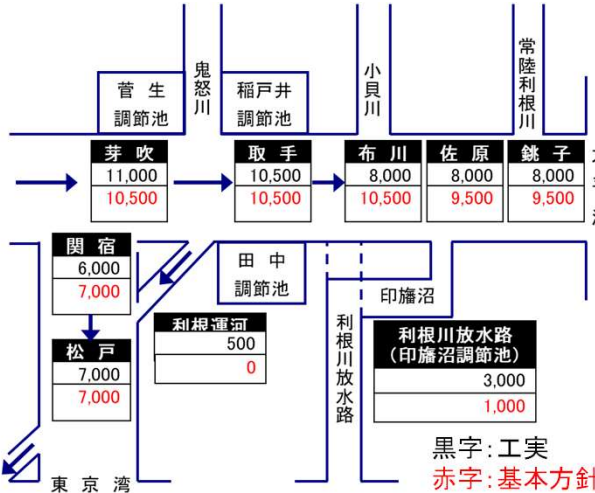
■令和元年東日本台風時の下流三調節池の洪水調節状況 (貯水率 田中:約70%、稲戸井:約95%、菅生:100%超)
