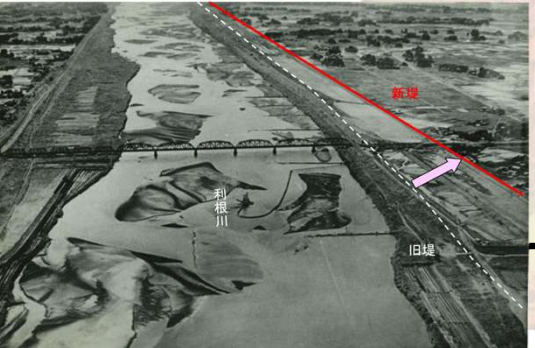
利根川・江戸川における引堤の整備 (現: 加須市)
