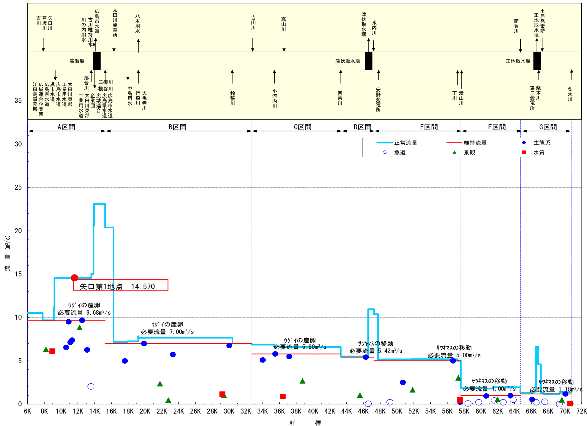
図 6-2 (2) 太田川 水収支縦断図 ウグイ産卵期 (2 月 1 日～4 月 30 日)
