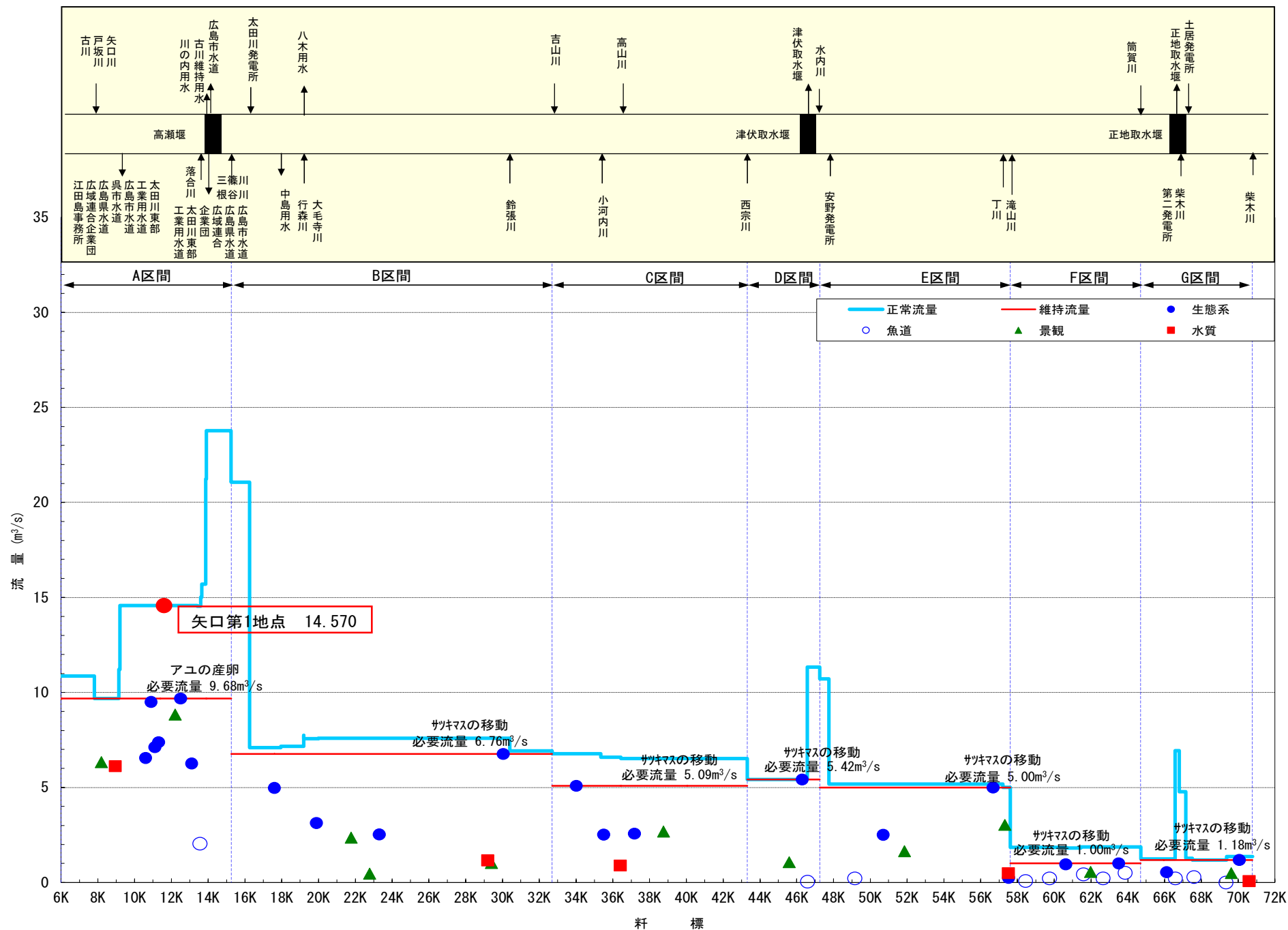
図 6-2 (7) 太田川 水収支縦断面図 アユ産卵期 (10 月 21 日 ~ 12 月 31 日)
