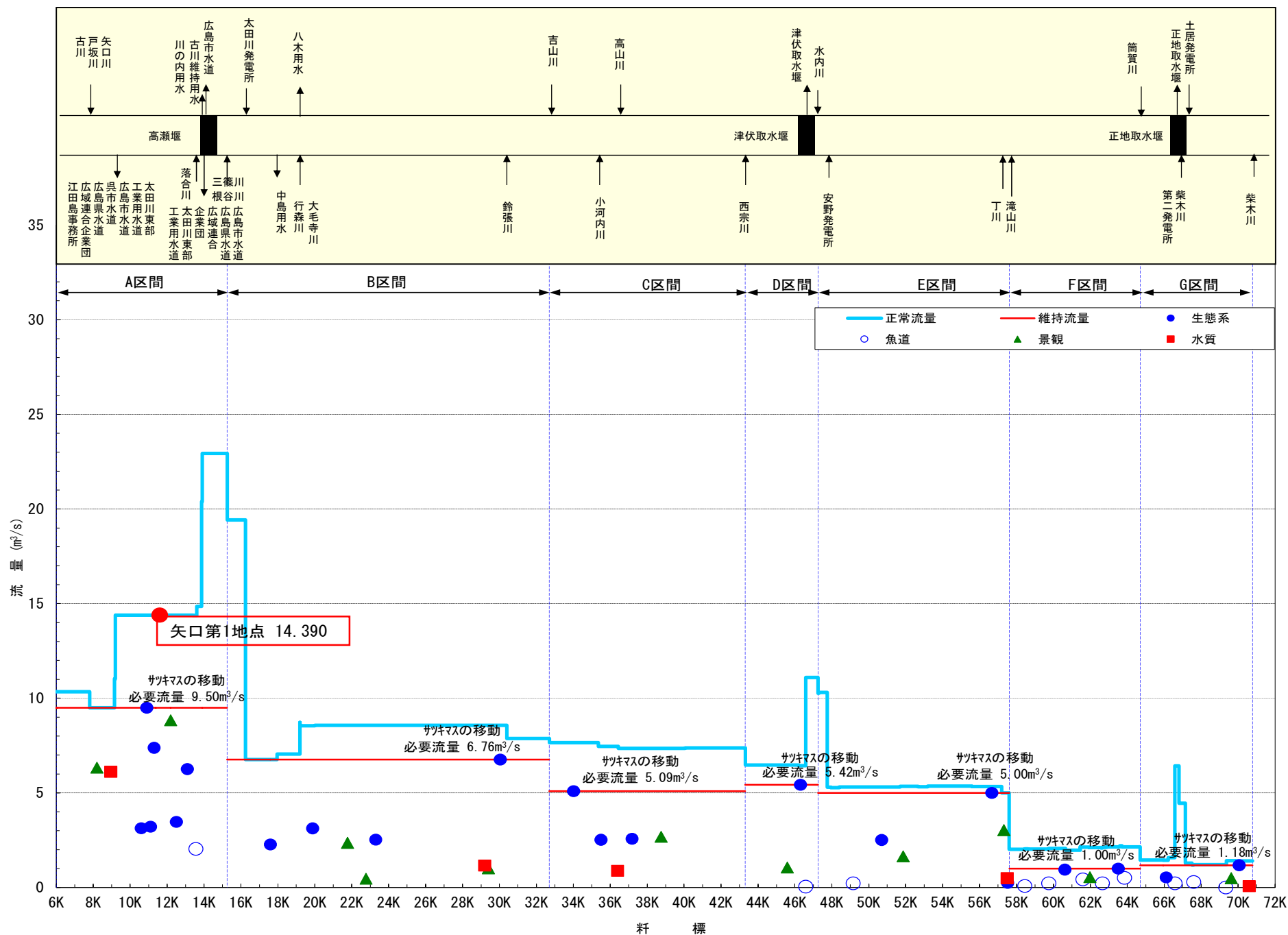
図 6-2 (3) 太田川 水収支縦断図 かんがい前期 (5 月 1 日~6 月 14 日)
