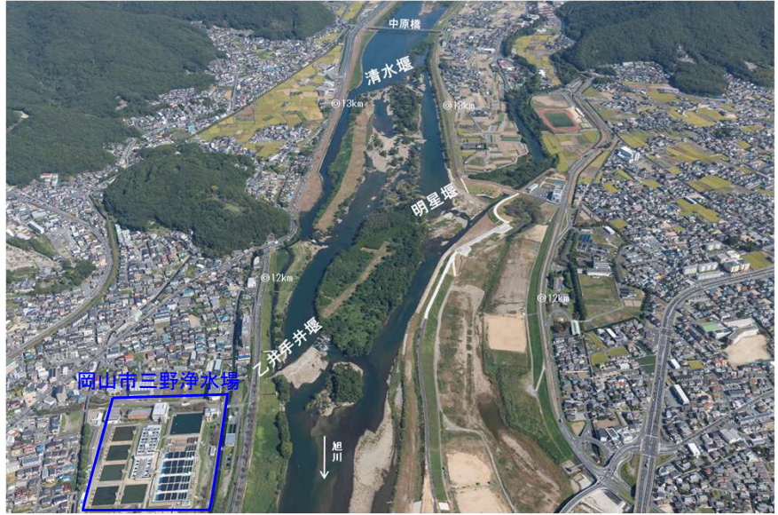
分流部付近の固定堰
