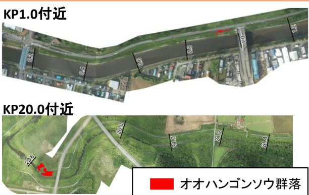
オオハンゴンソウ群落の分布状況
