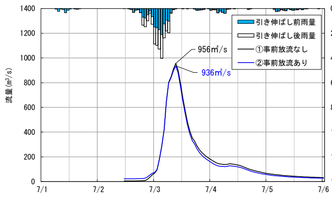
【平成30年7月3日型洪水】
