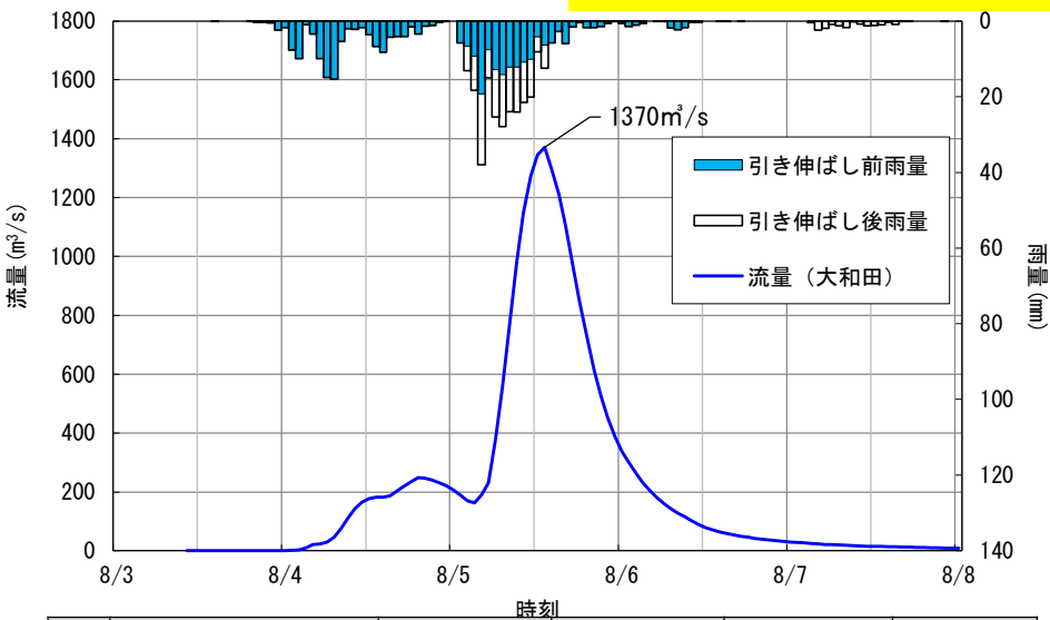
大和田地点 昭和56年8月波形
