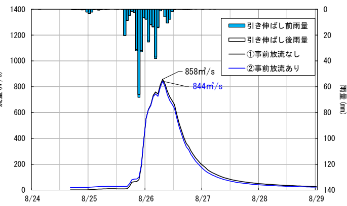
【昭和63年8月26日型洪水】
