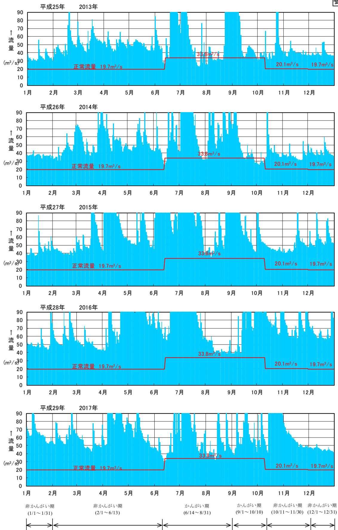
図 6 - 2 ( 1 ) 日平均流量図 荒瀬地点 (荒瀬水位・流量観測所 : 2013 年～2019 年)
