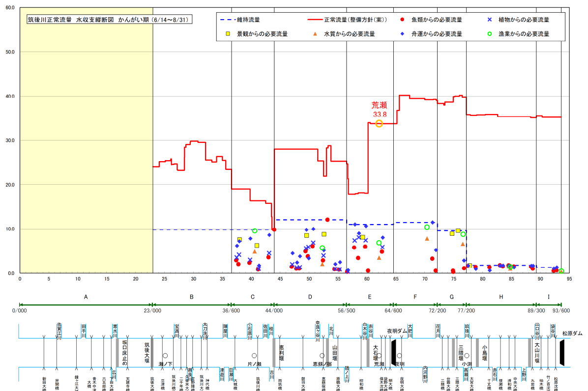
図 6-1 (1) 筑後川正常流量水収支縦断図【かんがい期：6/14~8/31】
