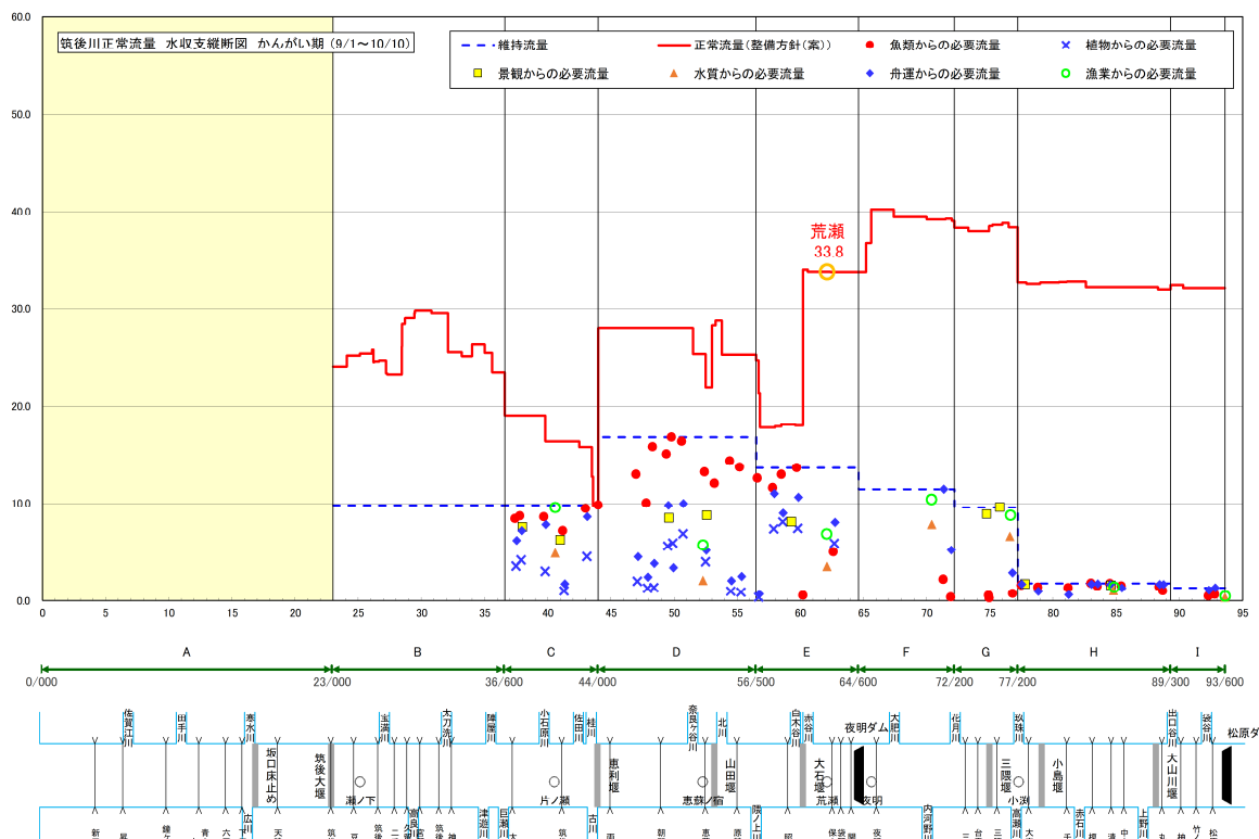
図 6-1 (2) 筑後川正常流量水収支縦断図【かんがい期：9/1~10/10】
