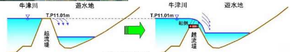
遊水地の事例 (六角川支川・牛津川)
