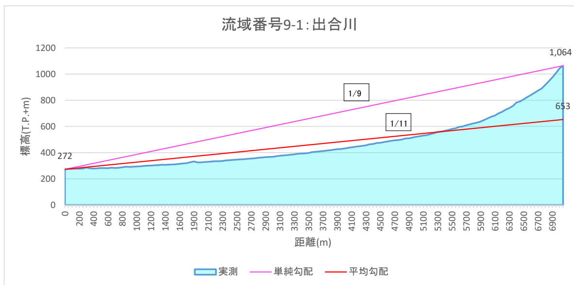
図 1-13 (16) 流域平均勾配の設定結果 (流域9-1)
