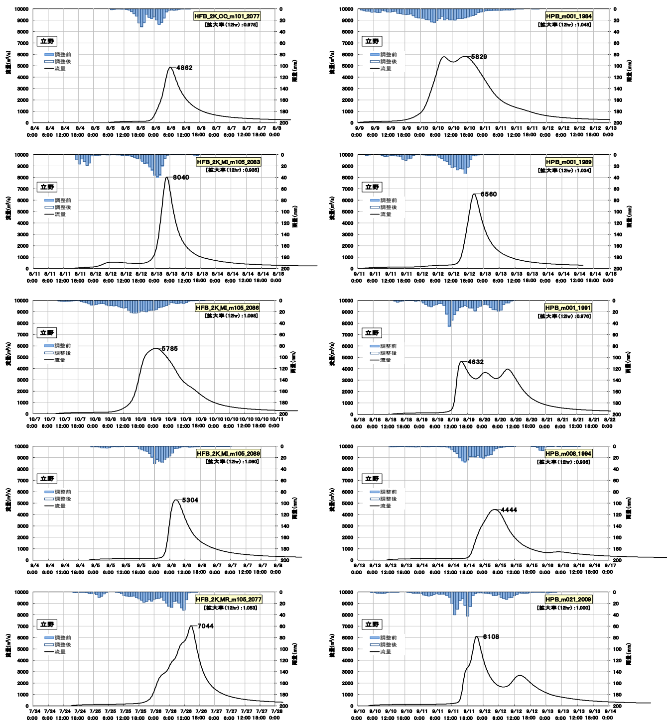
図 1-34 抽出した予測降雨波形群によるハイドログラフ（立野地点、過去実験）
