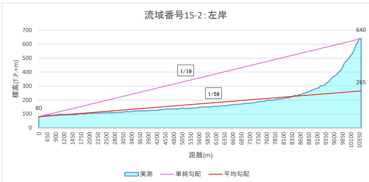
図 1-13 (29) 流域平均勾配の設定結果 (流域15-2)
