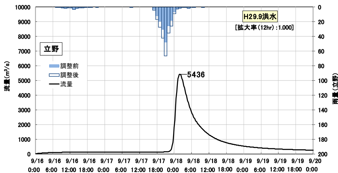
図 1-32 (3) 基本高水ハイドロ (円山川：立野 本川 W=1/100 降雨量変化倍率1.1倍後)
