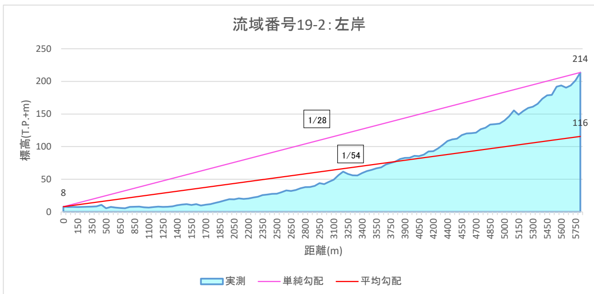
図 1-13 (37) 流域平均勾配の設定結果 (流域19-2)
