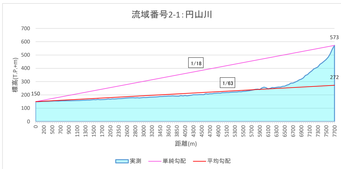
図 1-13 (3) 流域平均勾配の設定結果 (流域2-1)
