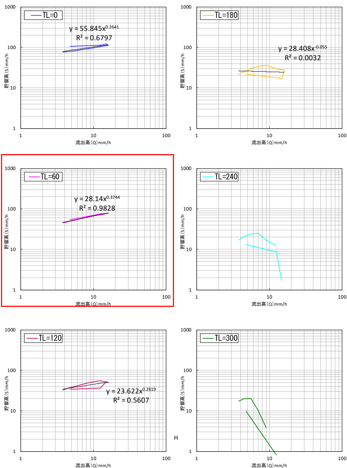
図 1-11 (2) 流出高と貯留高の関係（弘原地点：平成21年8月洪水）
