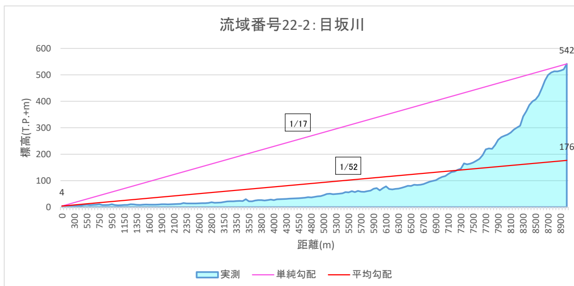
図 1-13 (43) 流域平均勾配の設定結果 (流域22-2)
