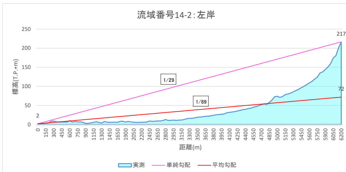
図 1-13 (27) 流域平均勾配の設定結果 (流域14-2)
