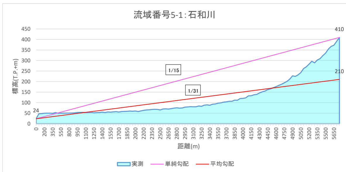
図 1-13 (9) 流域平均勾配の設定結果 (流域5-1)
