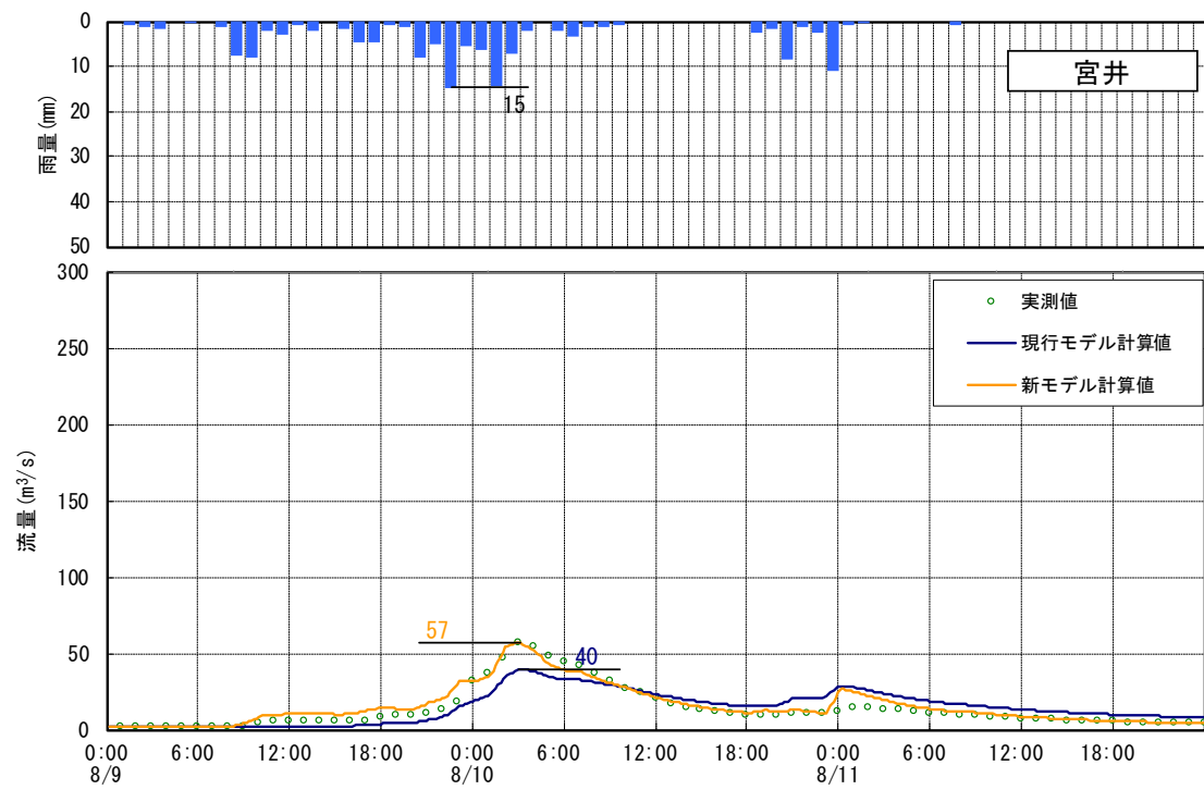
図 1-20 (3) 検証計算結果 (平成21年8月洪水)
