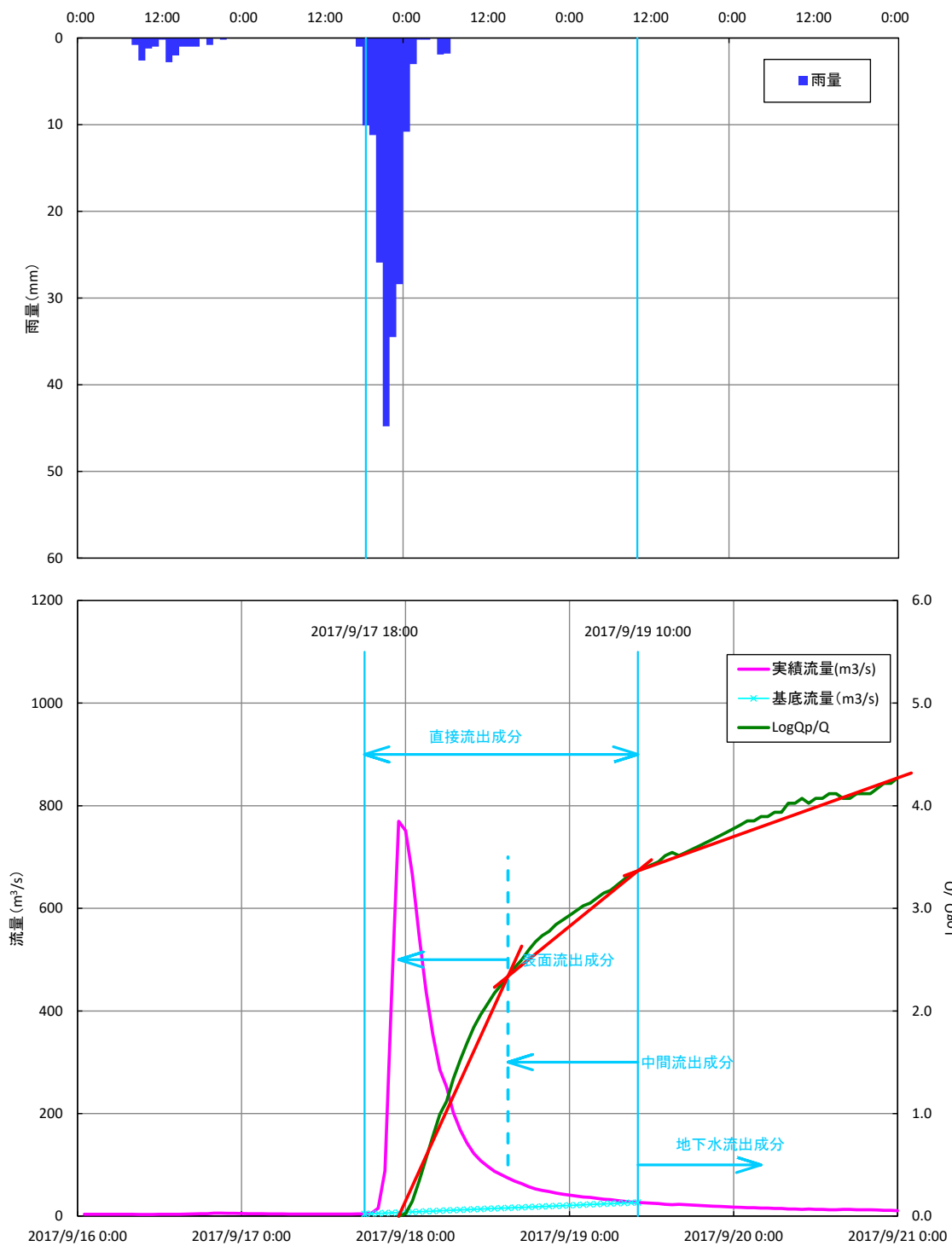
図 1-7 (2) 成分分離結果 (弘原地点 : H29. 9洪水)
