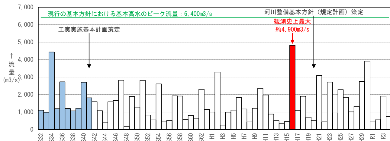
図 1-1 年最大流量（基準地点立野）
