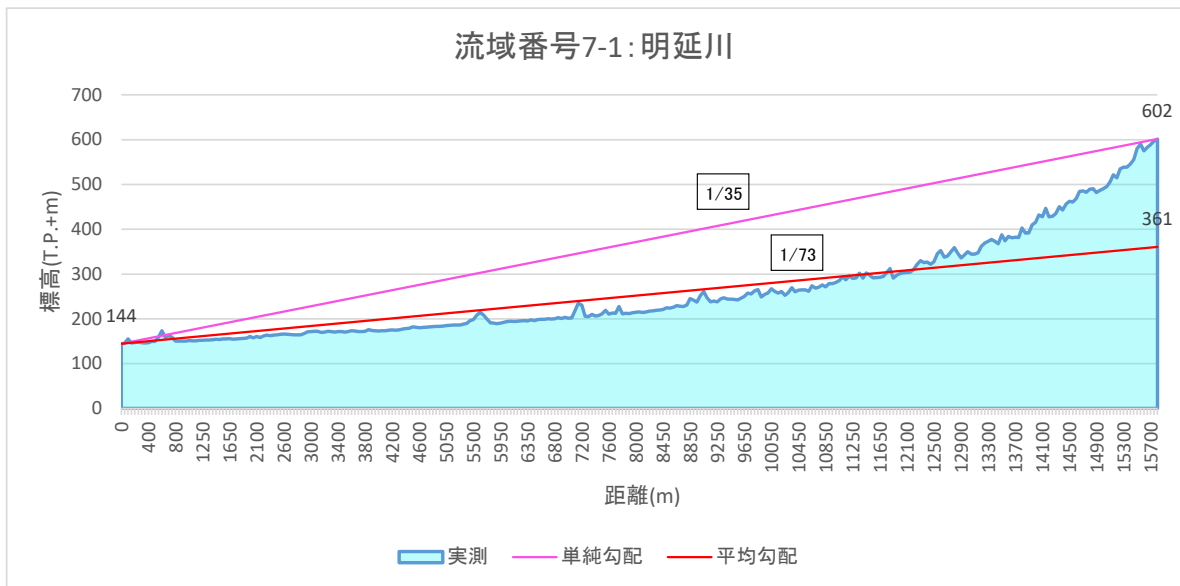
図 1-13 (13) 流域平均勾配の設定結果 (流域7-1)
