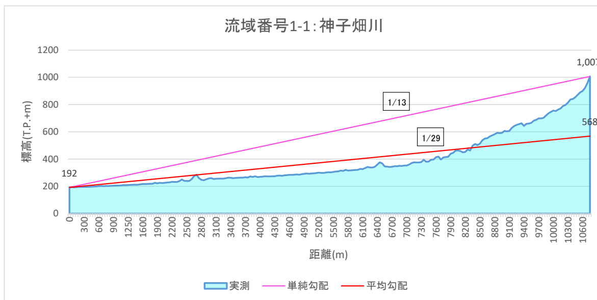
図 1-13 (1) 流域平均勾配の設定結果（流域1-1）
