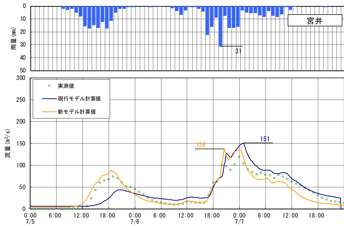
図 1-23 (3) 検証計算結果 (平成30年7月洪水)
