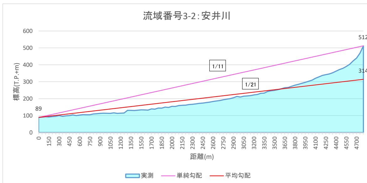
図 1-13 (6) 流域平均勾配の設定結果 (流域3-2)
