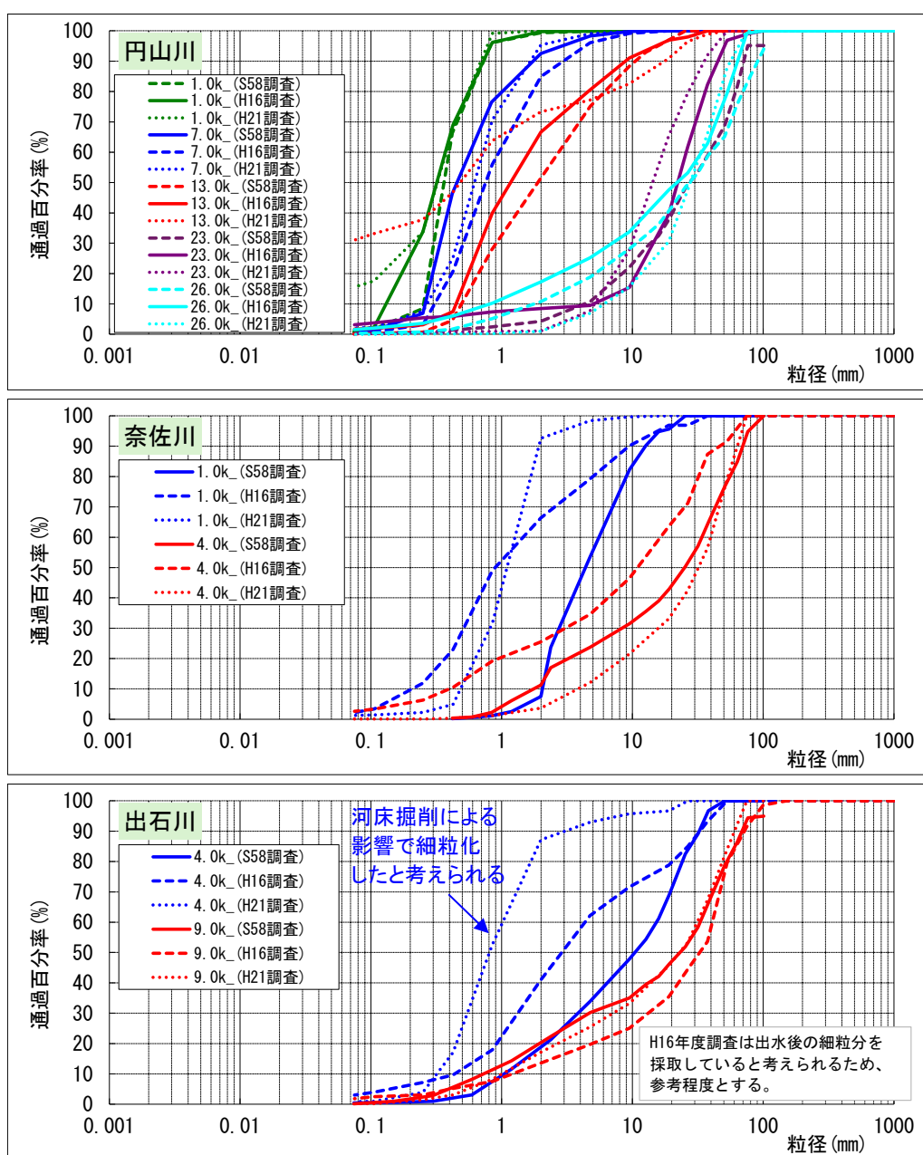
図 4-4 粒径加積曲線の経年変化
