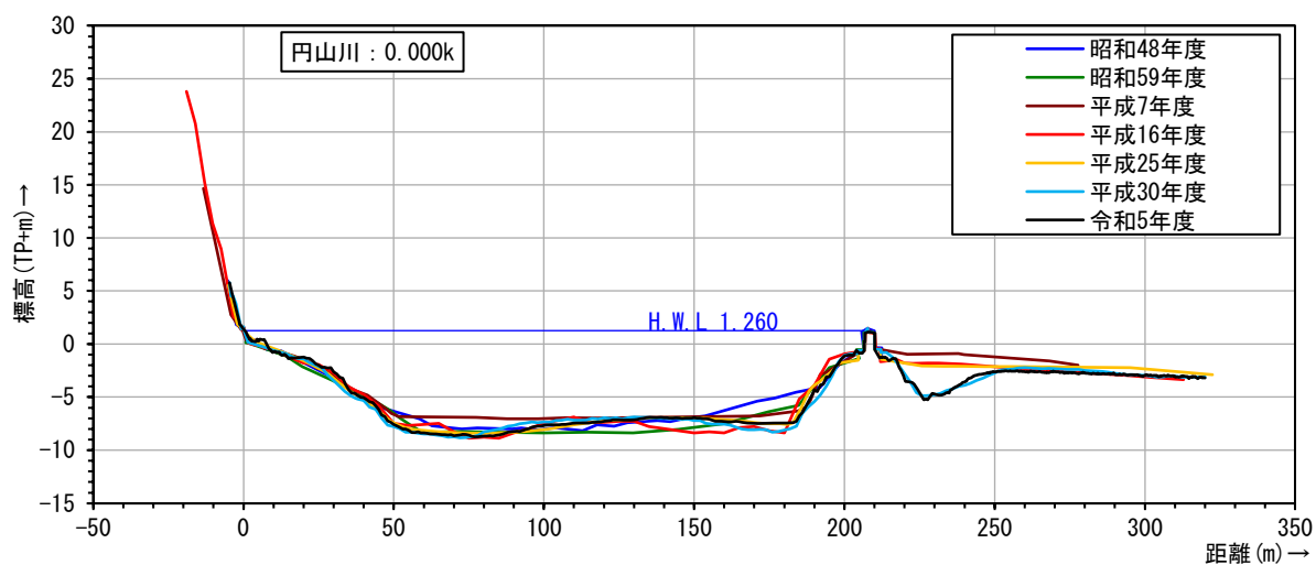
図 5-2 円山川河口部 (0.0k) の横断図
