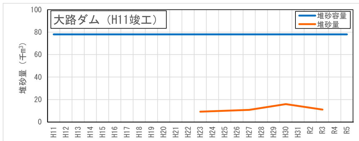
図3-2 (1) 大路ダムの堆砂状況
