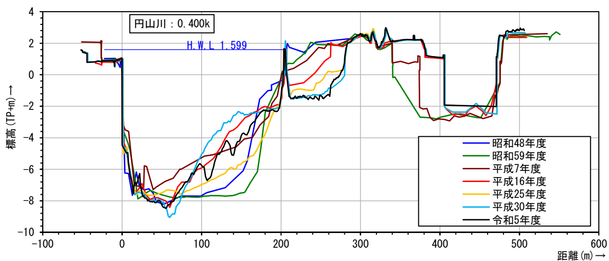
図 5-3 津居山港付近 (0.4k) の横断図
