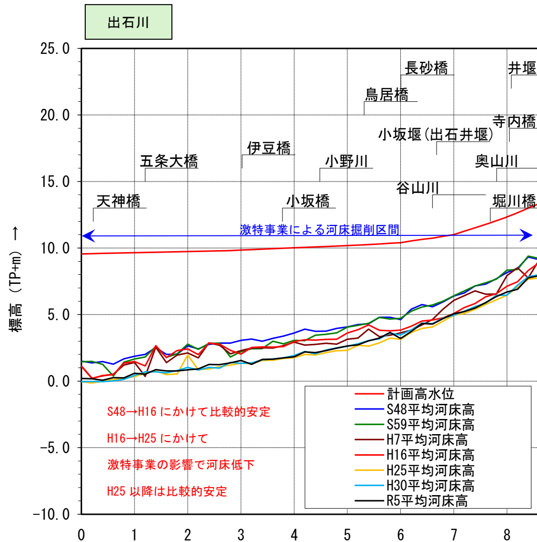
図 4-1 (2) 平均河床高縦断図 (奈佐川・出石川)
