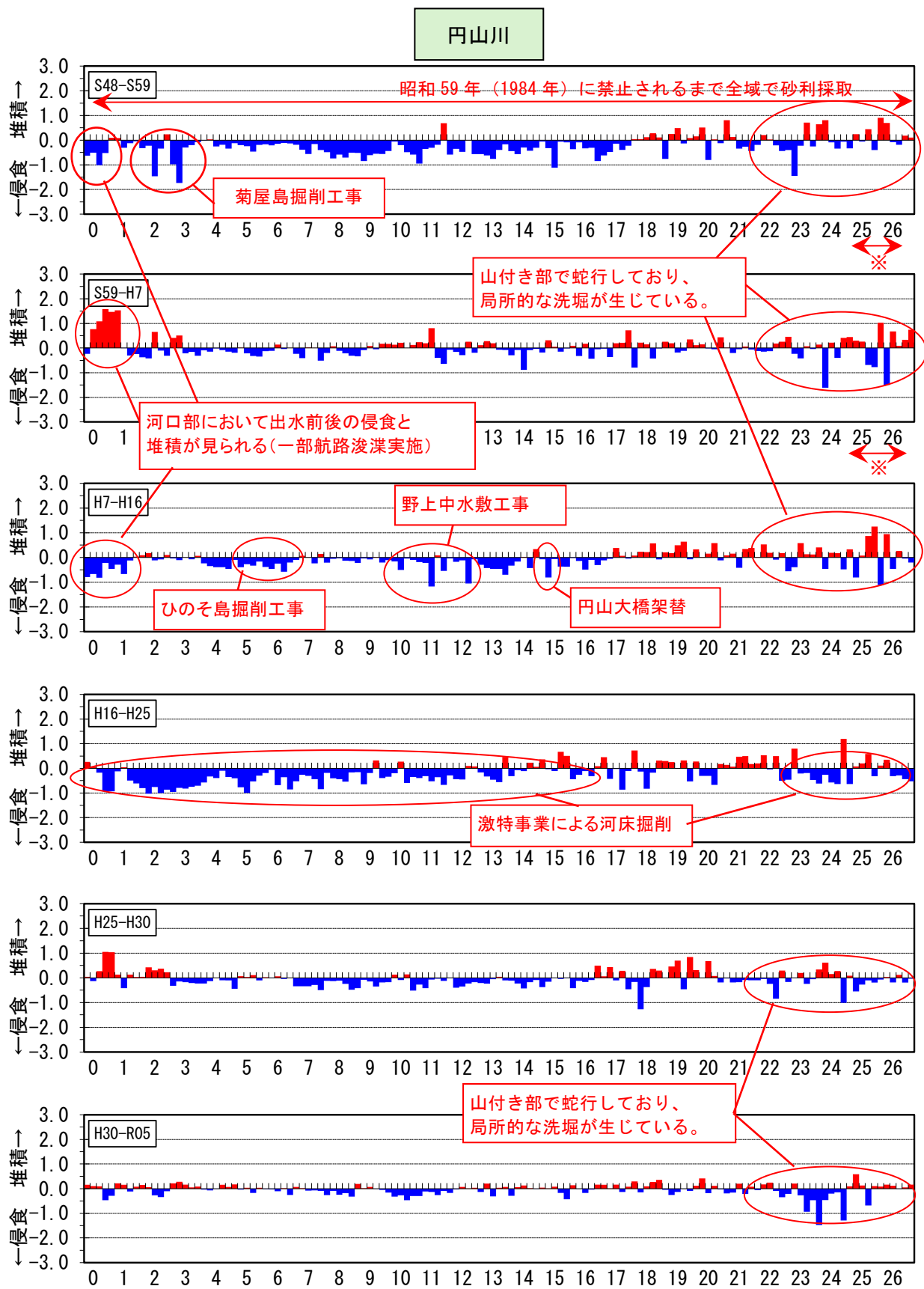
図 4-2 (1) 平均河床高変化量の経年変化図(円山川)
