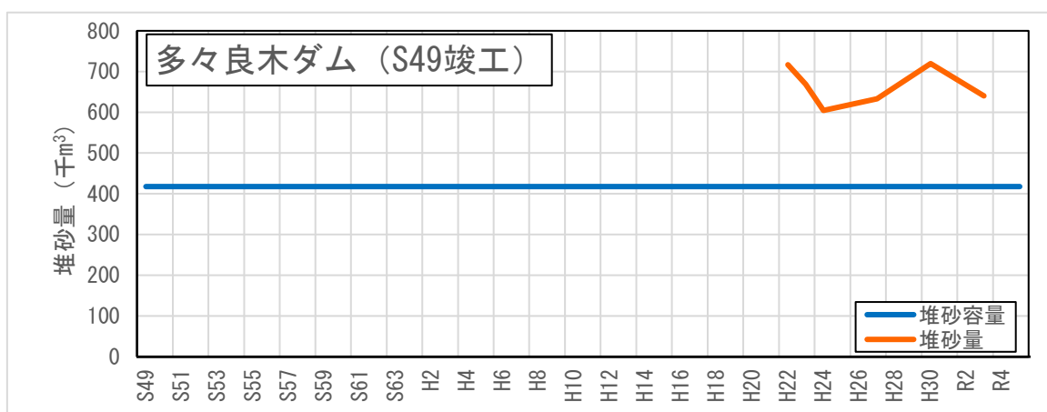
図 3-2 (5) 多々良木ダムの堆砂状況
