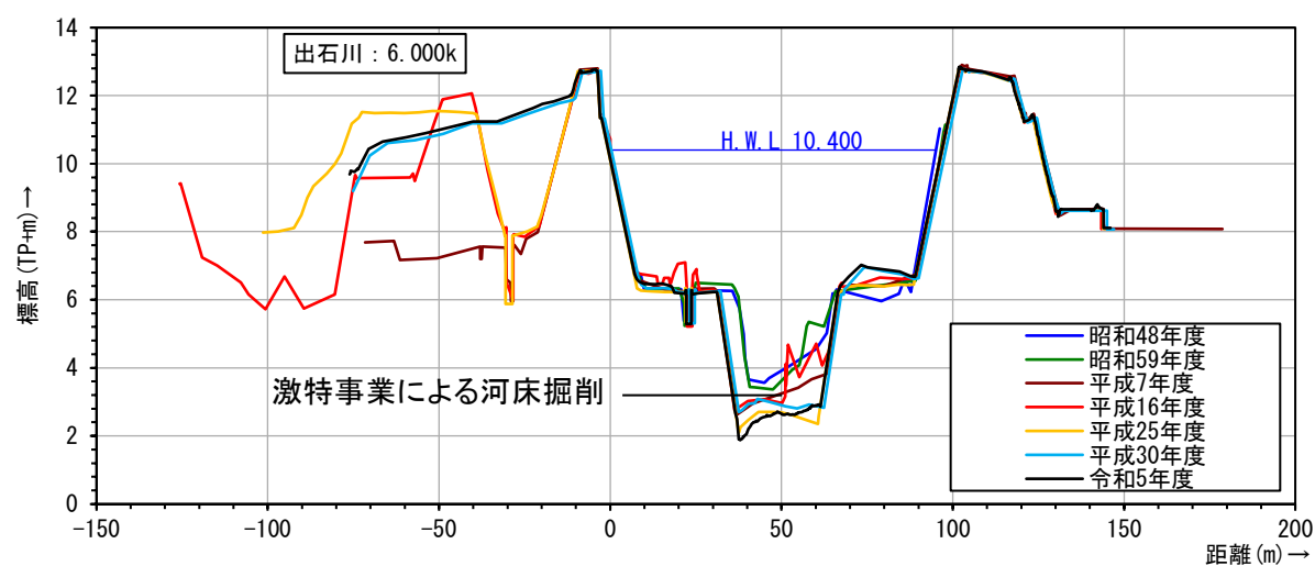
図4-3 (4) 代表横断面図 (出石川6k000)
