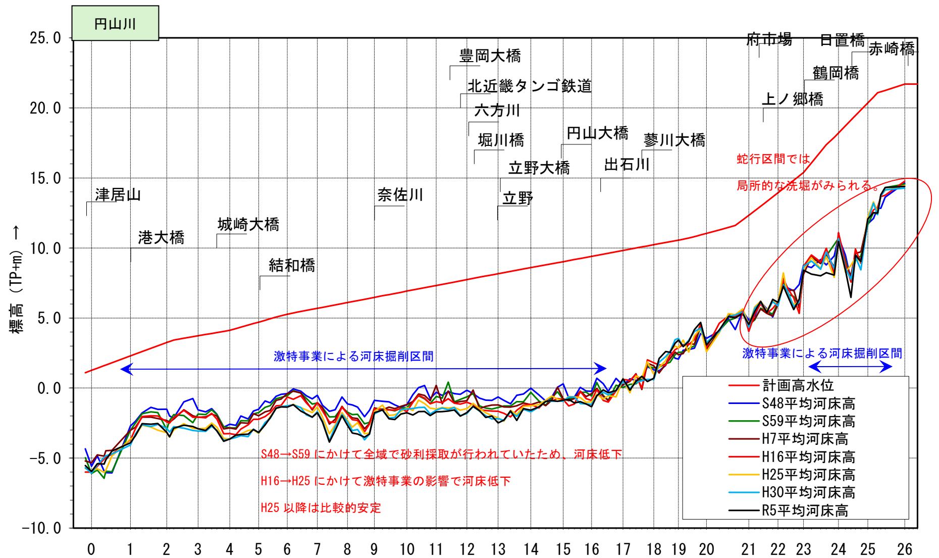
図 4-1 (1) 平均河床高縦断図 (円山川)
