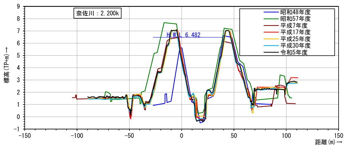
図4-3 (3) 代表横断面図 (奈佐川2k200)
