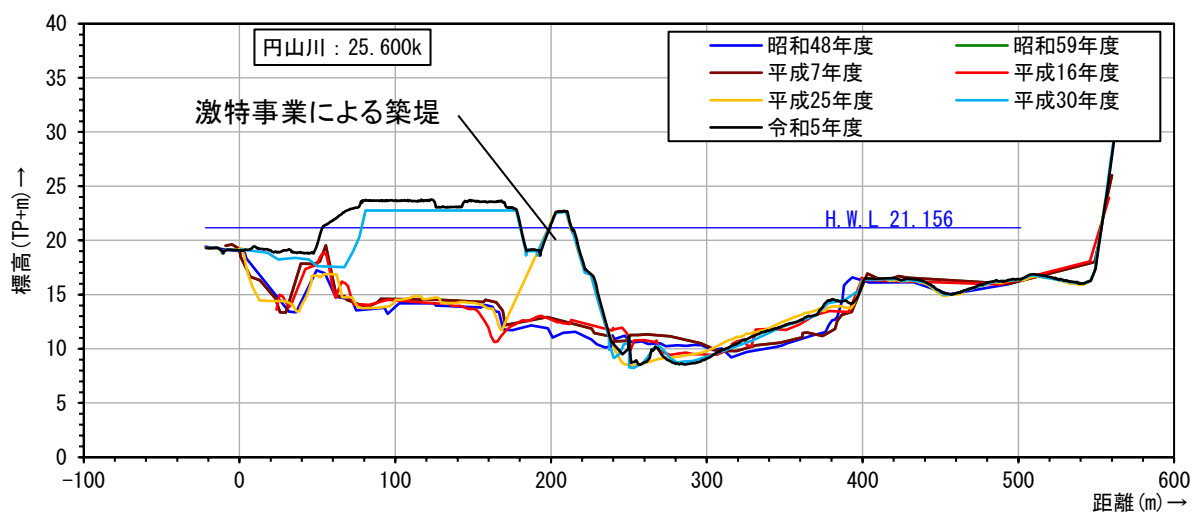
図4-3(2) 代表横断面図（円山川25k600）
