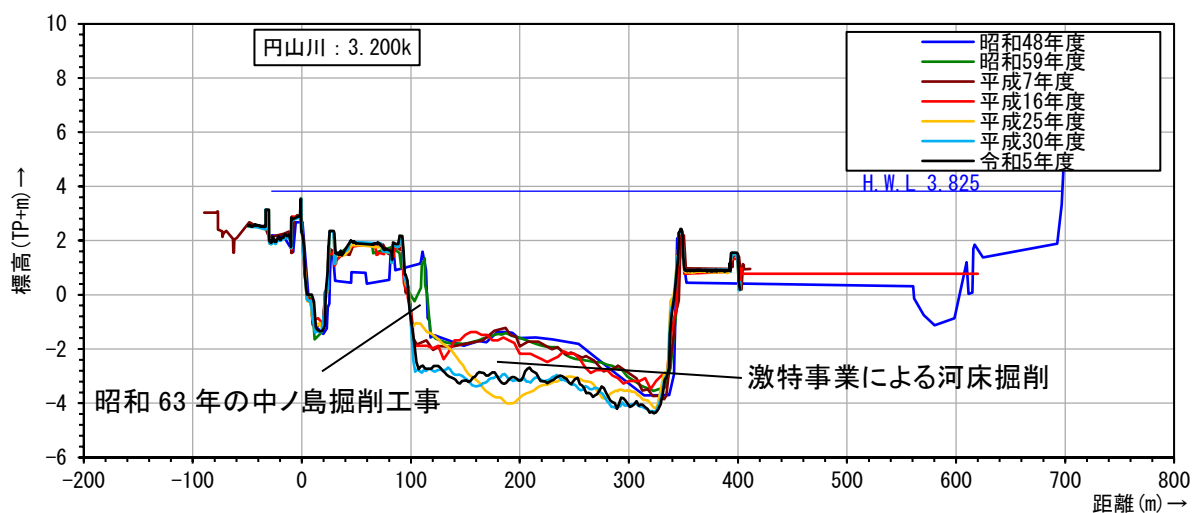
図4-3(1) 代表横断面図（円山川3k200）
