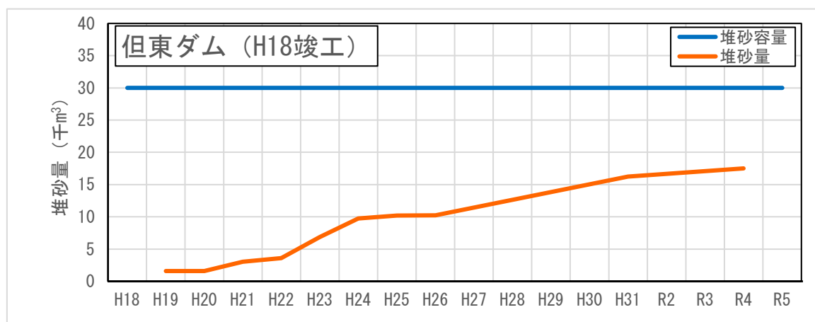
図3-2 (2) 但東ダムの堆砂状況
