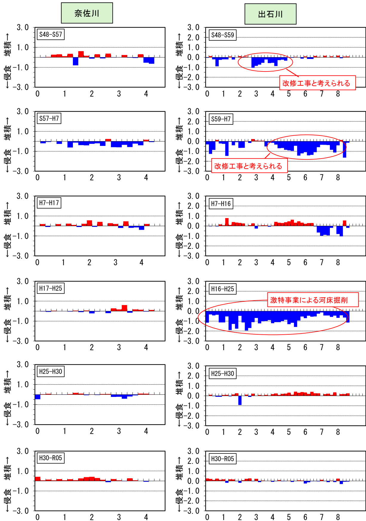
図 4-2 (2) 平均河床高変化量の経年変化図(左：奈佐川、右：出石川)
