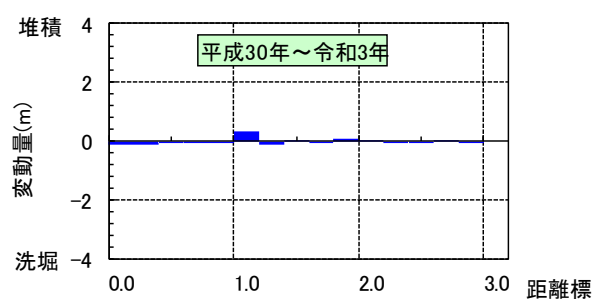
図-4.6 河床変動高の経年変化（万願寺川・東条川）
