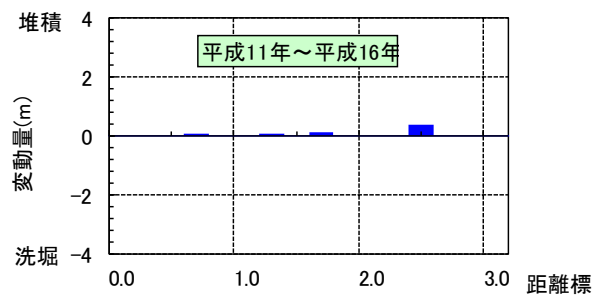
図-4.5 河床変動高の経年変化（万願寺川・東条川）
