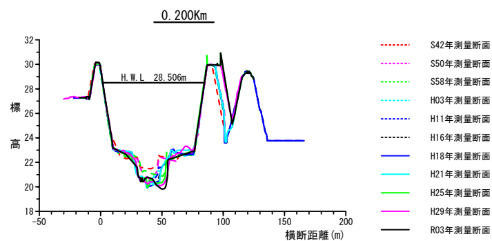
図-4.10 万願寺川（阿形橋上流 0k2）横断面図
