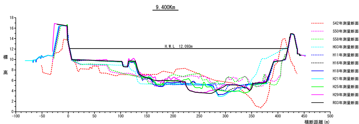
図-4.8 加古川 下流部（池尻橋上流 9k4）横断図
