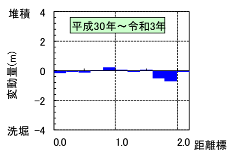
図-4.6 河床変動高の経年変化（万願寺川・東条川）
