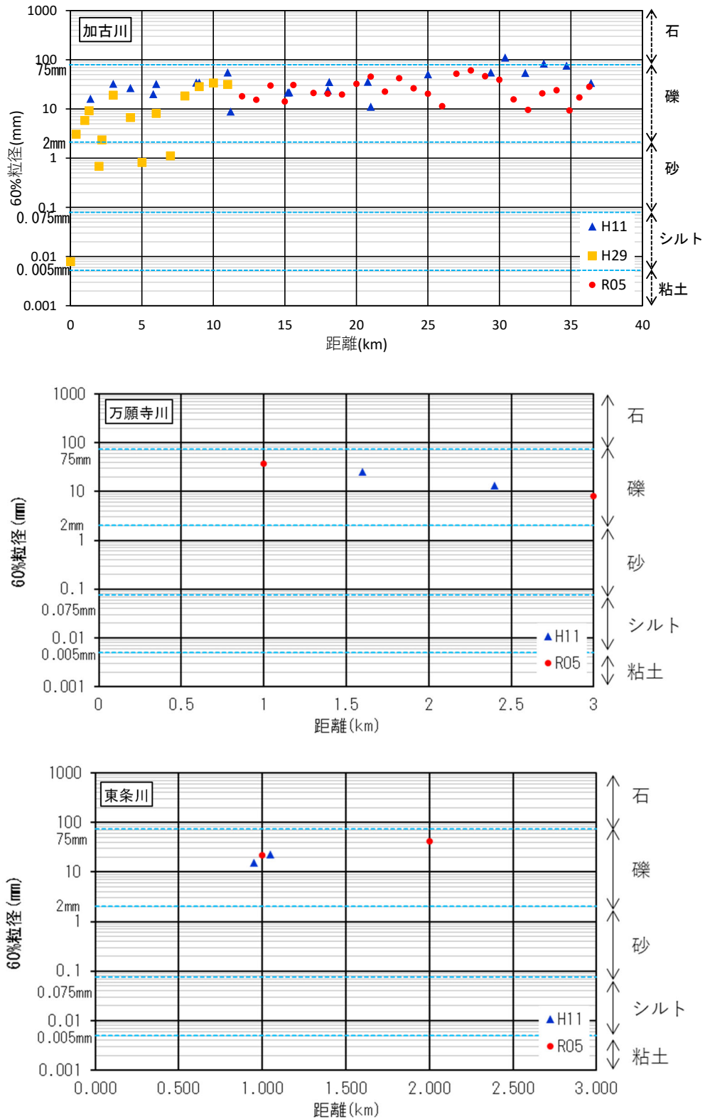
図-4.13 60%粒径の縦断分布
