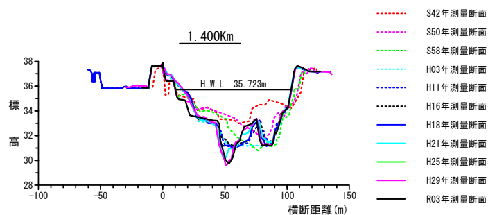
図-4.11 東条川（古川橋上流 1k4）横断面図
