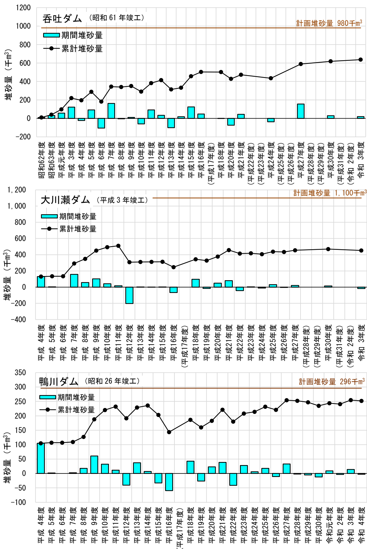
図-3.2 ダム堆砂量の経年変化
