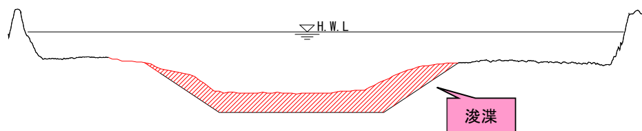
図- 5-3 河口部（0.0k）における浚渫工事実施状況（令和 3 年度の実施例）
