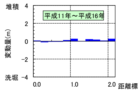
図-4.5 河床変動高の経年変化（万願寺川・東条川）
