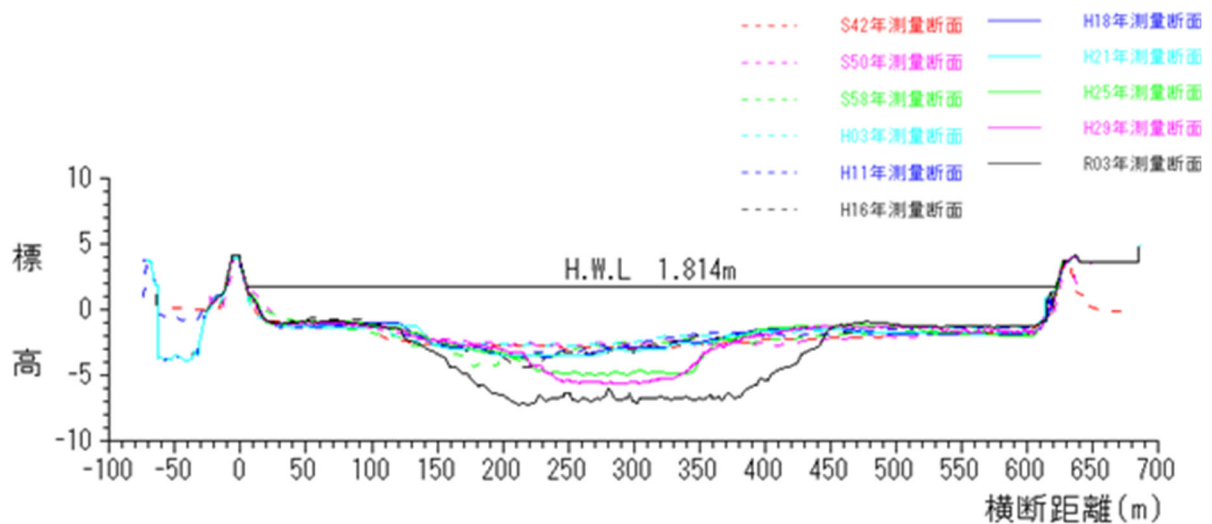
図- 5-2 河口部（0k0）の横断図
