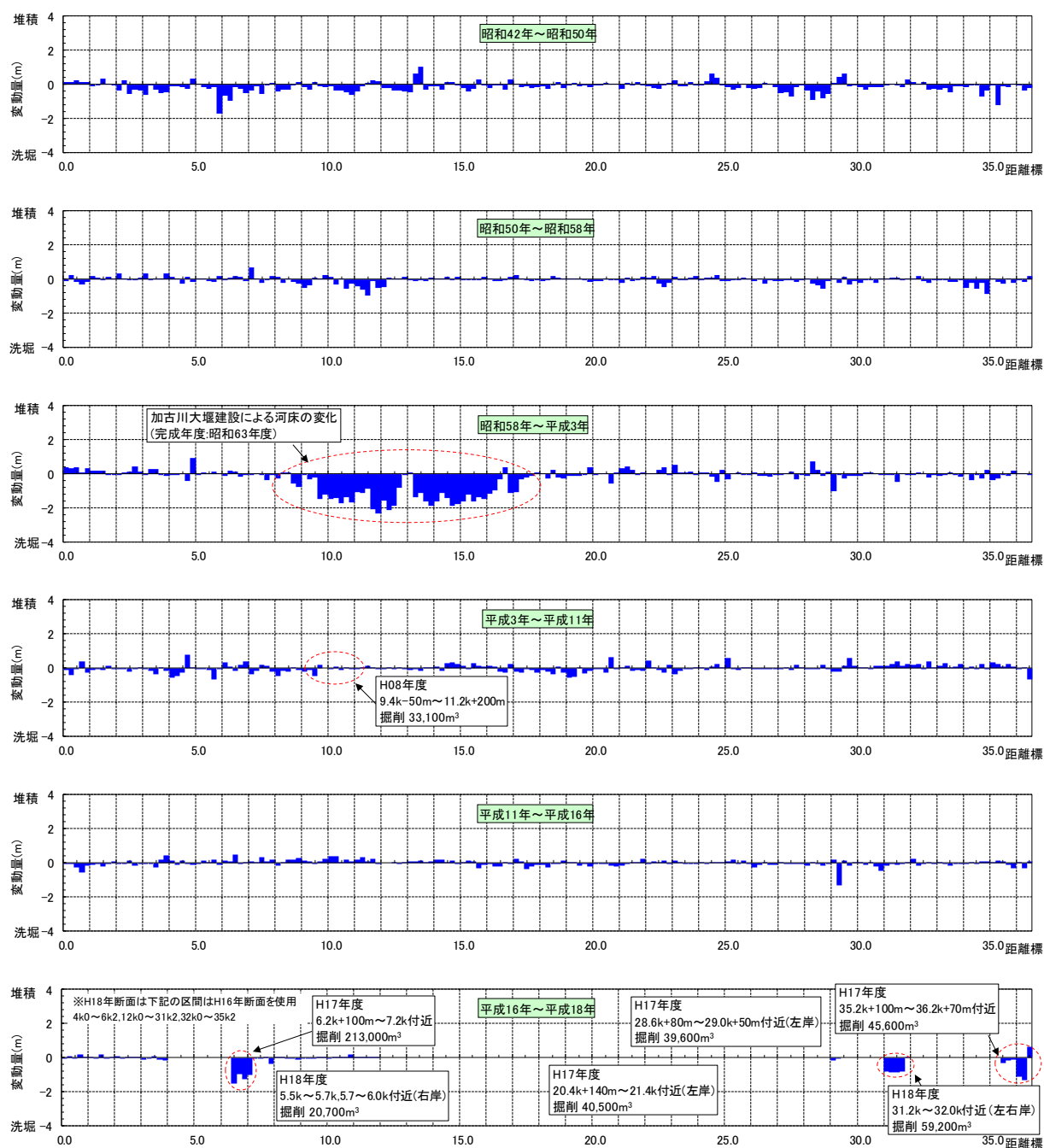
図-4.2 河床変動高の経年変化（加古川）
