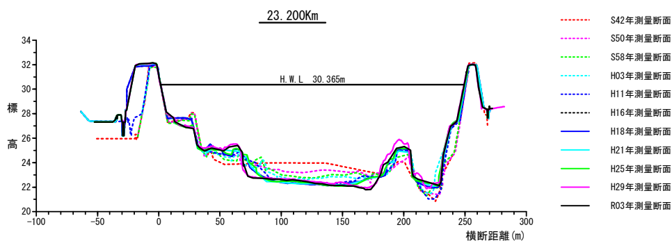
図-4.9 加古川 中流部（粟田橋上流 23k2）横断図
