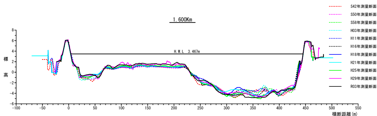
図-4.7 加古川 河口部（相生橋上流 1k6）横断図
