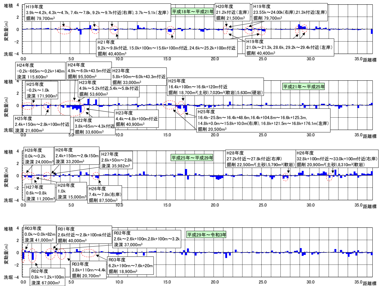
図-4.3 河床変動高の経年変化（加古川）
