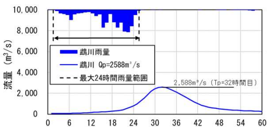
2003(H15).8.15(計画決定洪水)
