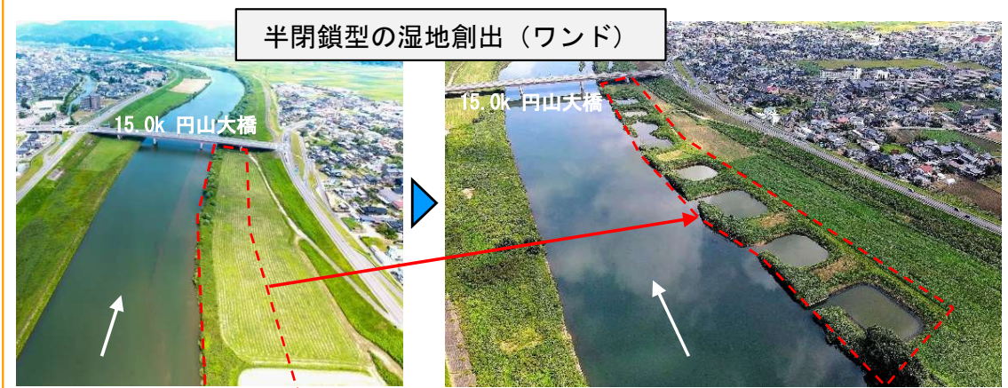
改良前（円山大橋上流） 改良後（円山大橋上流）
