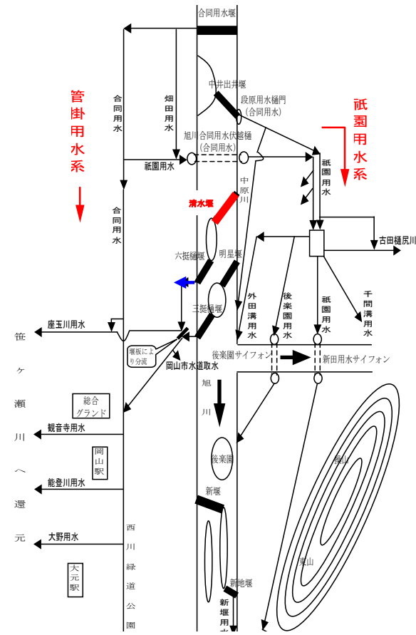
旭川合同用水水路系統模式図
