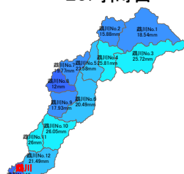
計算開始から 23時間目
