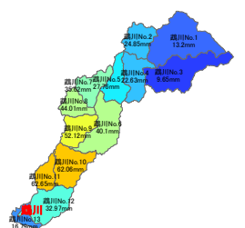
計算開始から 22時間目
