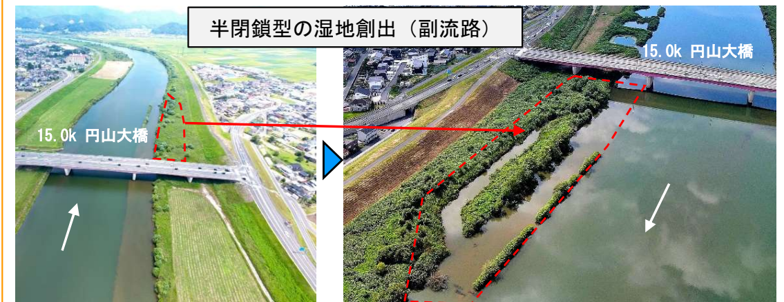
改良前（円山大橋下流） 改良後（円山大橋下流）
