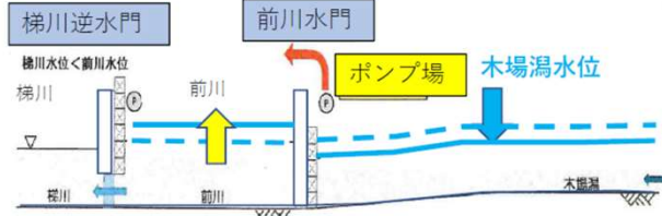
事前排水イメージ図 （梯川水位<前川水位の場合）
