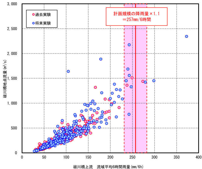
アンサンブル将来予測降雨波形データを用いた検討
