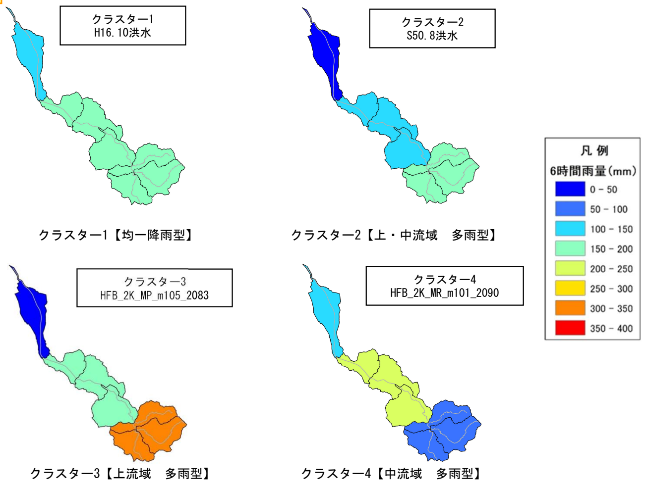
降雨寄与率の分析により主要洪水群に不足する降雨波形
