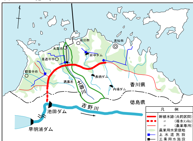
図 5.1.3 香川用水事業概略図
