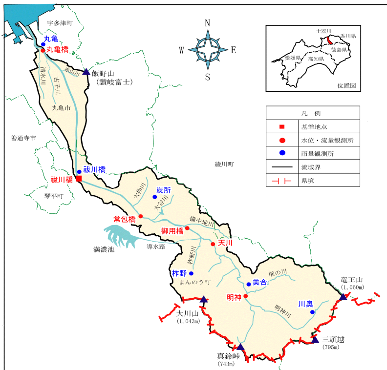
図 9.4.1 水位・流量・雨量観測所位置
