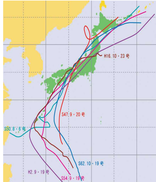
図 4.1.1 台風経路図
