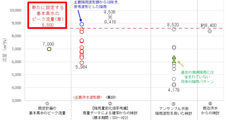
基本高水の設定に係る総合的判断（福島地点）
