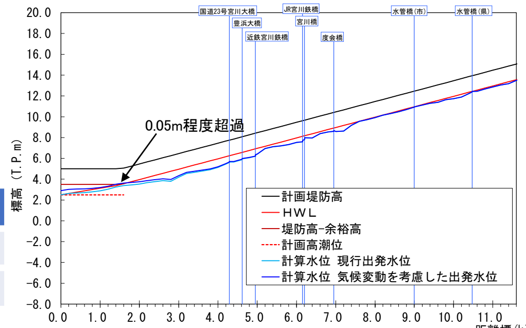
宮川計画高水流下時水位縦断面図
