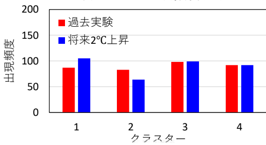
アンサンブル降雨波形の出現頻度(クラスター別)
