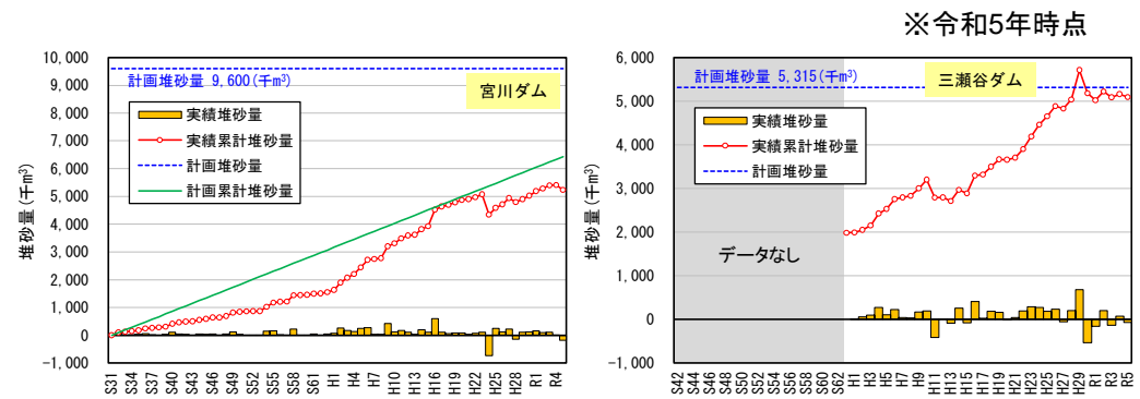
ダム堆砂状況の推移
