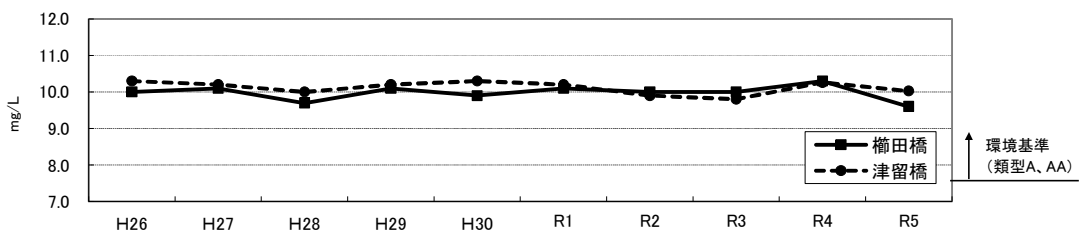
図 6-5 溶存酸素量 (DO)
