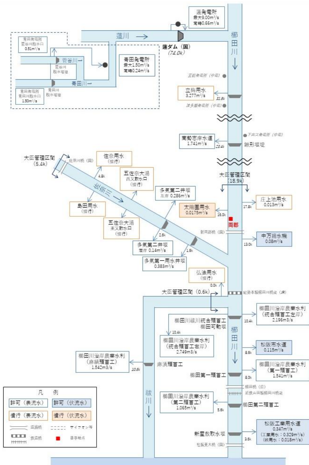
図 5-1 櫛田川水系 水利使用模式図（主な水利権を記載）
