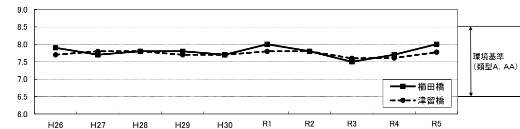
図 6-2 水素イオン濃度 (pH)
