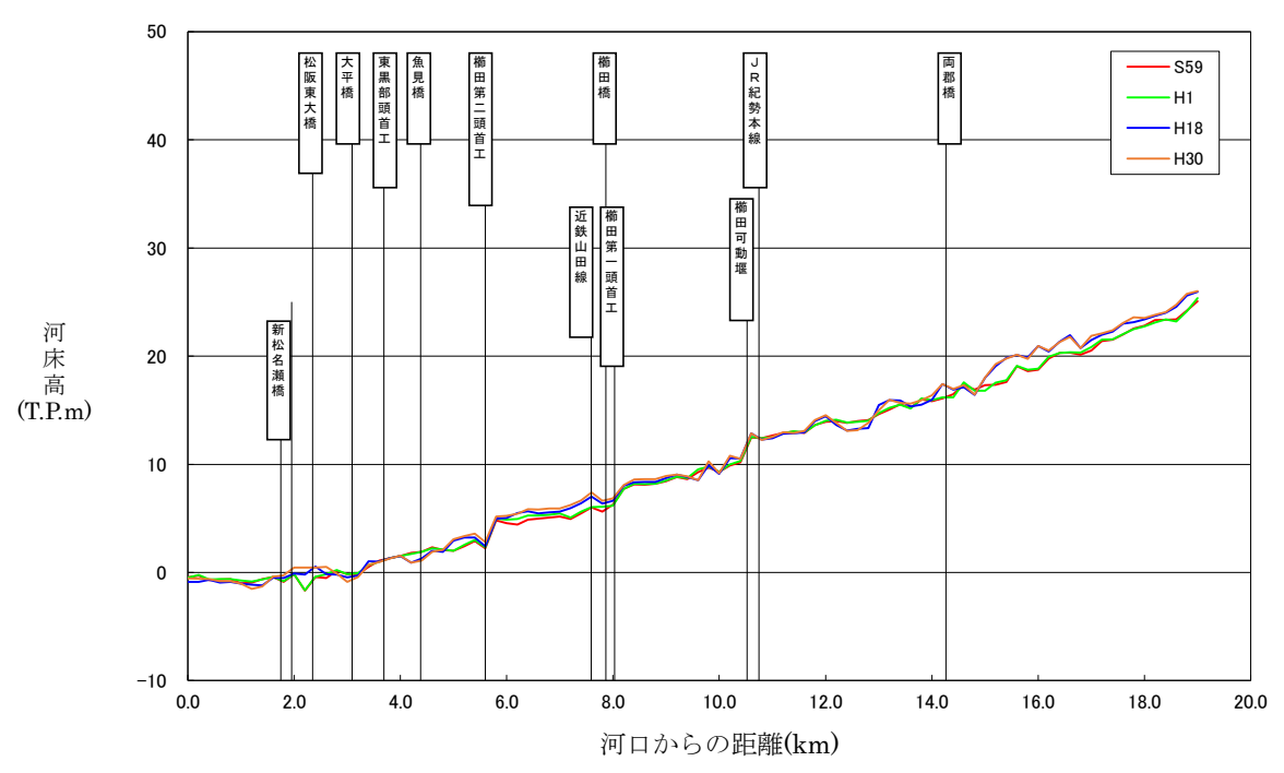
図 8-2 榑田川平均河床縦断図（大臣管理区間）
