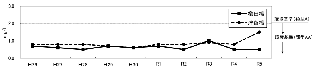
図 6-3 生物化学的酸素要求量 (BOD) [75%値]
