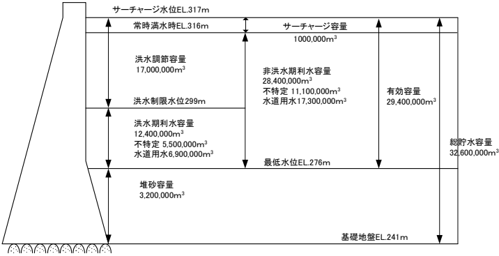
図 4-3 貯水池容量配分図
