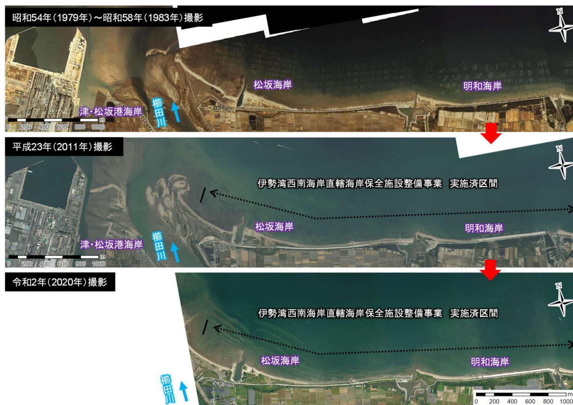
図 5-3 河口部平面形状の経年変化状況
