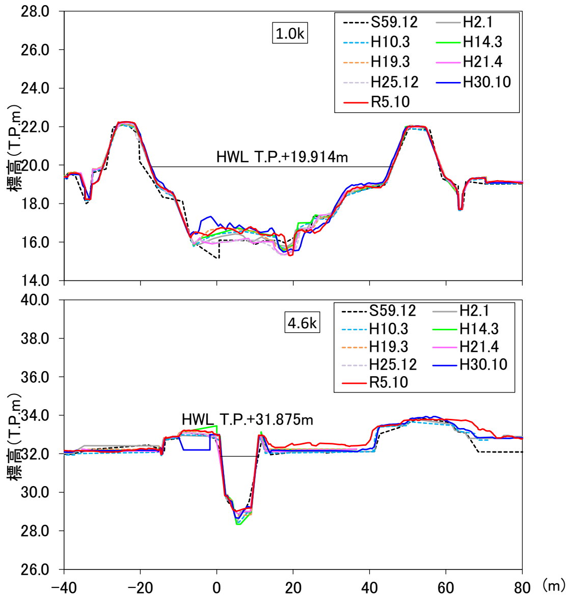
図 4-8 横断形状の経年変化状況（佐奈川）
