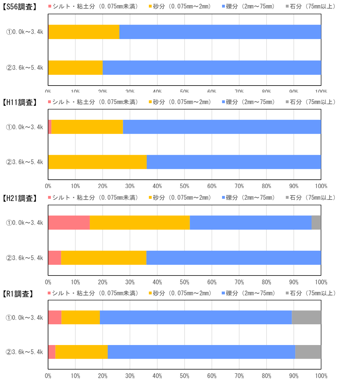
図 4-10 河床材料の粒度分布の経年変化 (佐奈川)
