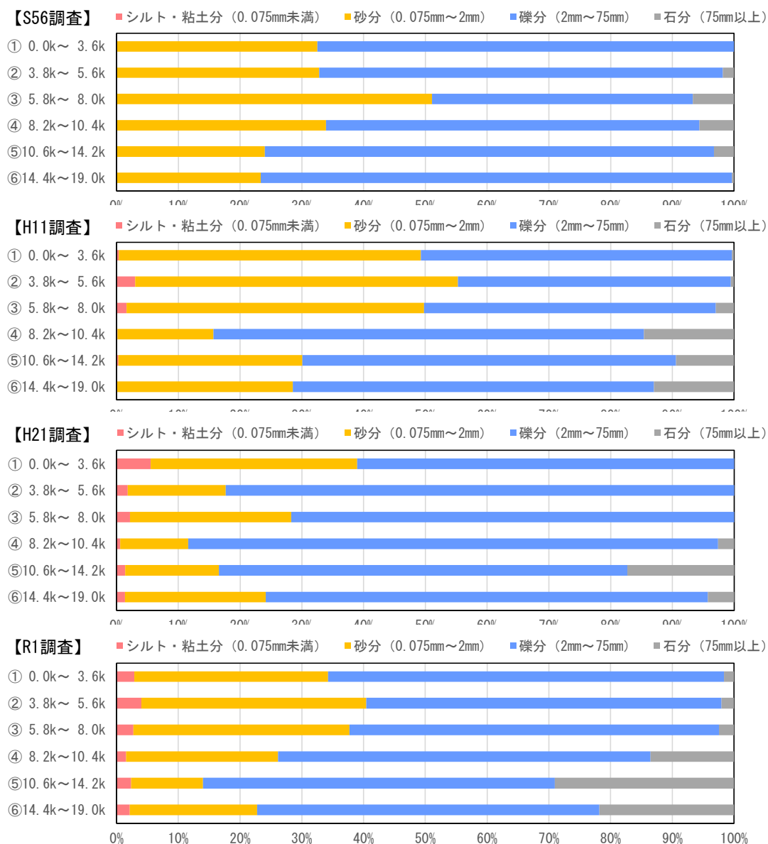
図 4-9 河床材料の粒度分布の経年変化（櫛田川）
