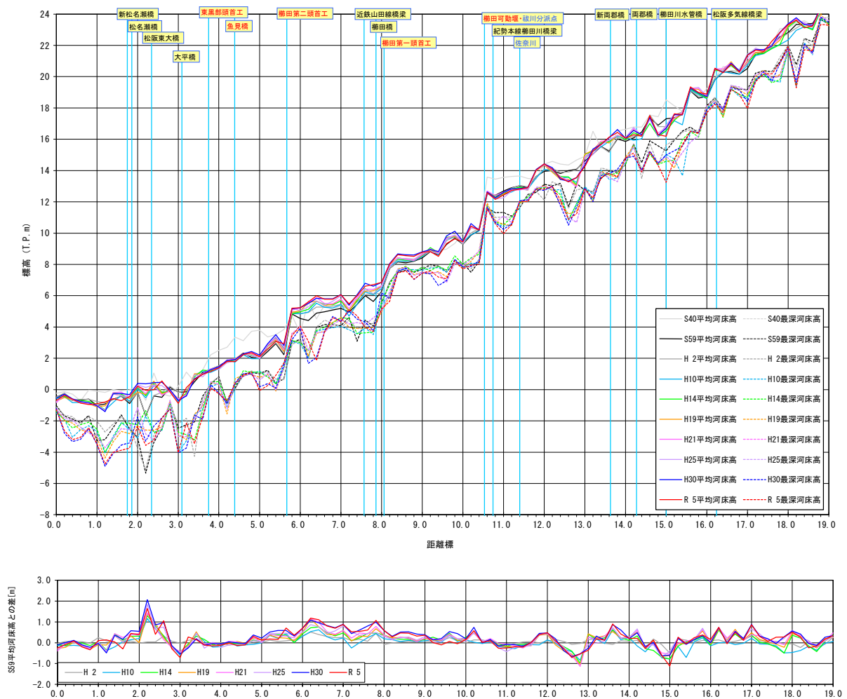
図 4-4 河床変動縦断図（櫛田川）
