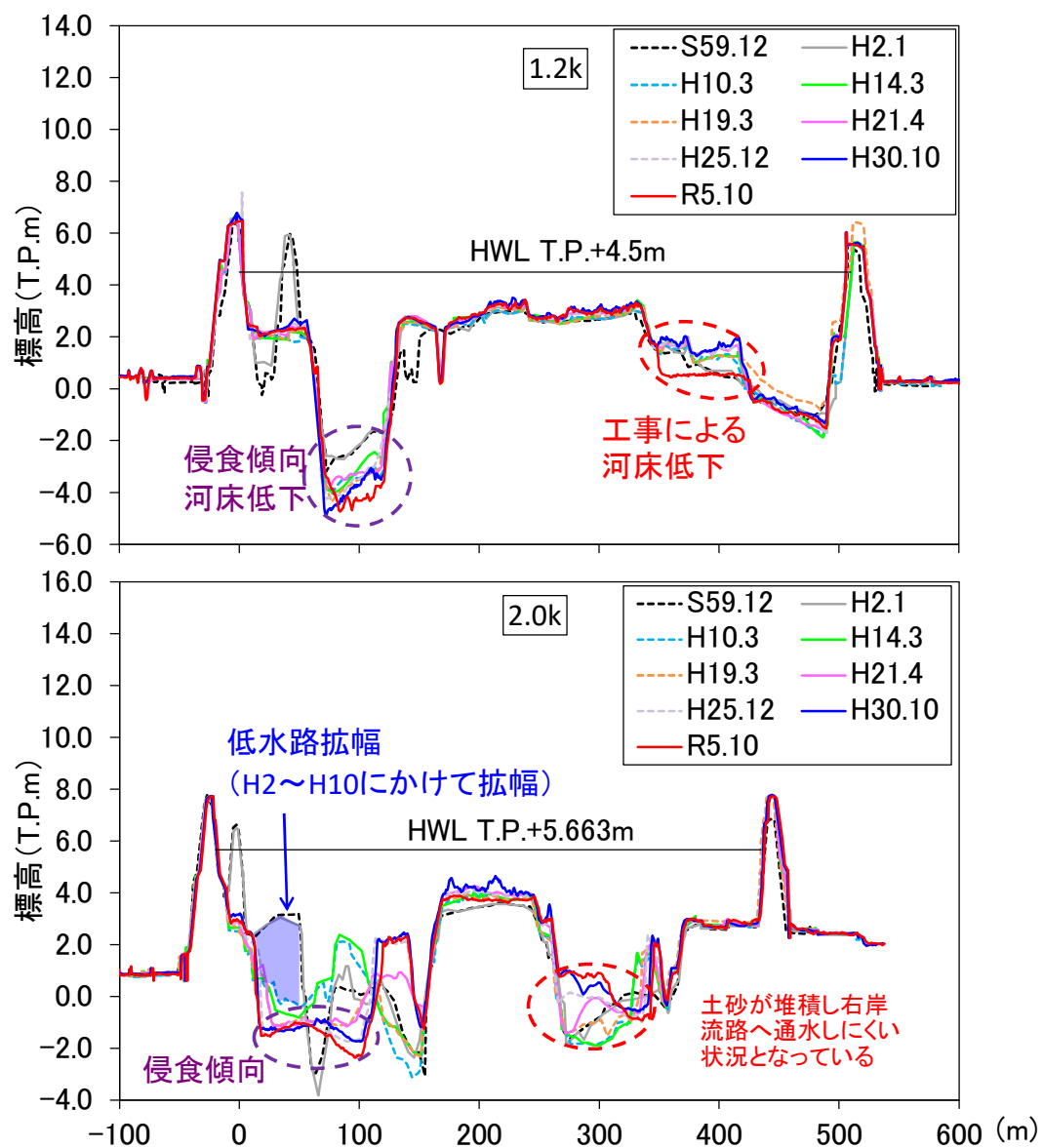
図 4-7(1) 横断形状の経年変化状況（櫛田川）
