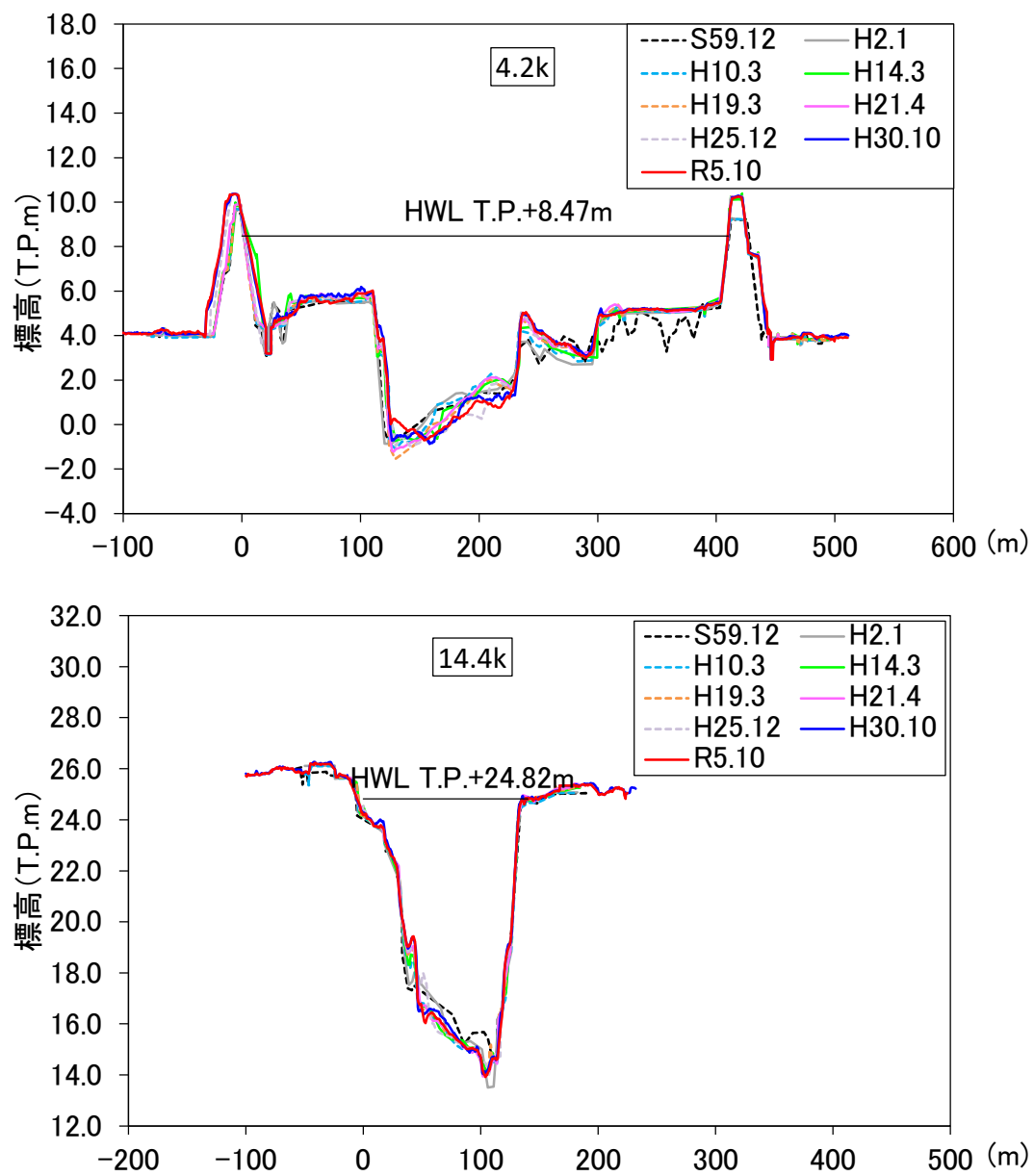
図 4-7(2) 横断形状の経年変化状況（櫛田川）
