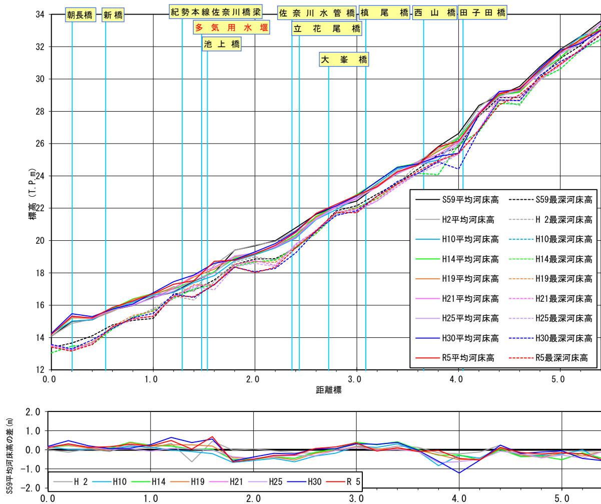
図 4-6 河床変動縦断図（佐奈川）
