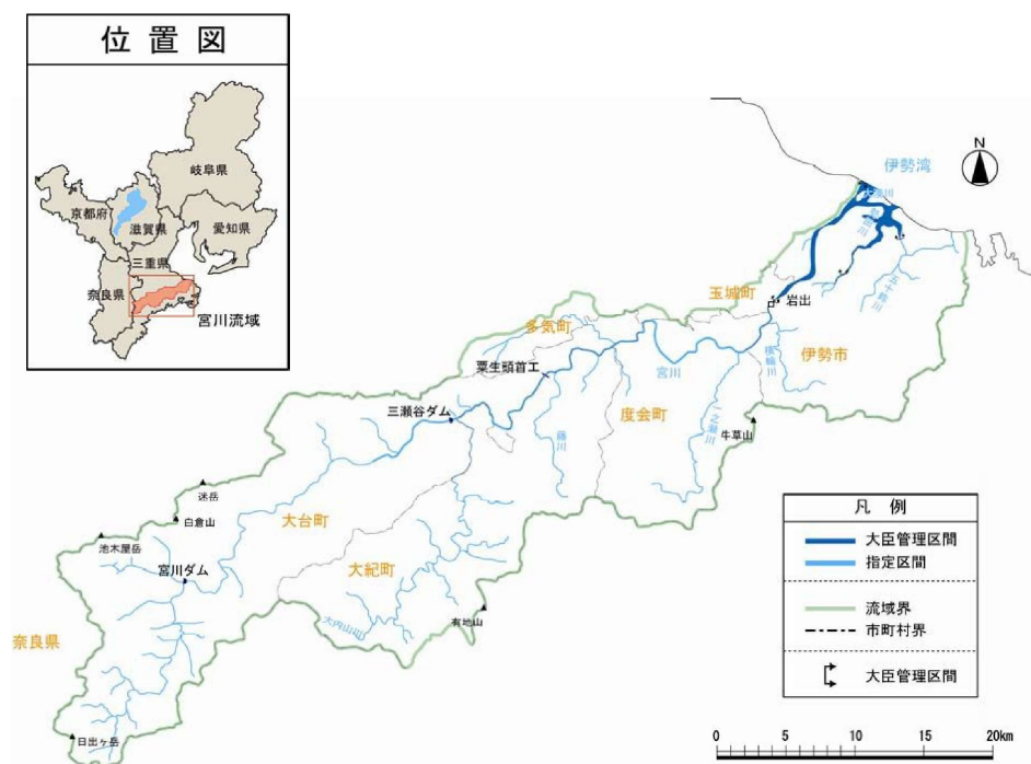
図 9-1 宮川管理区間概要図
