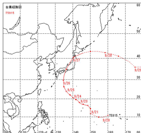
図 4-3 台風経路図
