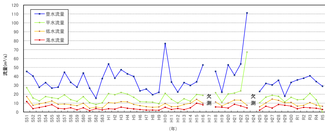
図 6-2 岩出地点流量変化 (豊水流量・平水流量・低水流量・渇水流量)
