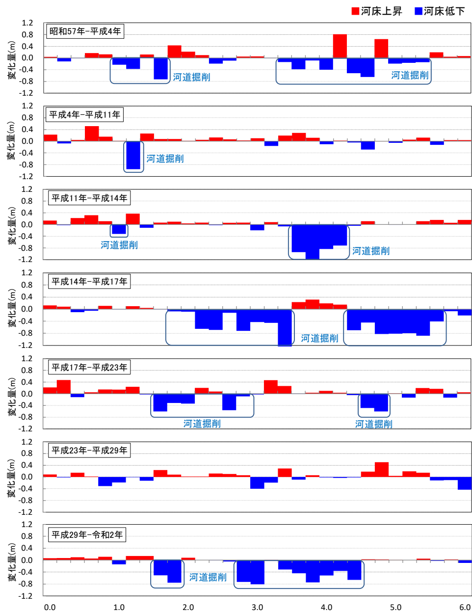
図 8-5 勢田川 河床変動量の経年変化
