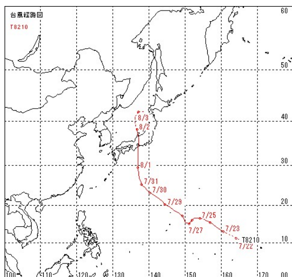
図 4-8 台風経路図
