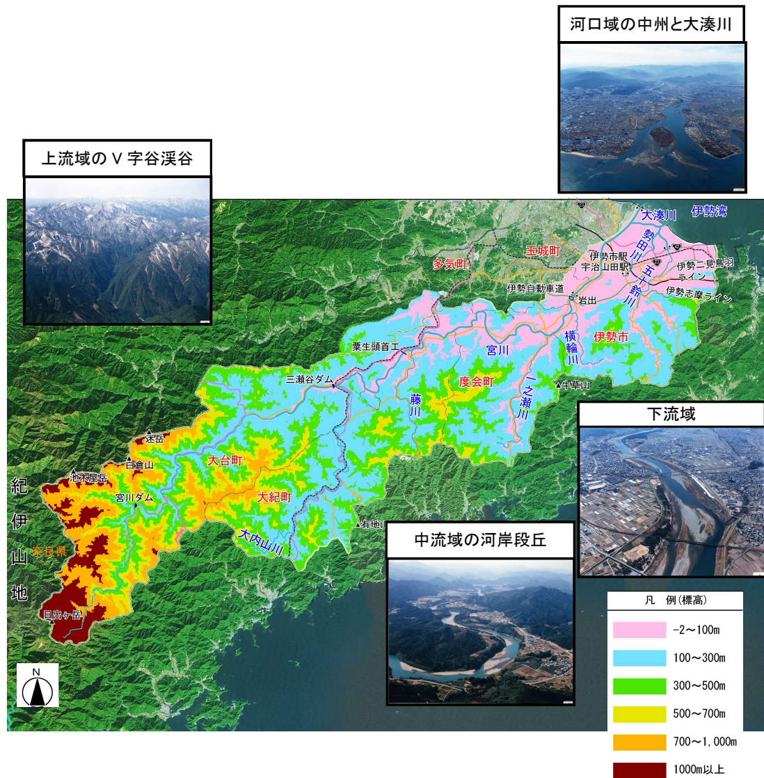
図 1-2 宮川流域地形図
