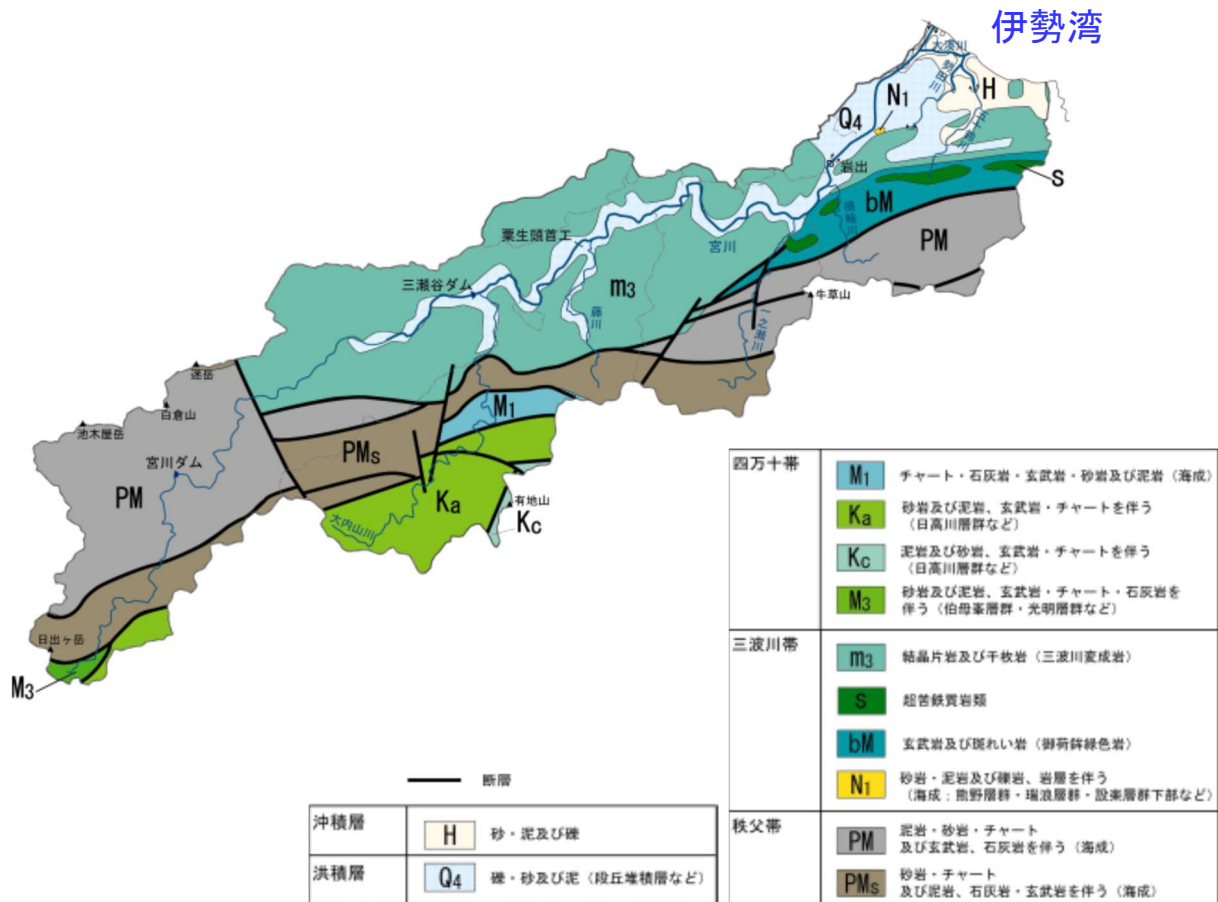
図 1-3 宮川流域地質図
