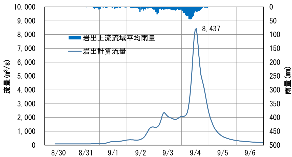
図 1.24 平成 23 年 9 月洪水 推定結果（基準地点岩出）
