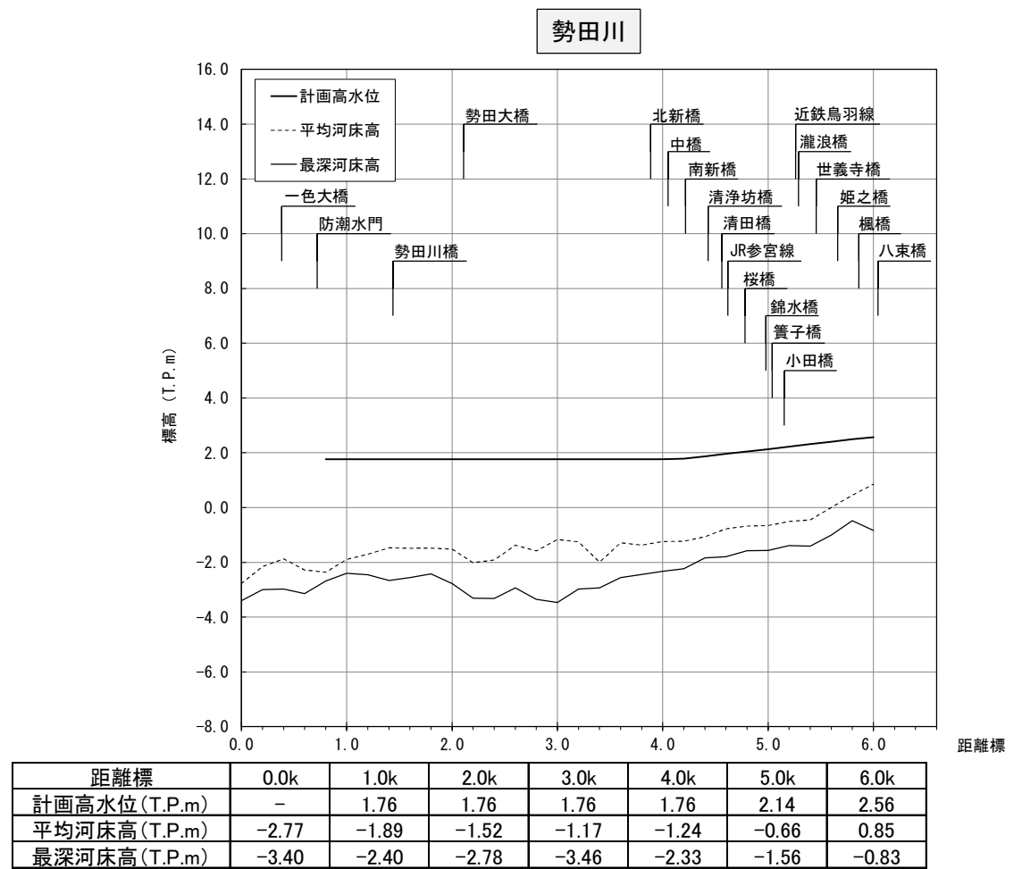
図 5.2 計画縦断図（五十鈴川、勢田川）
