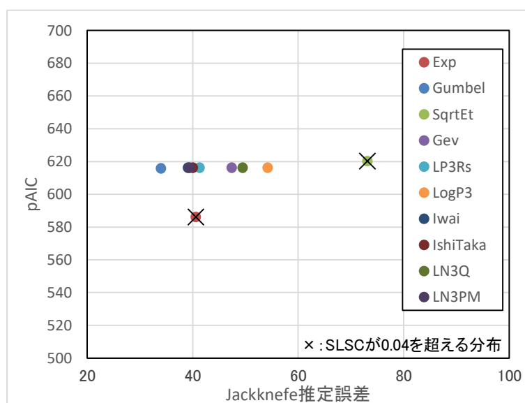
図 1.13 pAIC と Jackknife 推定誤差の関係 (基準地点岩出)
