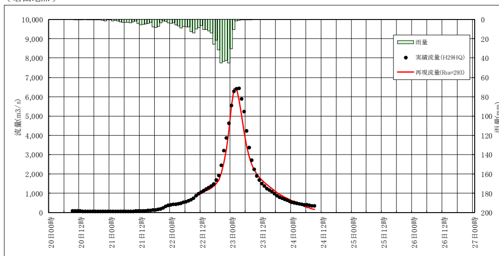
図 1.5(3) 再現ハイドログラフ (平成29年10月23日洪水)
