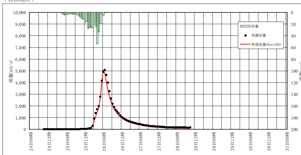
図 1.5(2) 再現ハイドログラフ (平成27年8月26日洪水)
