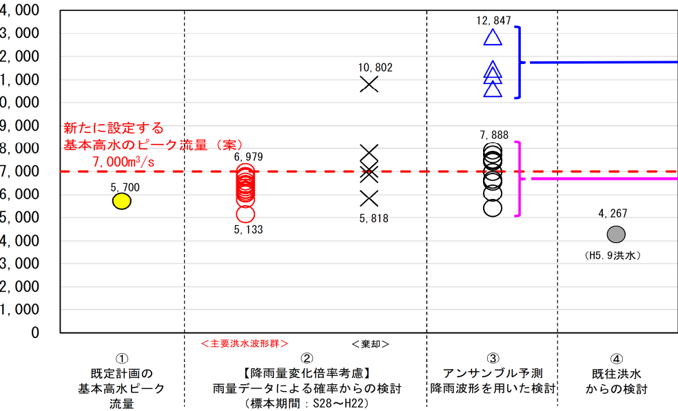
基本高水の設定に係る総合判断（基準地点府内大橋）
