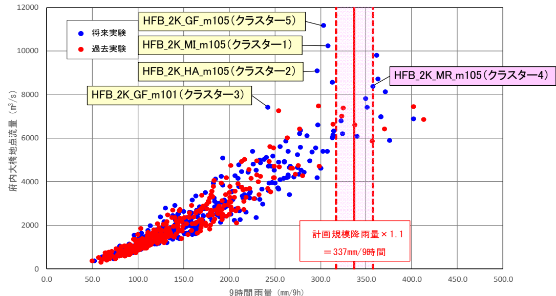
基本高水の設定に係る総合判断（基準地点府内大橋）
