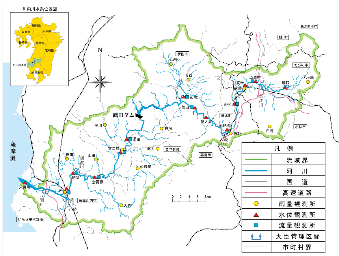
図 9-2 川内川流域水文観測所位置図
