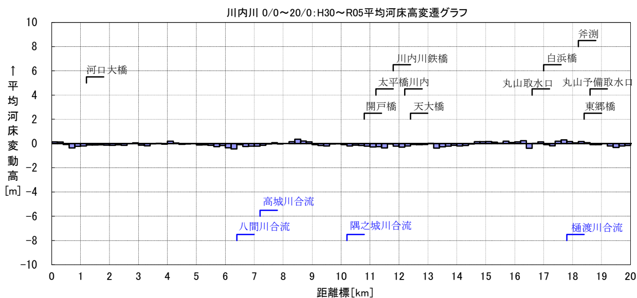
図 8-3 (2) 平均河床高変動量経年変化図 (川内川下流区間 : 0.0～20.0k)
