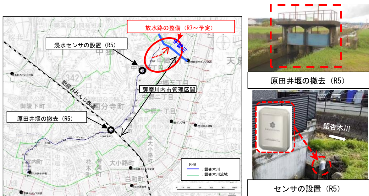
図 4-1 薩摩川内市による内水対策の事例
