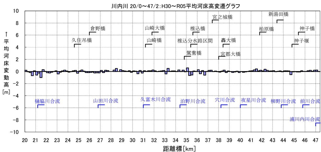
図 8-3(4) 平均河床高変動量経年変化図 (川内川中流区間 : 20.0～47.2k)
