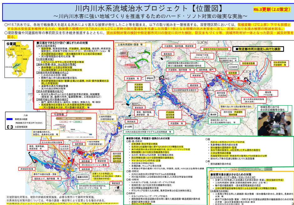
図 9-3 川内川水系流域治水プロジェクト 2.0
