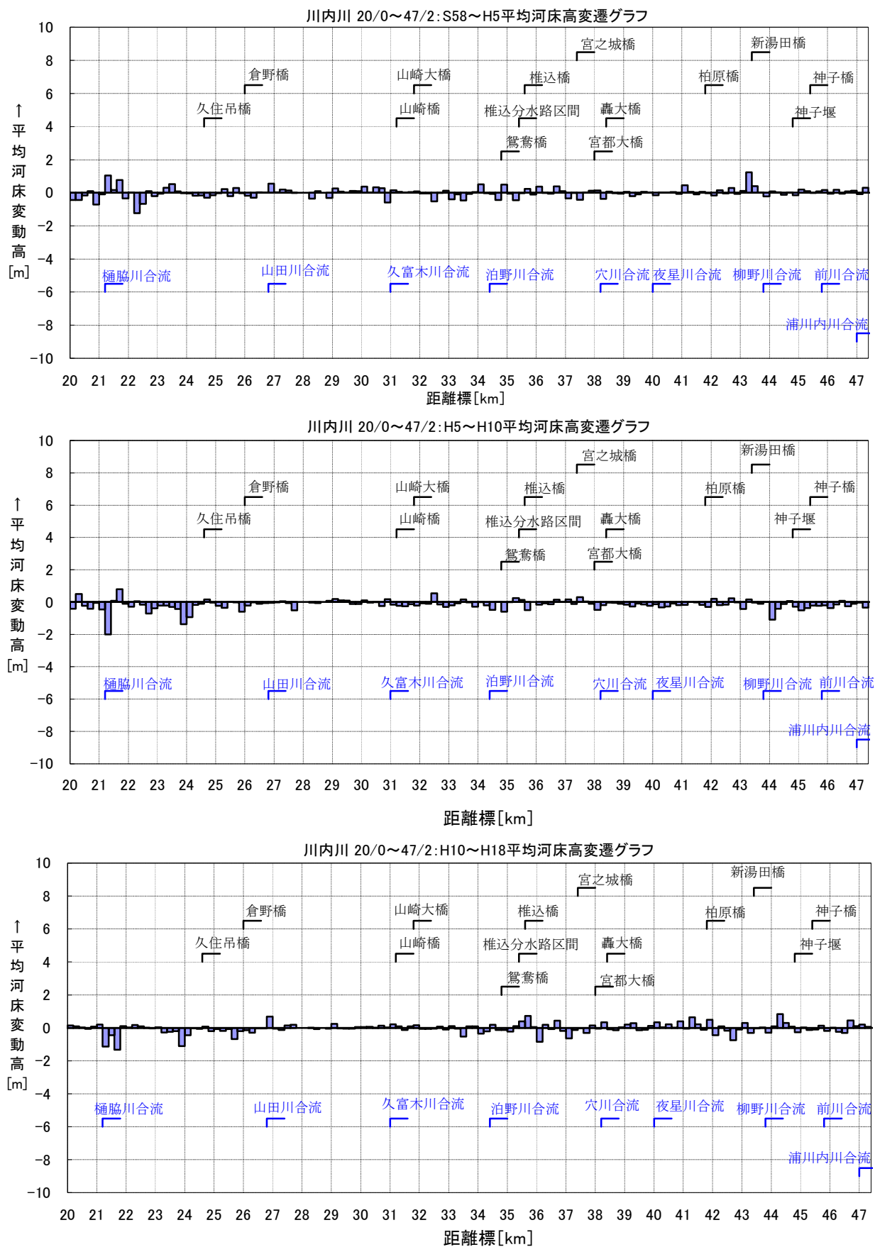
図 8-3 (3) 平均河床高変動量経年変化図 (川内川中流区間 : 20.0~47.2k)
