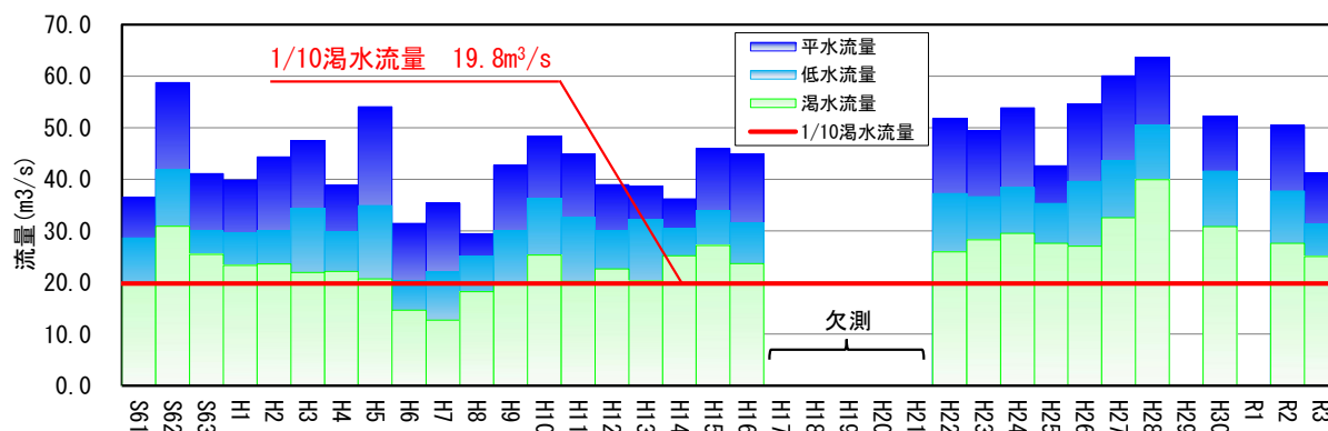
図 6-1 川内川 倉野橋地点流況図
