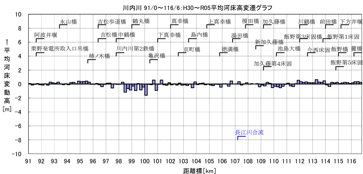
図 8-3 (8) 平均河床高変動量経年変化図 (川内川上流区間 : 91.0～116.6k)
