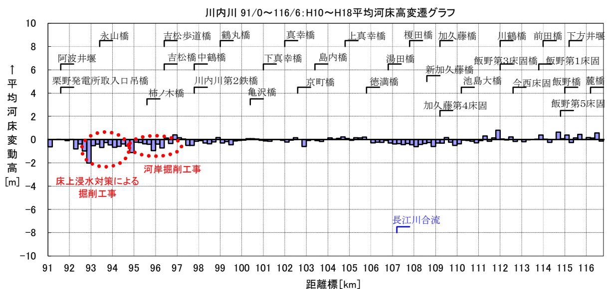
図 8-3 (7) 平均河床高変動量経年変化図 (川内川上流区間 : 91.0～116.6k)
