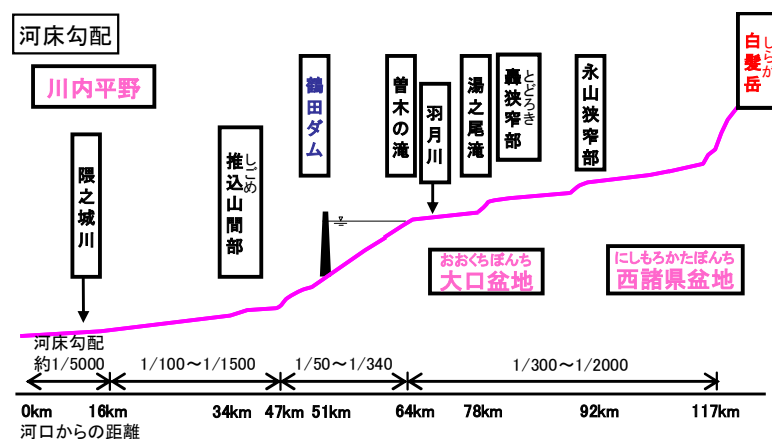
図 1-3 (1) 川内川縦断図
