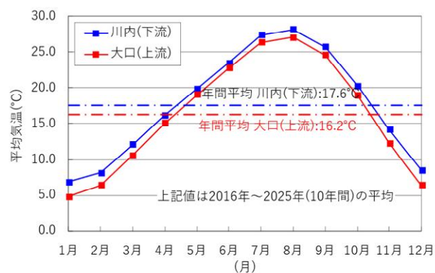
図 1-6 代表地点の月別平均気温 (出典：気象庁資料)
