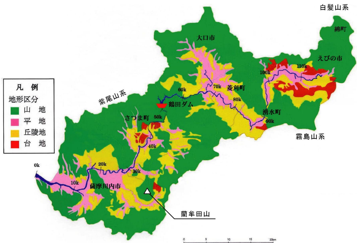
図 1-2 川内川地形分類図
