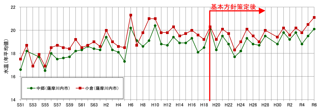
図 2-6 年平均水温の変化
