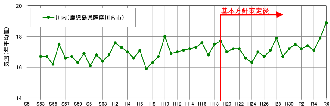
図 2-5 年平均気温の変化
