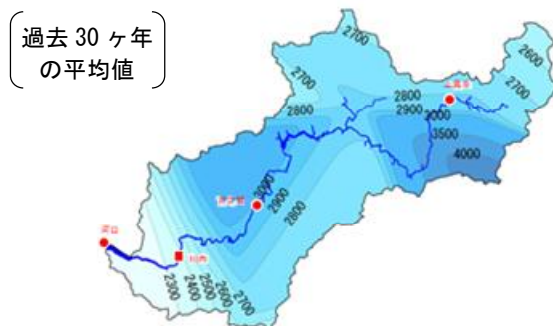
年間降水量分布図
