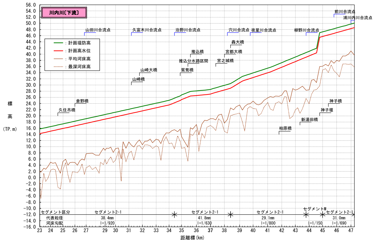
図 8-2(1) 川内川河床縦断図
