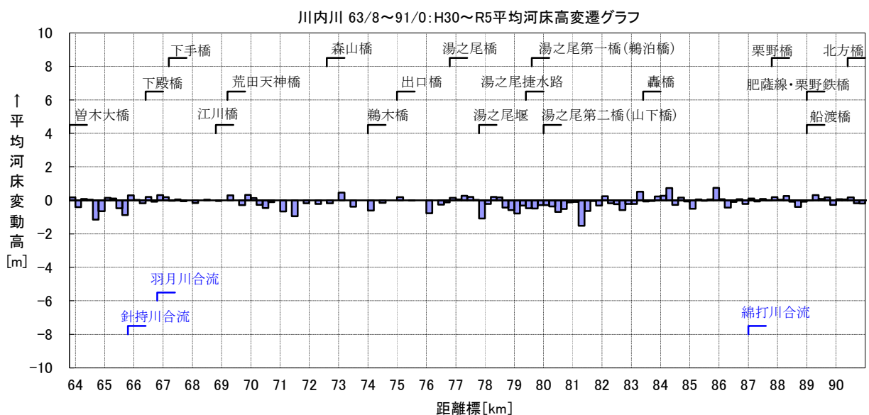
図 8-3(6) 平均河床高変動量経年変化図 (川内川上流区間 : 63.8～91.0km)
