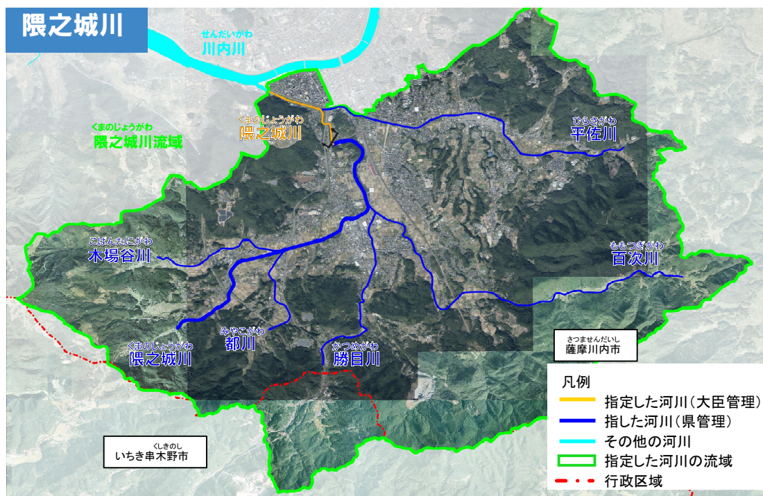
図 4-6 特定都市に指定した河川の流域図（隈之城川）
