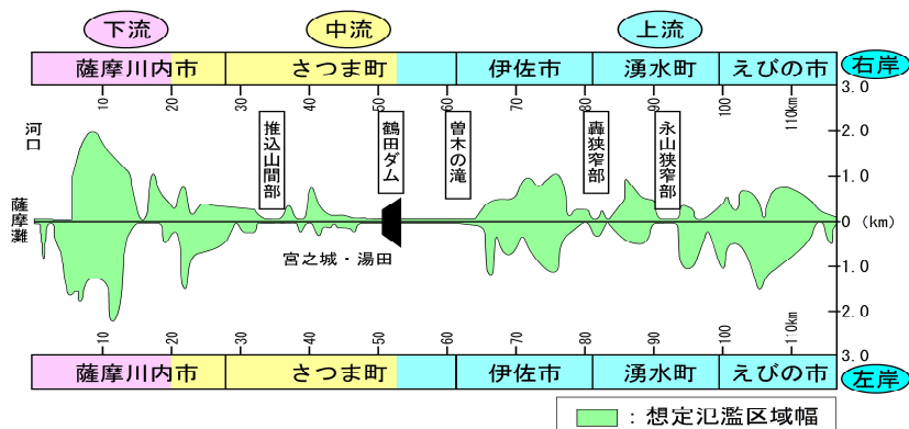
図 1-3 (2) 川内川氾濫原縦断図
