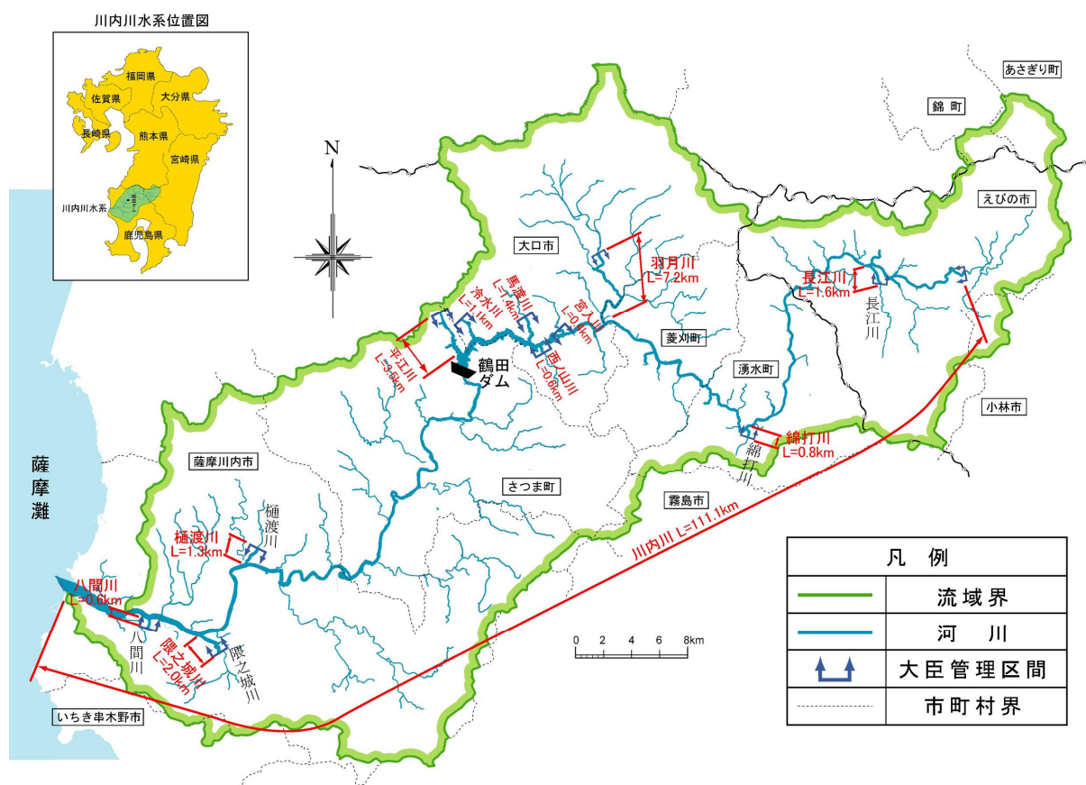
図 9-1 川内川水系の大臣管理区間
