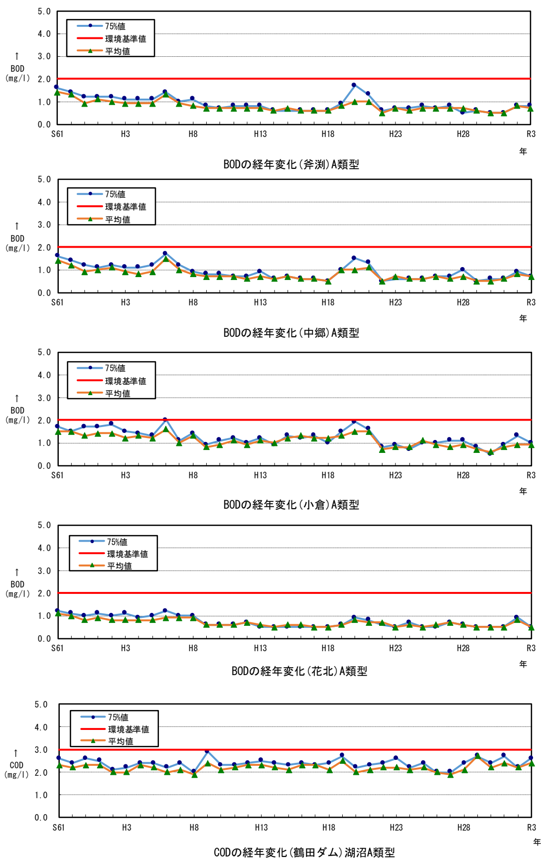
図 6-3(2) 水質観測地点の BOD (COD) 75%値経年変化図
