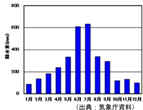
図 1-7 川内川流域平均年間降雨量及び平均月別降雨量
