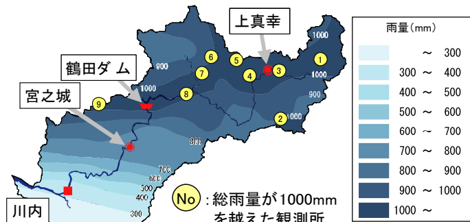
〔 川内川流域総雨量図 〕
