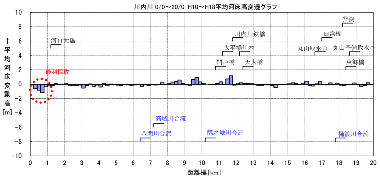
図 8-3(1) 平均河床高変動量経年変化図 (川内川下流区間 : 0.0～20.0k)
