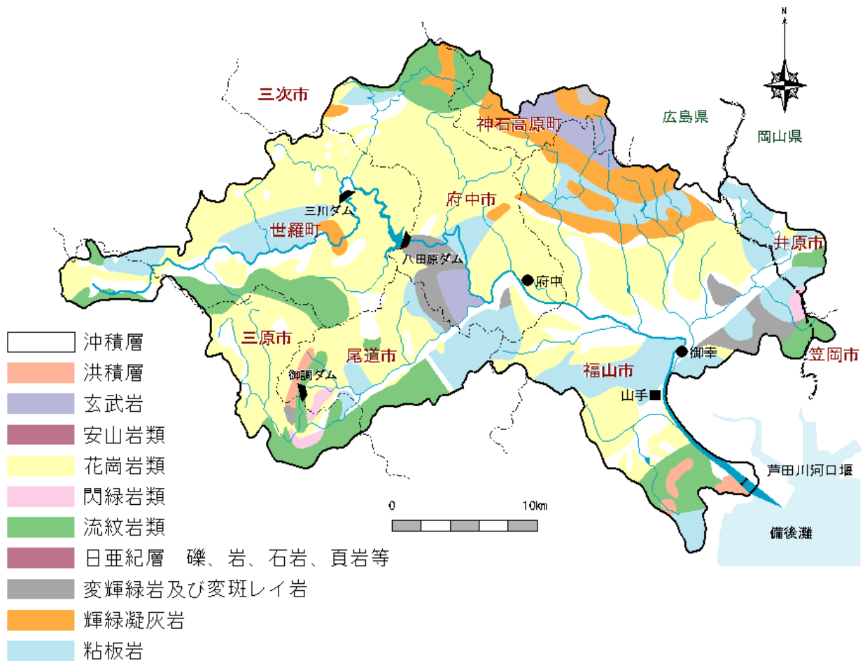
図 1-6 芦田川流域の地質図
