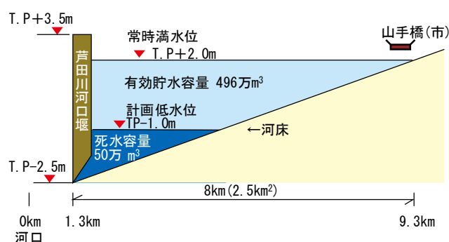
図 9-3 芦田川河口堰の様子、貯水池容量配分図
