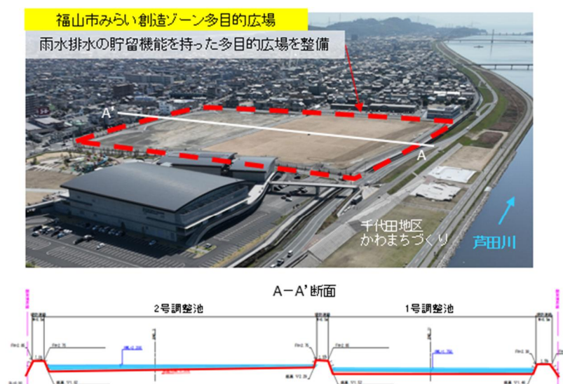
雨水貯留施設（福山市） 雨水貯留施設の整備
