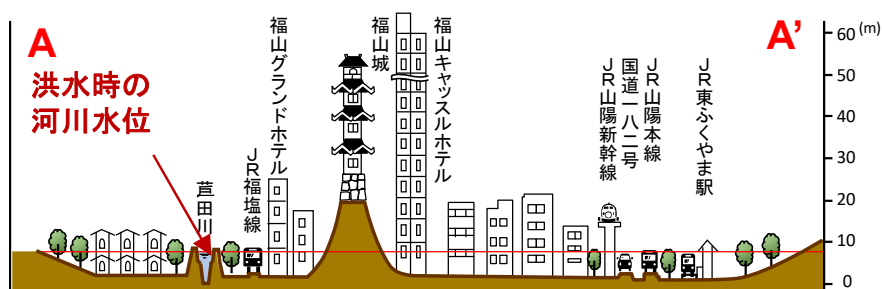
図 1-4 河床高と堤内地盤高比較図
