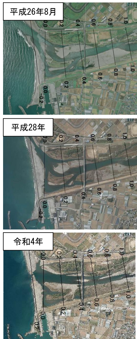
図 8-11 (2) 河口砂州の形状の経年変化
