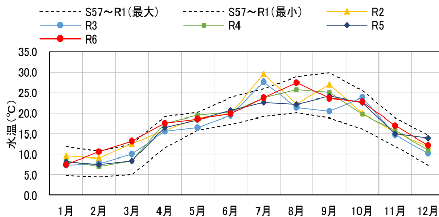
図 2-39 水温（深淵）の経月変化
