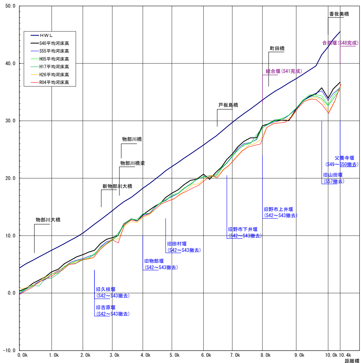
図 8-9 平均河床高縦断図の経年変化
