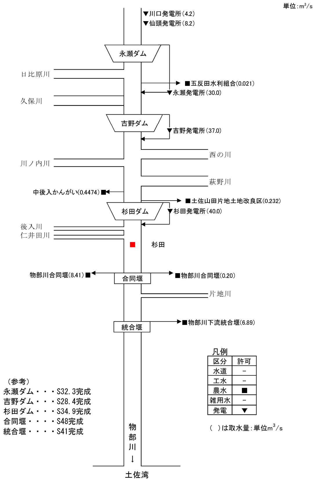
図 5-4 水利用の現状模式図 (物部川)
