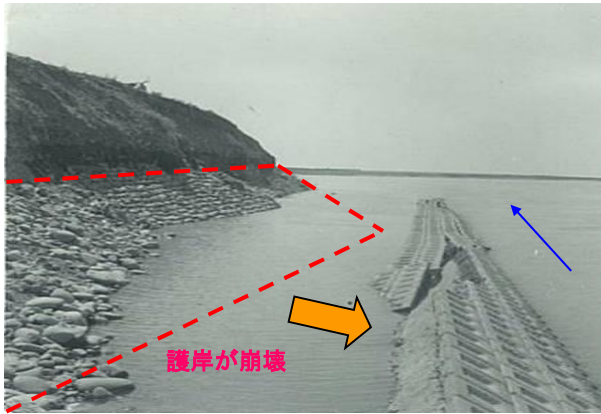
昭和38年（1963年）8月洪水での局所洗掘による護岸崩壊
