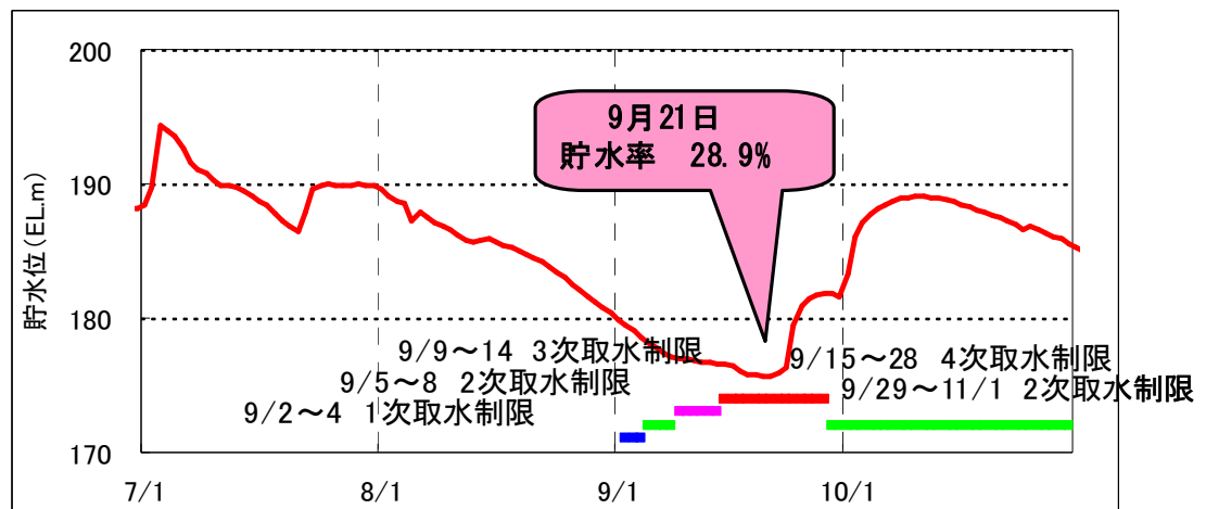
図 5-5 永瀬ダム渇水運用状況図（平成 7 年(1995 年)）
