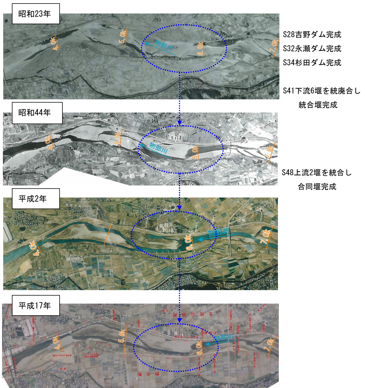
図 8-8(1) 流路の固定化の進行状況 (4.0k～7.0k 付近)
