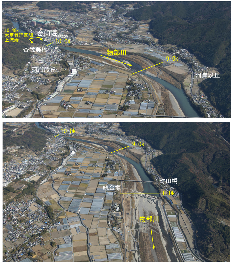
図 8-4 統合堰～合同堰
