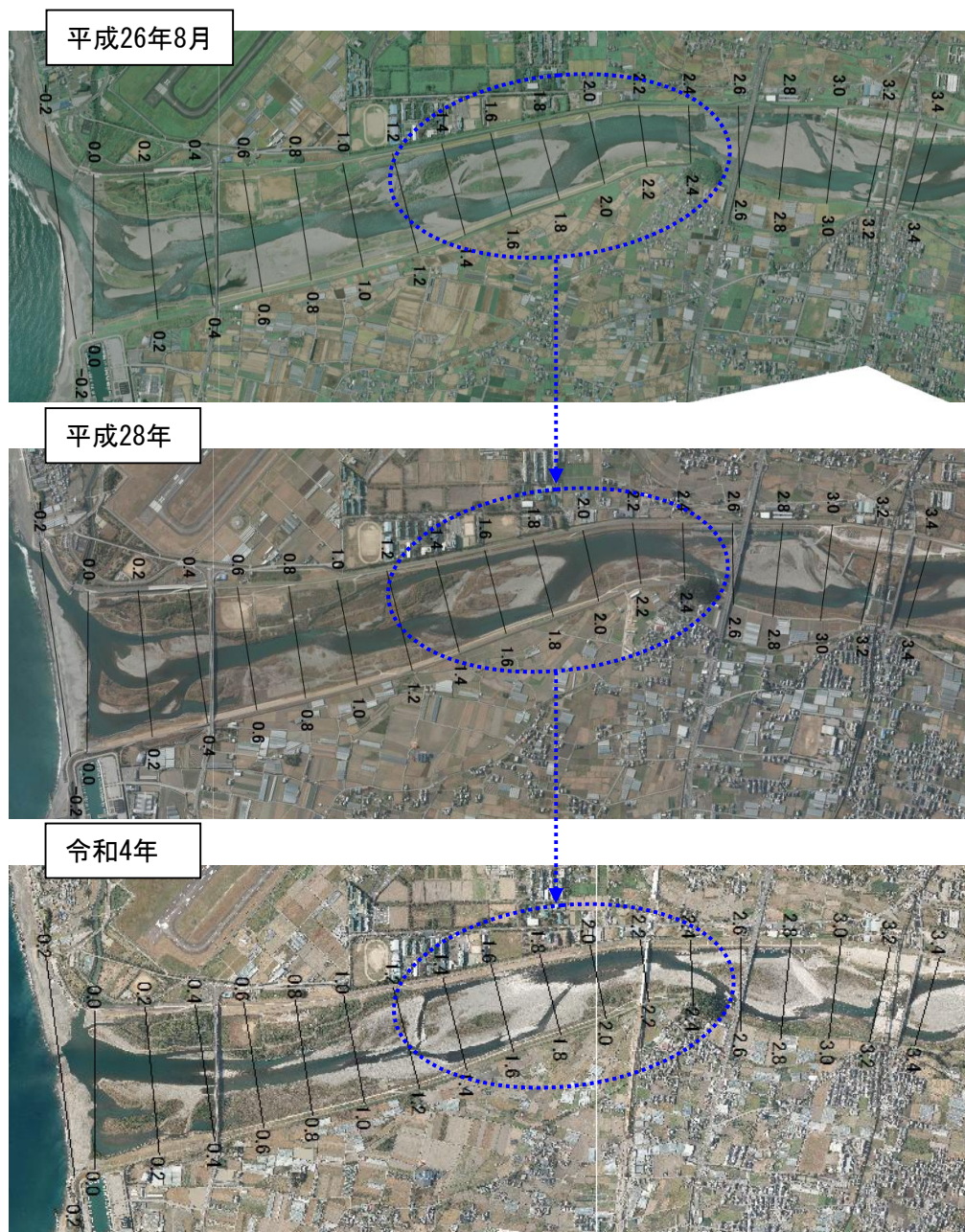
図 8-7(3) 流路の固定化の進行状況 (1.0k~3.0k 付近)
