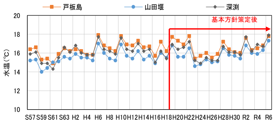
図 2-38 水温（年間平均値）の経年変化
