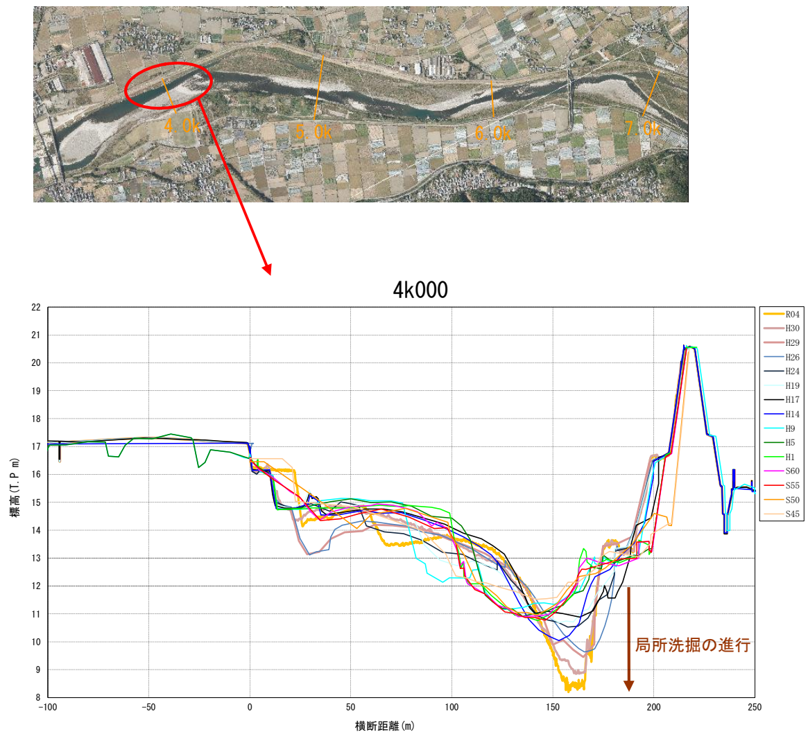
図 8-10 水衝部（4.0k 地点）の横断形状経年変化
