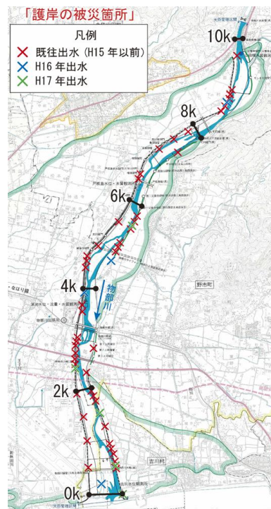
図 4-3(1) 既往洪水での護岸等被災状況
