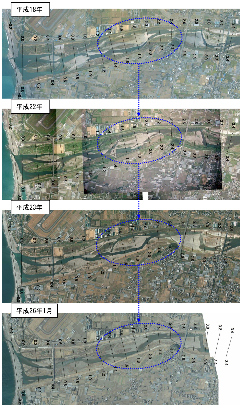
図 8-7(2) 流路の固定化の進行状況 (1.0k~3.0k 付近)
