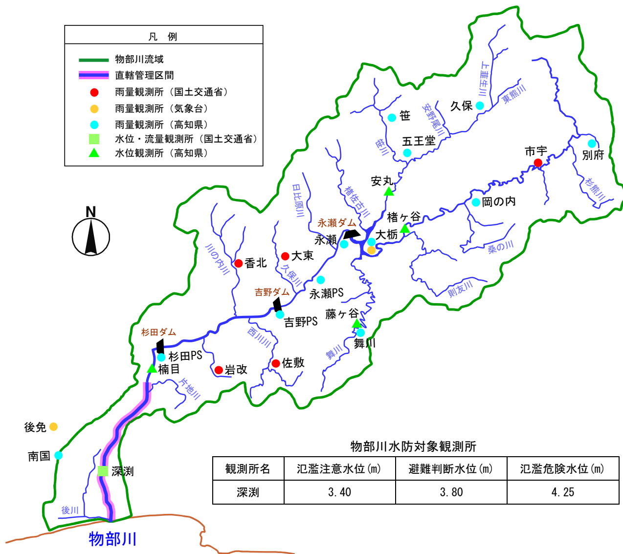
図 9-1 物部川流域水文観測所位置図
