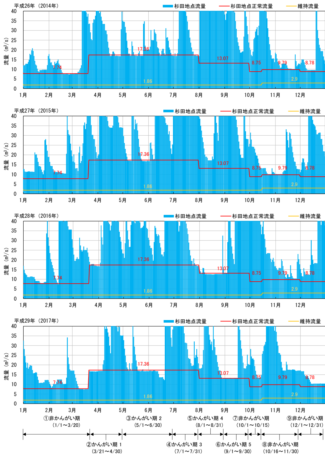
図 6-2(3) 日平均流量及び正常流量の比較図（杉田地点：平成26年～平成29年）
