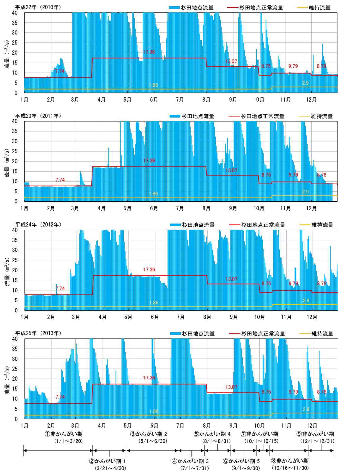
図 6-2(2) 日平均流量及び正常流量の比較図 (杉田地点：平成22年～平成25年)
