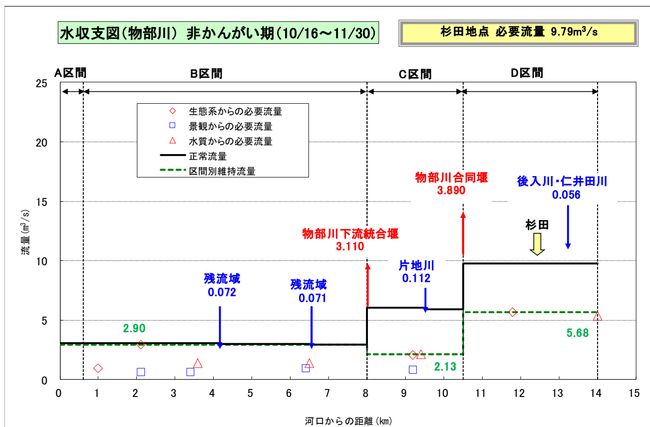
図 6-1(8) 物部川の水収支縦断図 (非かんがい期 : 10/16～11/30)
