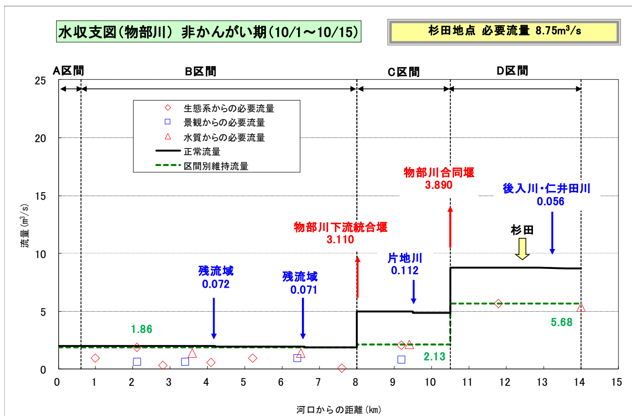
図 6-1(7) 物部川の水収支縦断図 (非かんがい期 : 10/1～10/15)
