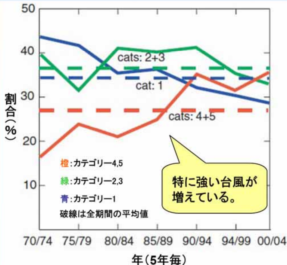
各カテゴリー※の熱帯低気圧の割合
