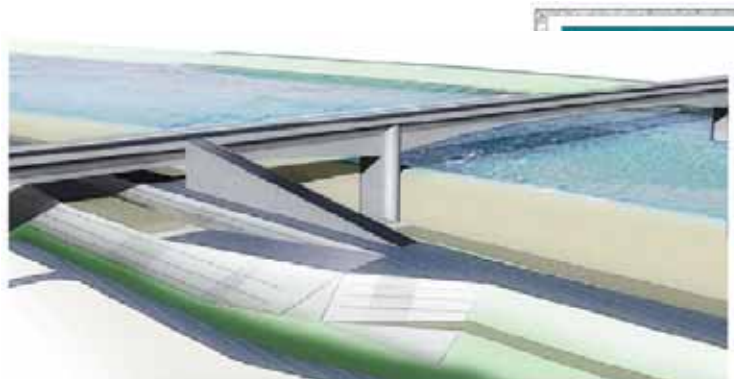
規格の高い道路と河川堤防の接続イメージ
