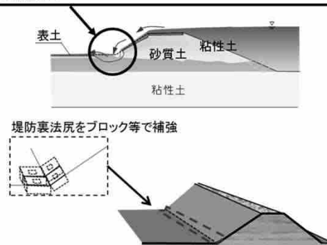
堤防裏法尻の補強
