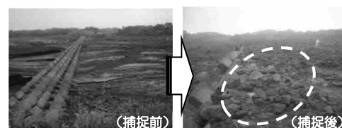
遊砂地工による流出土砂の捕捉状況（大沢川遊砂地）
