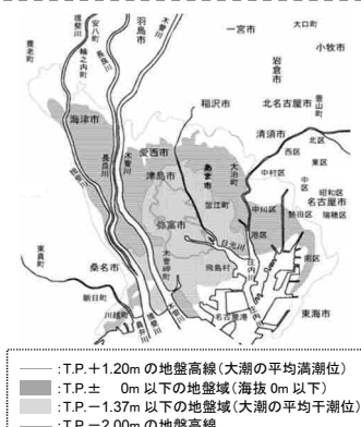
濃尾平野の海拔ゼロメートル地帯 （「平成28年における濃尾平野の地盤沈下の状況」より）
