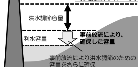
ダム流入予測高度化活用例
