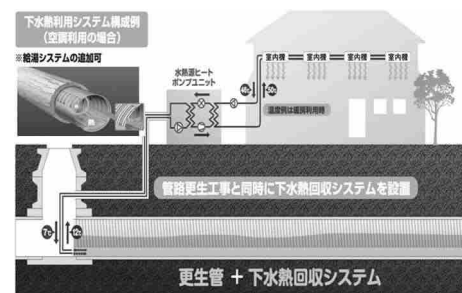
下水熱利用
