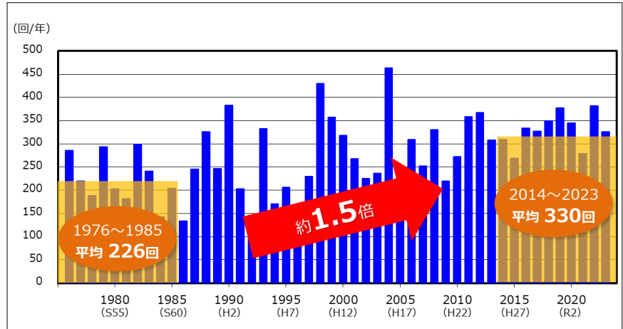
1 時間降水量50mm以上の年間発生回数 (アメダス1,300地点あたり) * 気象庁資料より作成
