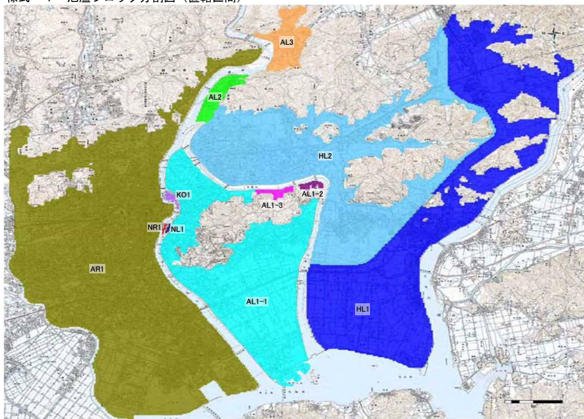
様式－１ 氾濫ブロック分割図（直轄区間）
