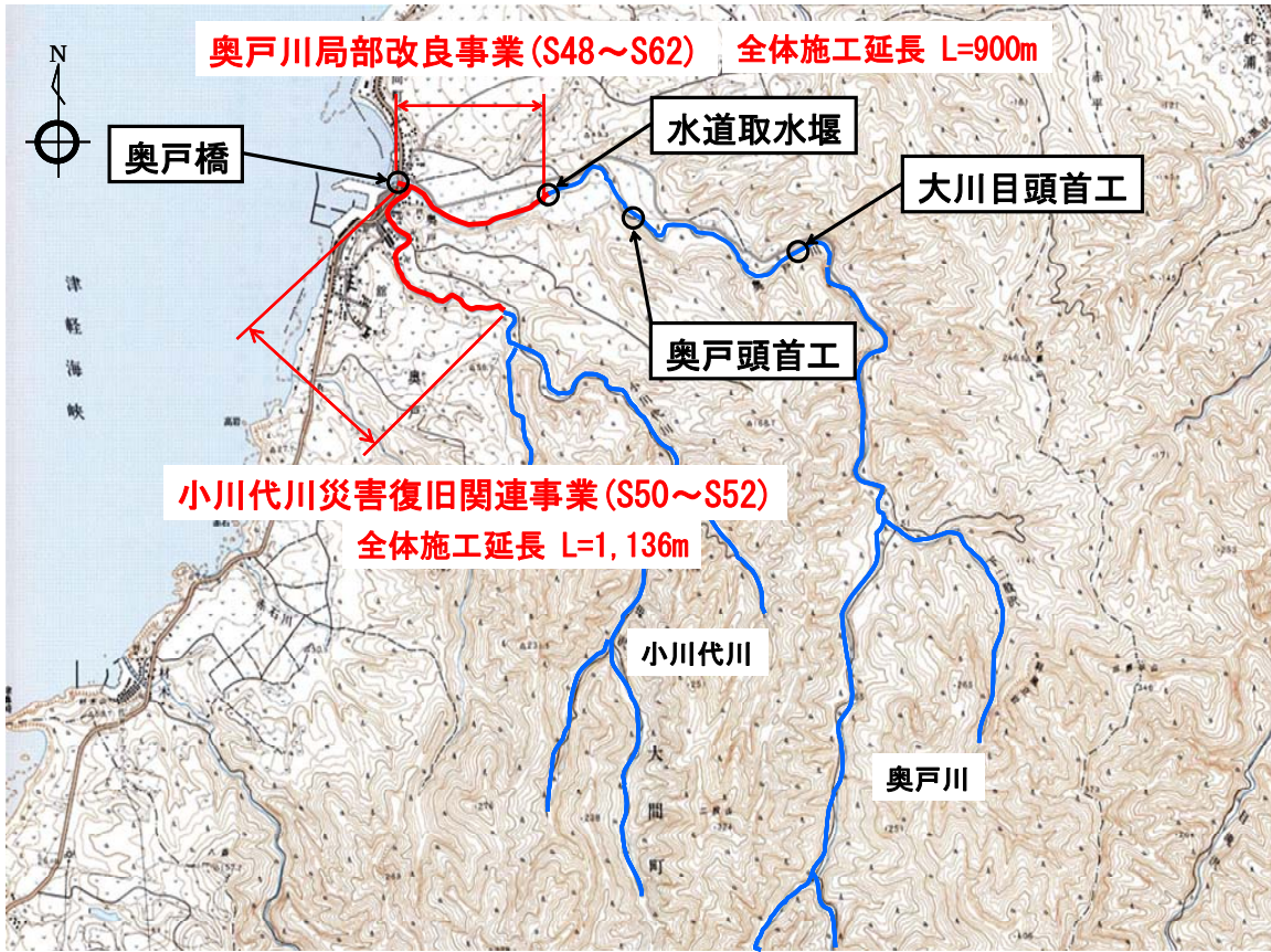
図－2.1 河川改修事業実施状況
