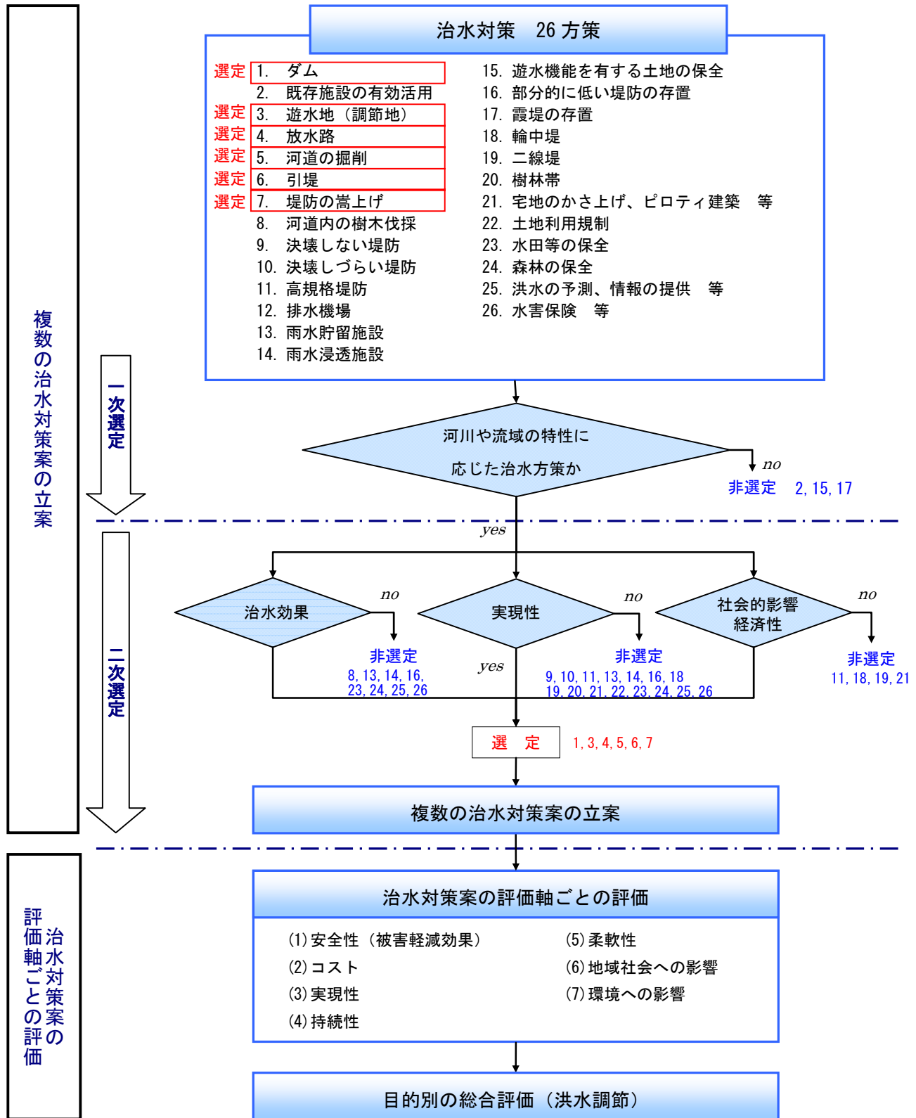
図－6.1 治水対策案検討フロー
