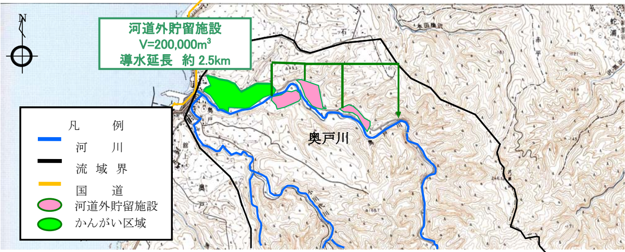
図－12.2 河道外貯留施設位置
