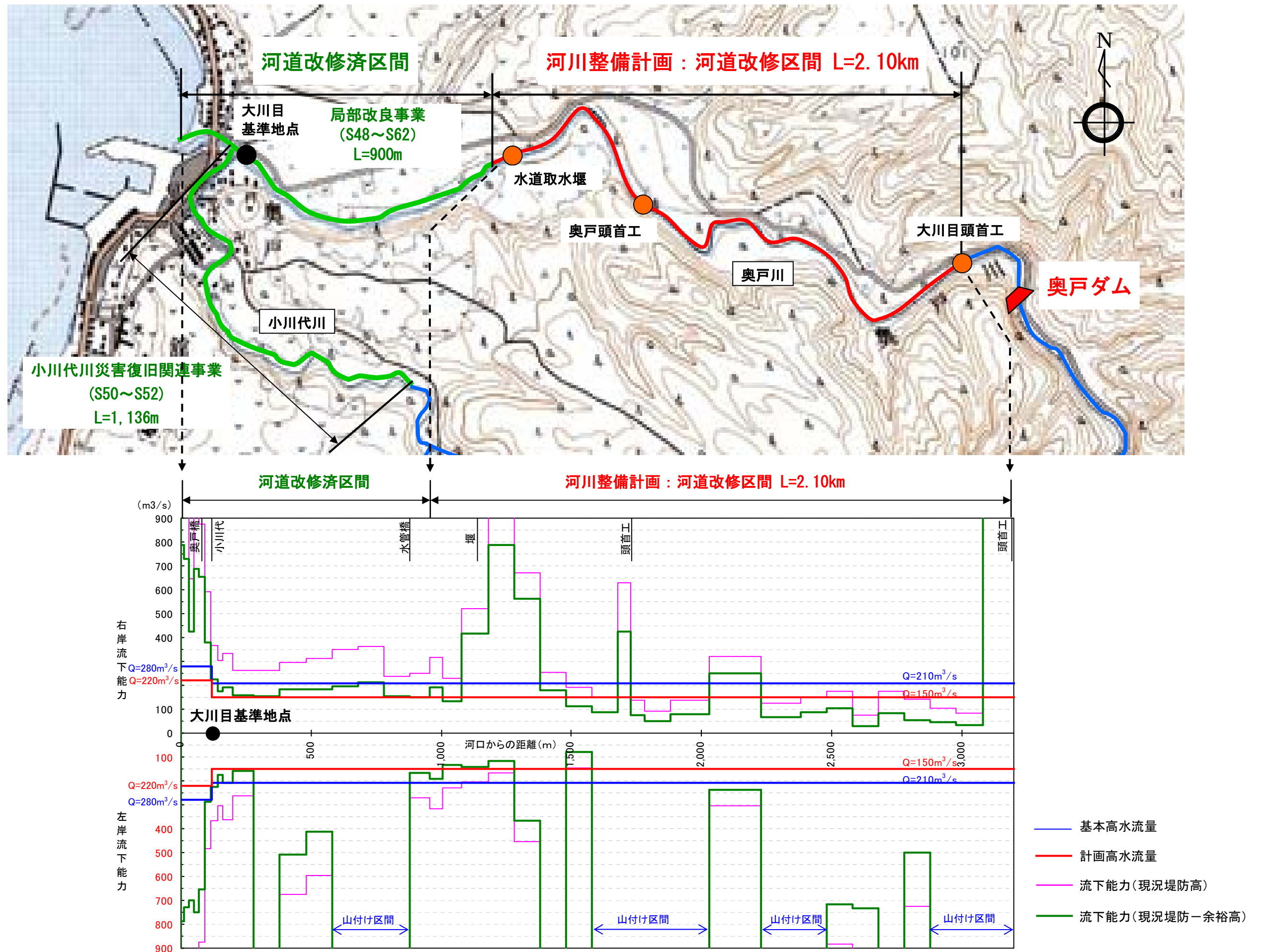
図-3.1 奥戸川流下能力図
