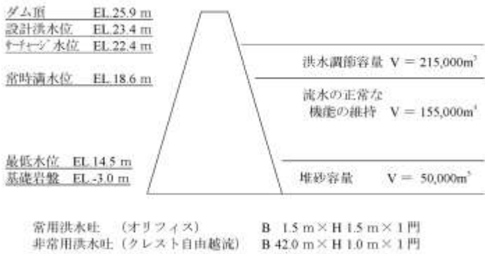
図ー2.1 貯水池容量配分図
