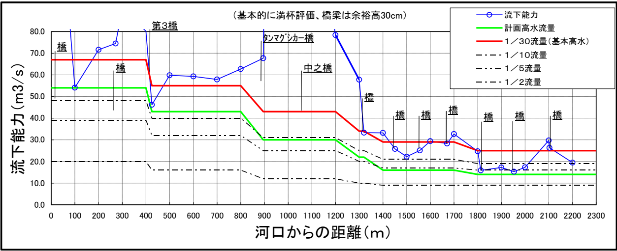
図－1.5 謝名堂川流下能力図
