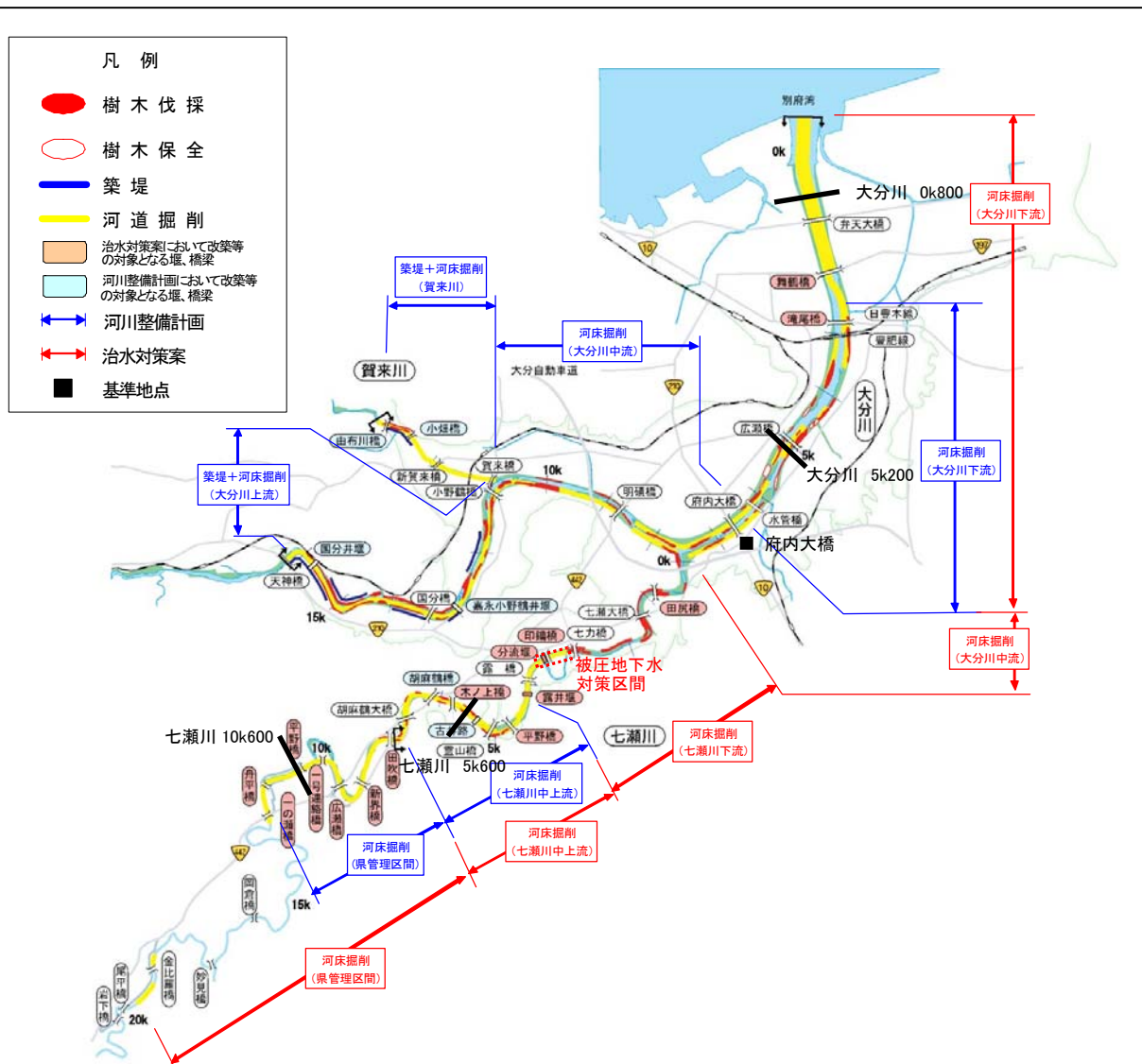
大分川河道掘削イメージ
