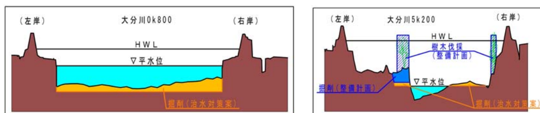
大分川河道掘削イメージ
