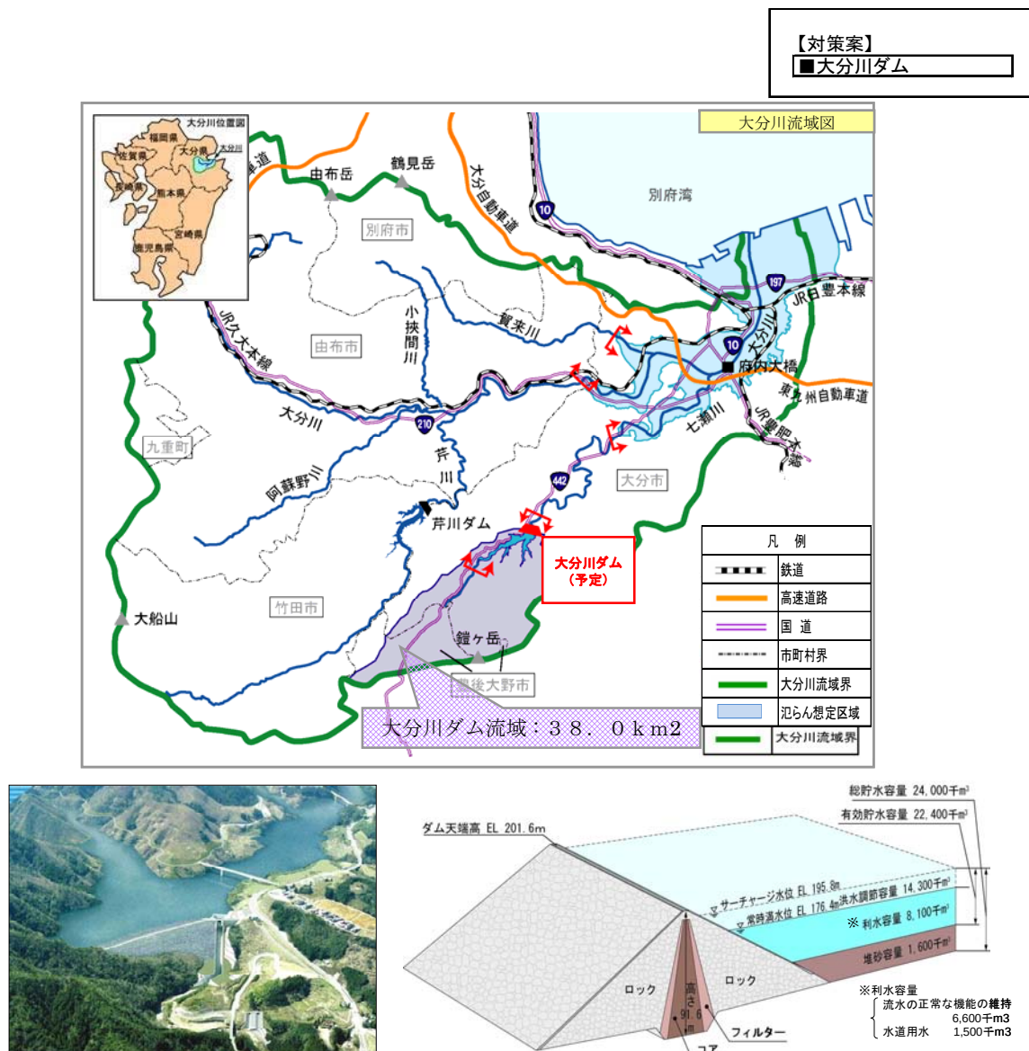
大分川ダム完成予定イメージ
