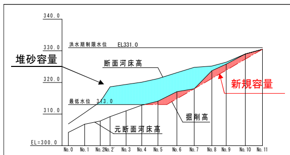
芹川ダム貯水池縦断面図（二又川）
