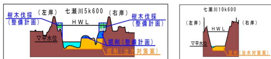
七瀬川河道掘削イメージ
