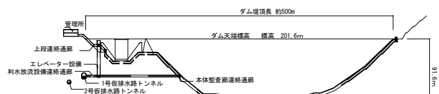
図 3-2-4 ダム軸縦断面図
