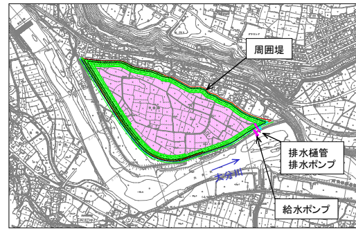
平瀬地区貯水池平面図
