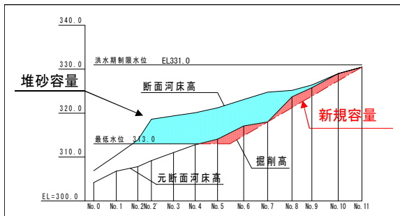
芹川ダム貯水池縦断面図（二又川）
