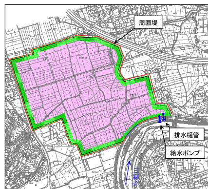
下宗方地区貯水池平面図
