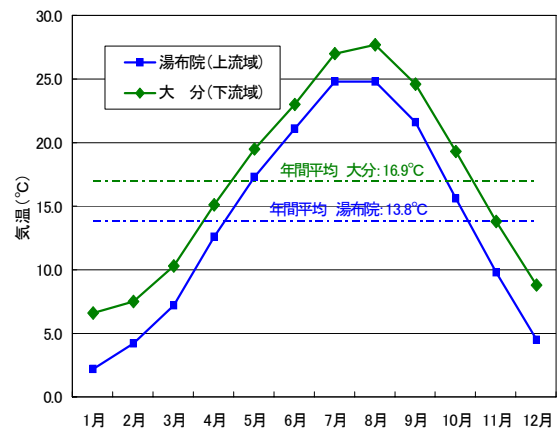
図 2-1-7 代表地点の月別平均気温
