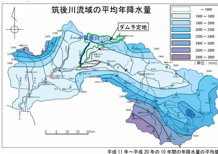
図 2.1-8 流域平均年降水量
