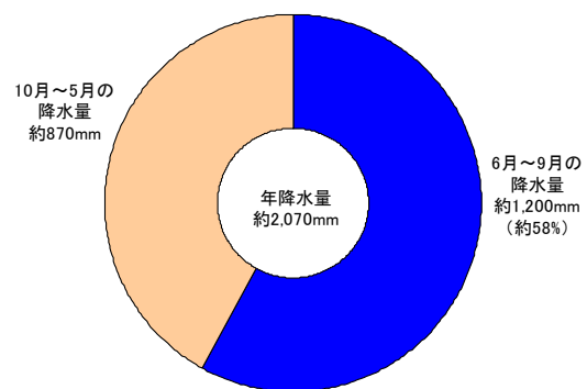
筑後川流域年降水量 (平成11年～平成20年の平均)
