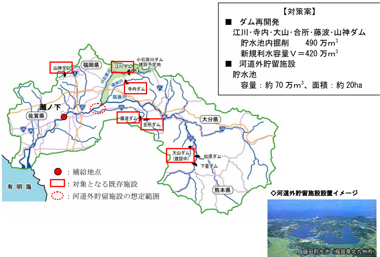
◇合所ダム貯水池内掘削 概略位置図
