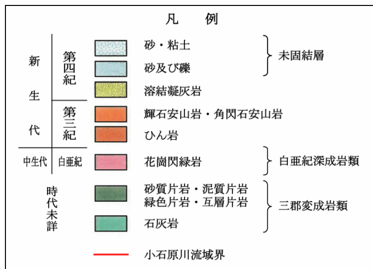
図 2.1-6 小石原川流域の地質状況
