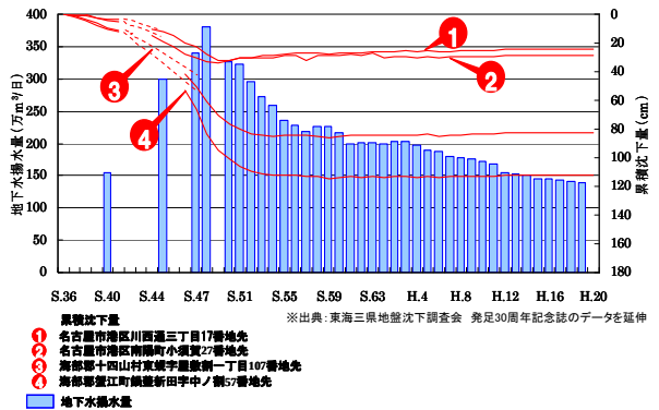
濃尾平野南部臨海域における一等水準点の地盤沈下と地下水揚水量の経年変動
