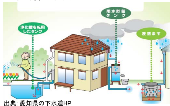
図 4.4.15 雨水・中水利用の概要
