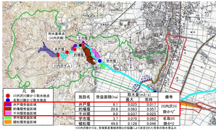
図一 2.2.4 川内沢川の水利用
