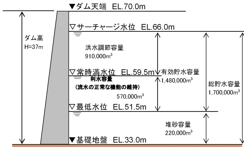
図一 3.1.3 川内沢ダム貯水池容量配分図
