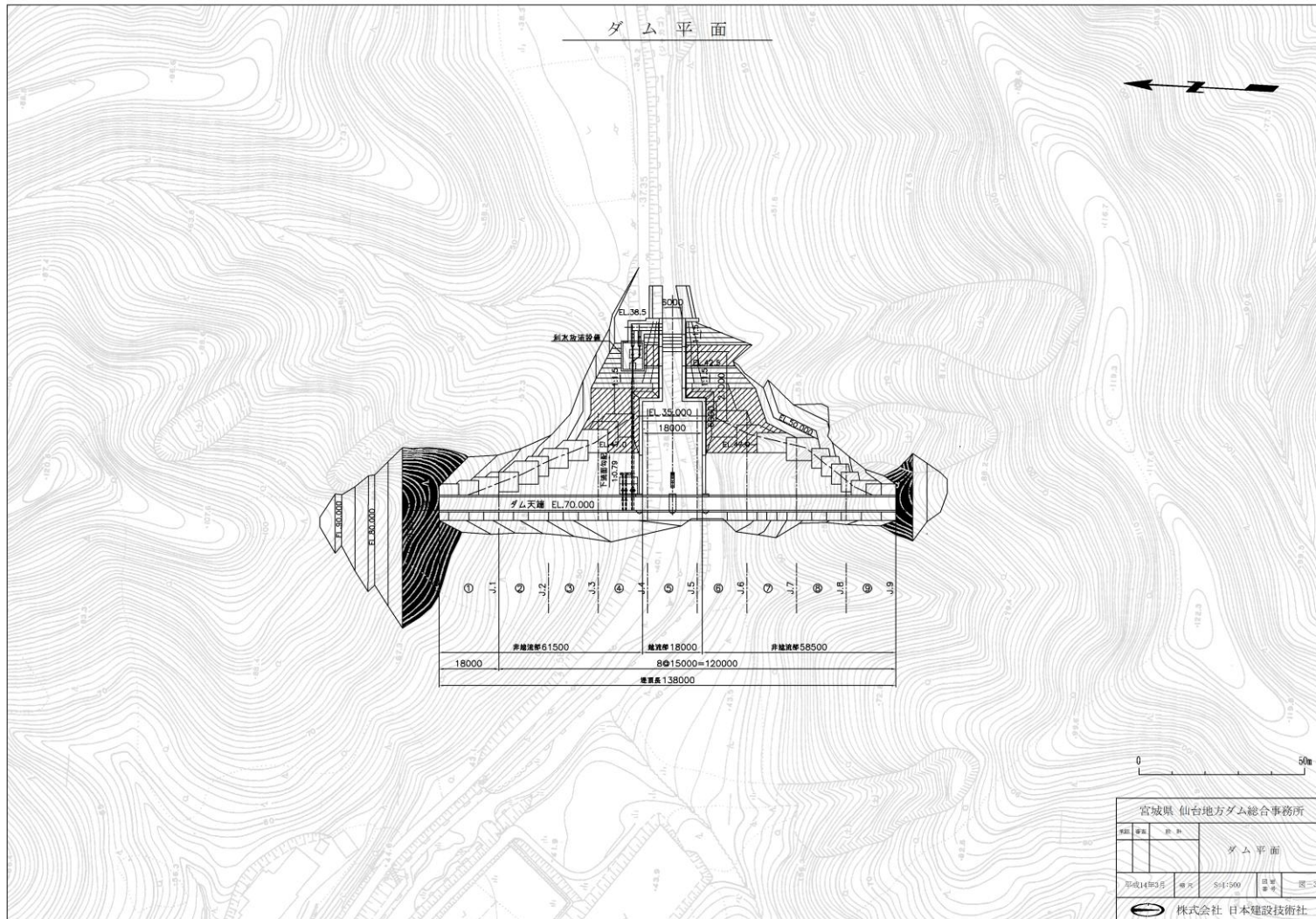
図- 3.1.4 ダム平面図 (現計画)
