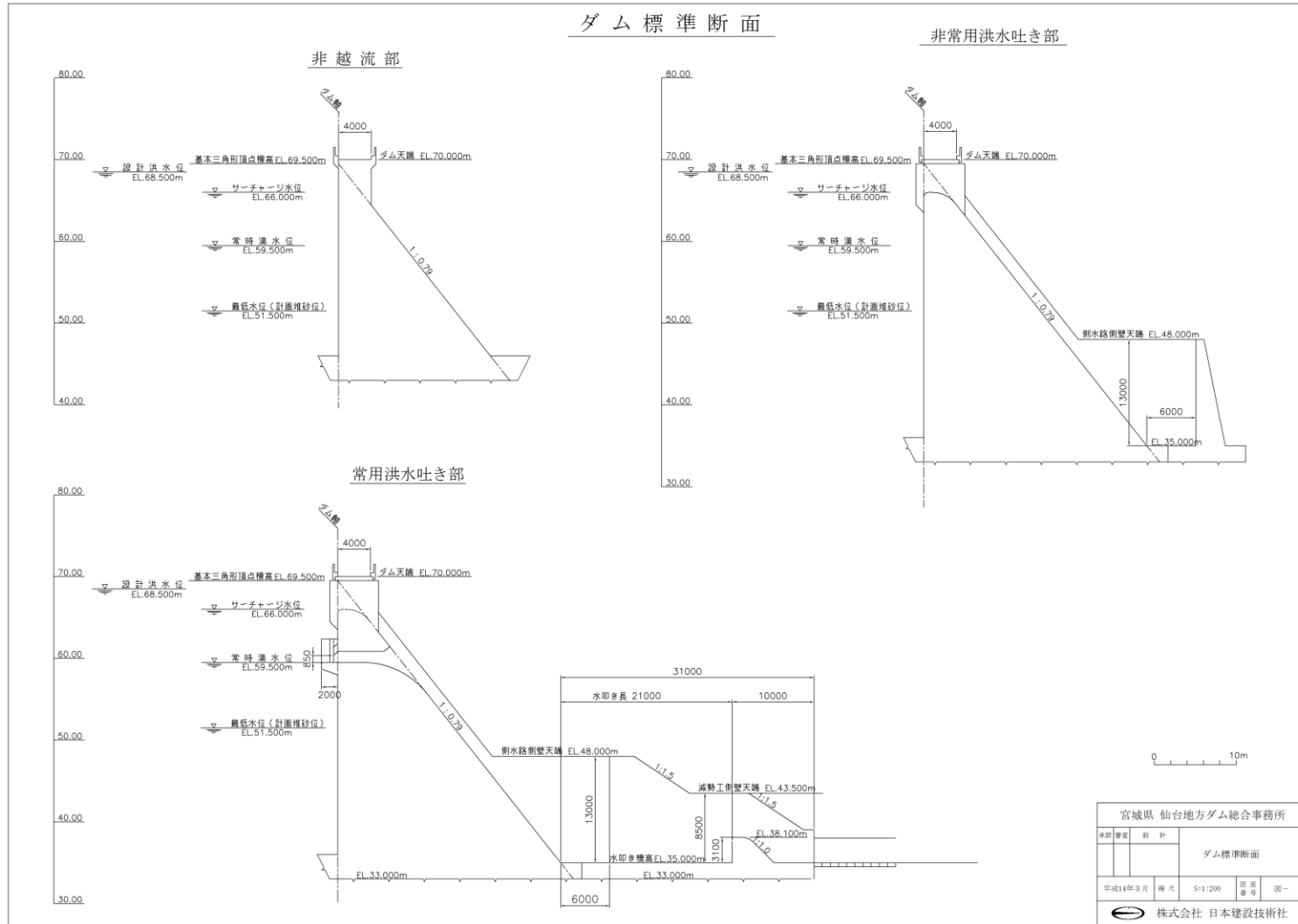
図一 3.1.7 ダム標準断面図 (現計画)
