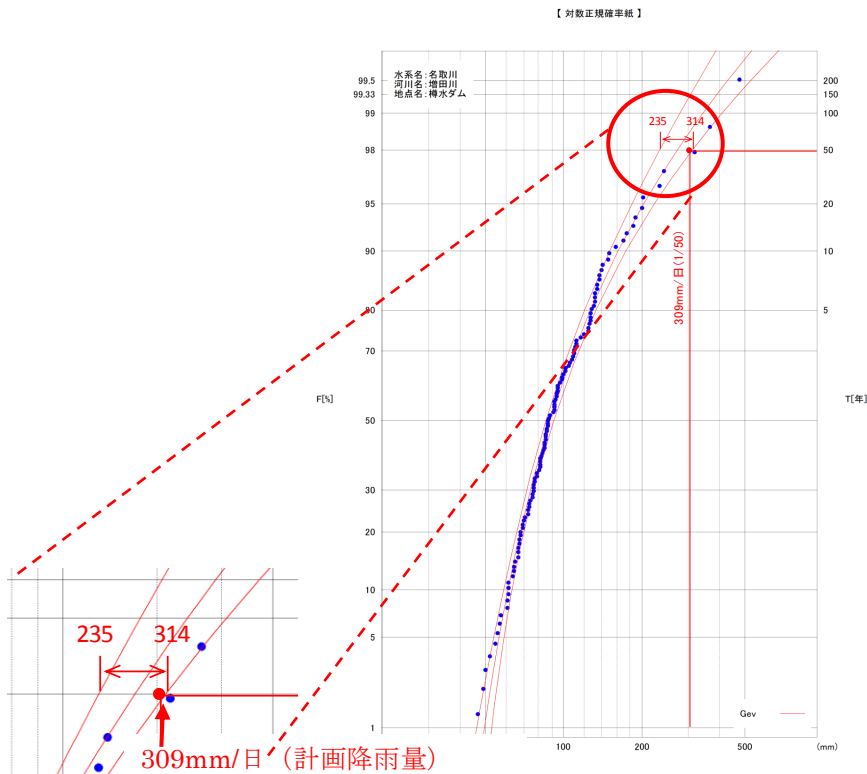
図－ 4.1.2 Gev（一般化極値分布）法の超過確率図
