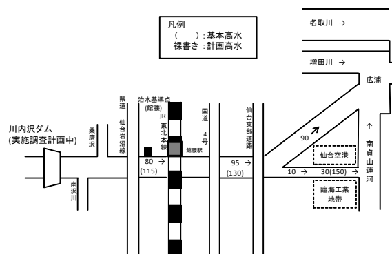
図ー 4.1.3 基本高水ピーク流量配分図
