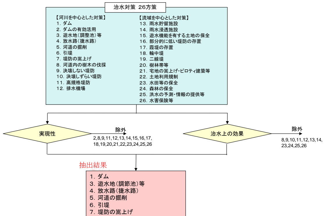
図一 4.2.2 複数の治水対策案の抽出
