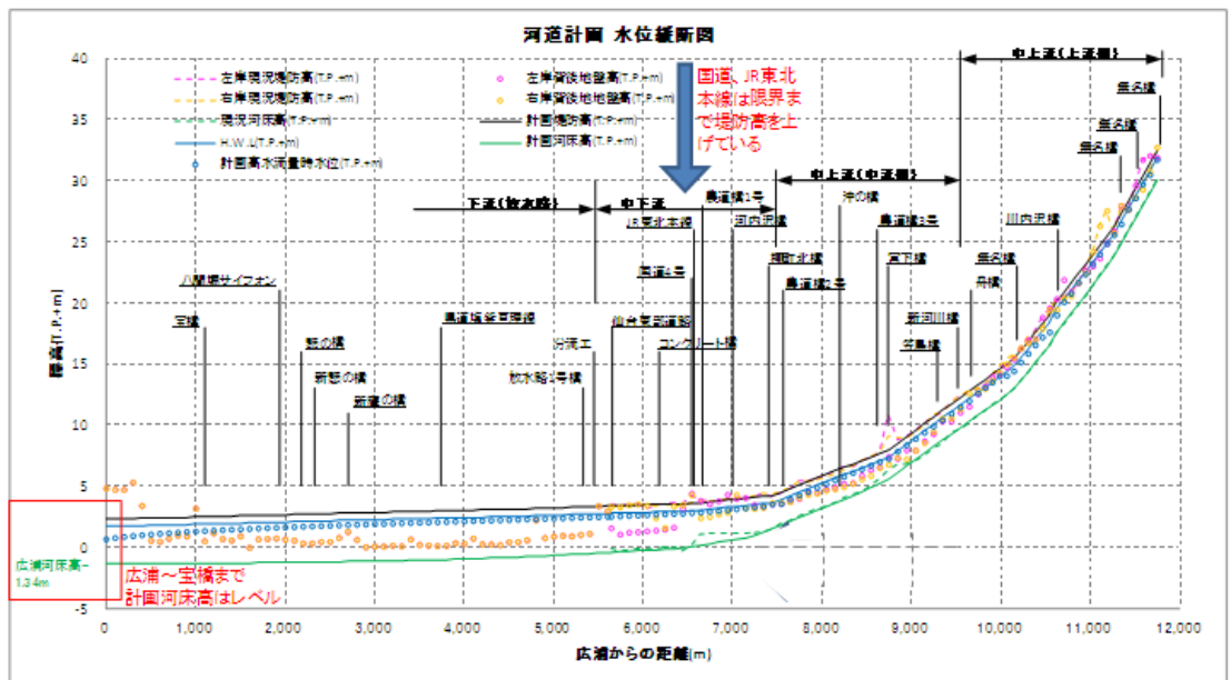
図-4.2.30 現在進めている河道計画の縦断面図
