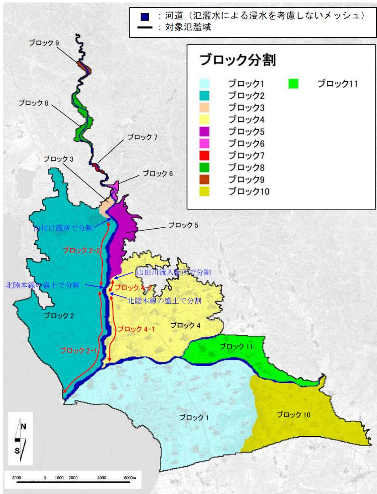
様式－１ 氾濫ブロック図（姉川・高時川）
