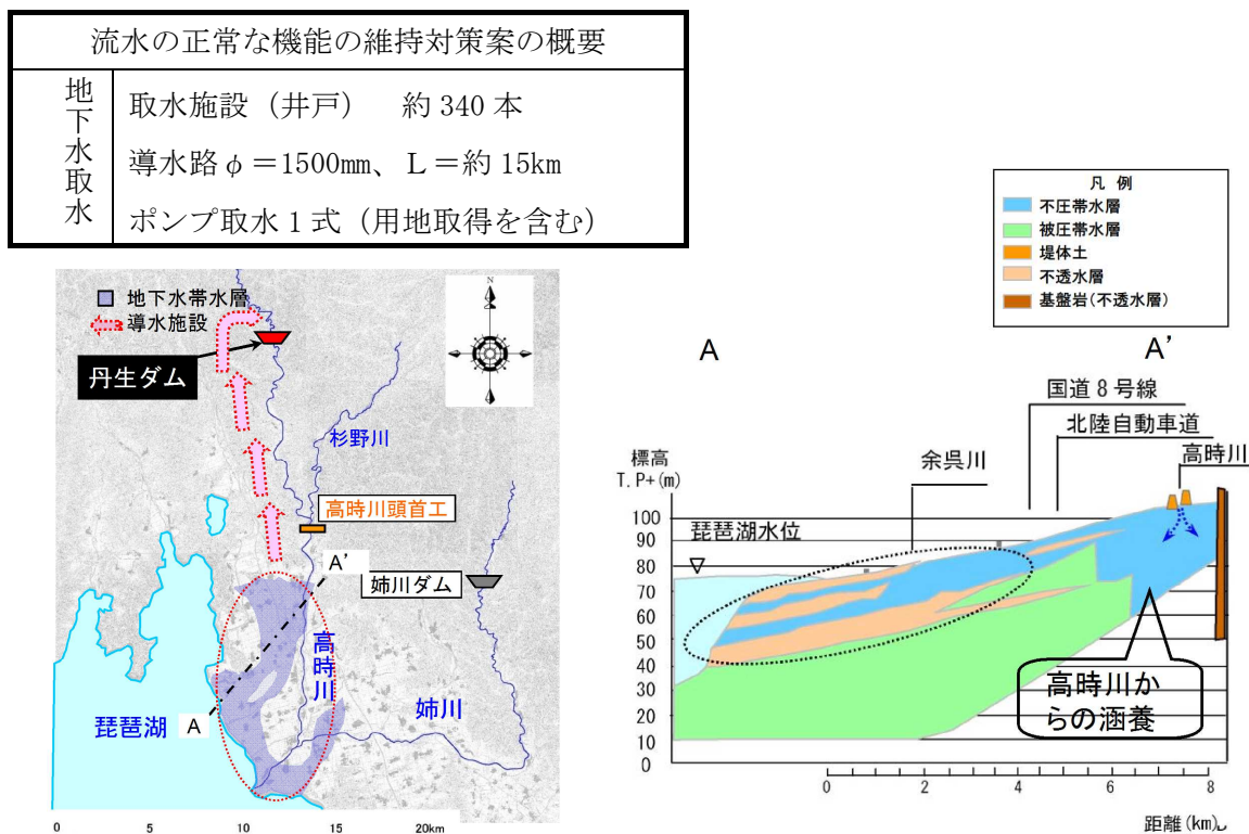
図 4.4.20 地下水取水による導水施設整備イメージ
