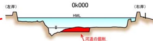
河道掘削のイメージ
