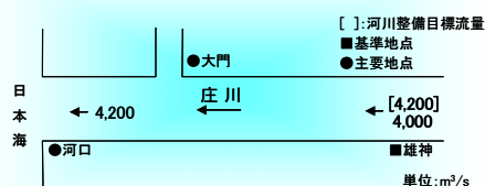
主要地点における河道配分流量
