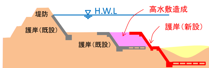
急流河川対策のイメージ
