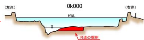
河道掘削のイメージ
