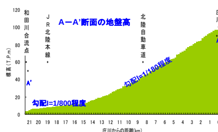
放水路縦断勾配
