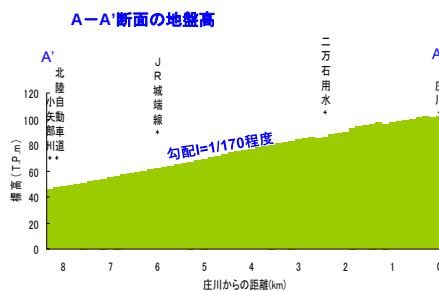
放水路縦断面勾配
