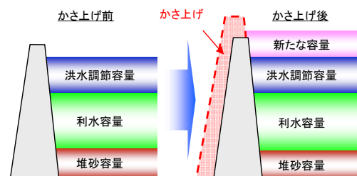
境川ダムかさ上げのイメージ
