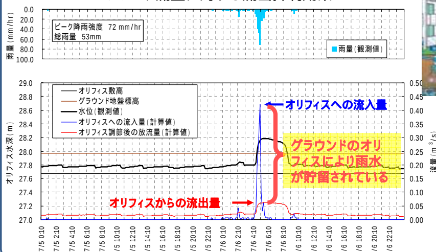
高校のグラウンドを利用した雨水貯留浸透施設（オリフィス設置）のピーク流量に対する流出抑制効果
