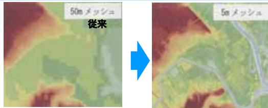
従来の地形データ：標高誤差1m程度 新たに作成する地形データ：標高誤差30cm程度 出典：「図解航空レーザ測量」(財)日本測量調査技術協会
