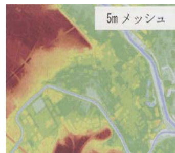
新たに作成する地形データ：標高誤差30cm程度 出典：『図解 航空レーザ計測』(財)日本測量調査技術協会
