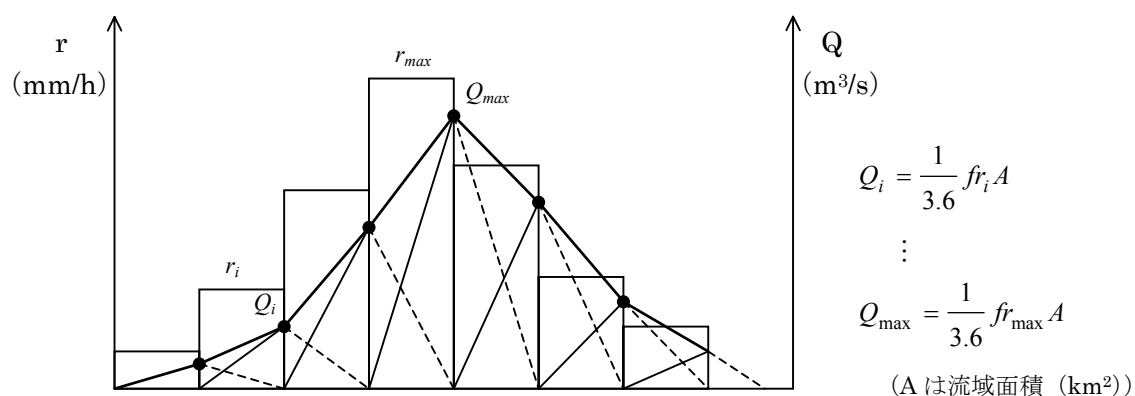
図-3 合成合理式による流出計算
