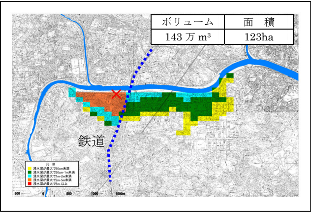
2池モデル計算結果
