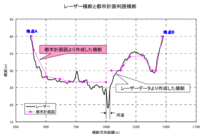
図-5 レーザ測量データ（メッシュデータ）による流域横断の例
