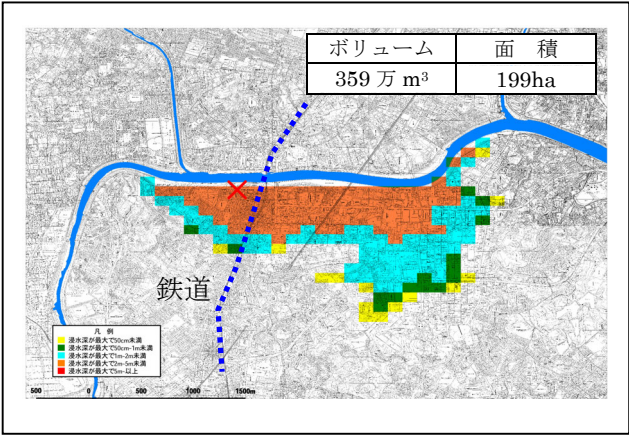
1池モデル計算結果
