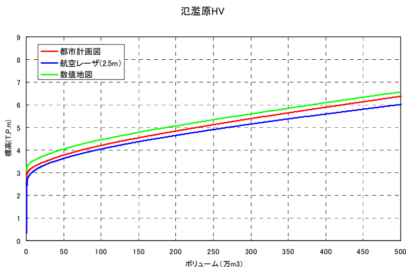
図-8 航空レーザ測量、都市計画図、数値地図による H・V の例
