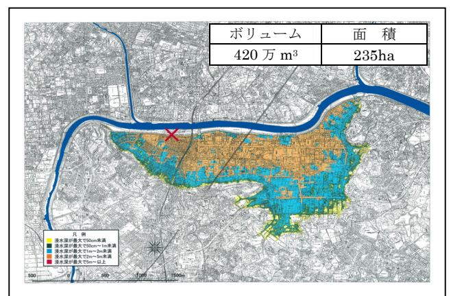
図-10 池モデルによる浸水区域の例
