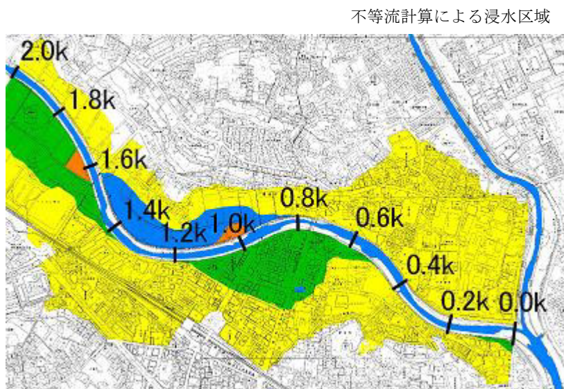
図-7 不等流モデルによる浸水区域
