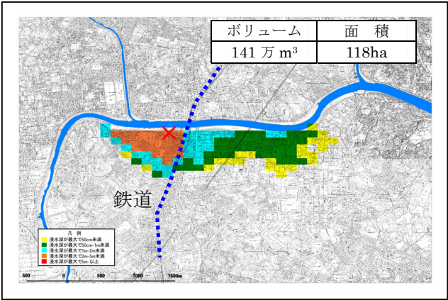
2次元不定流計算結果
