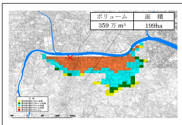
図-10 池モデルによる浸水区域の例
