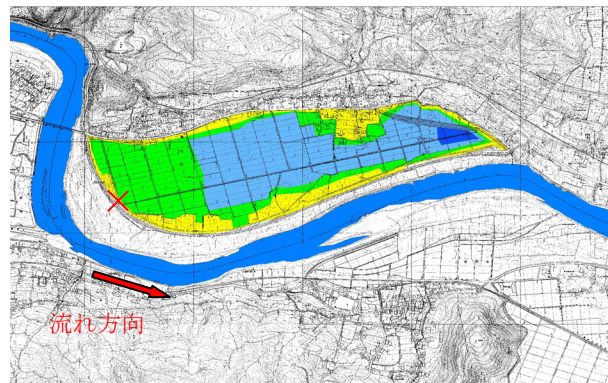
貯留型はん濫
