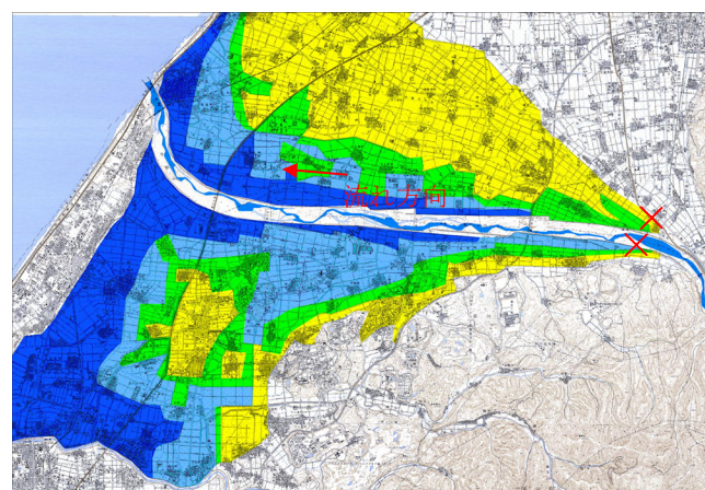
拡散型はん濫
