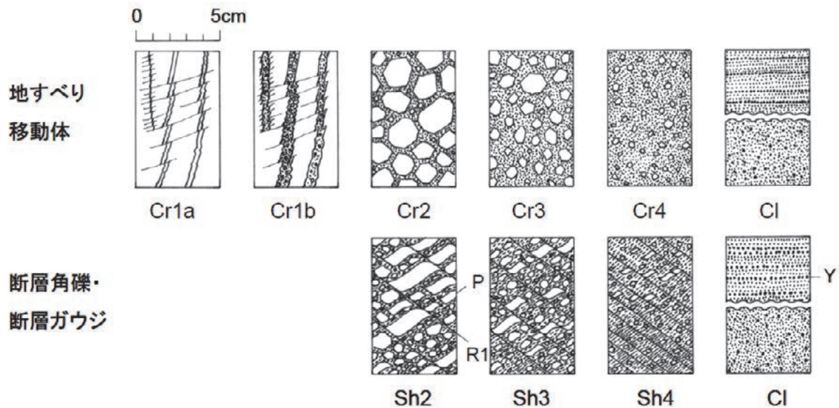
図15-4-4 地すべり移動体及び断層岩類の破碎度区分の例（脇坂・上妻・綿谷・豊口, 2012）
