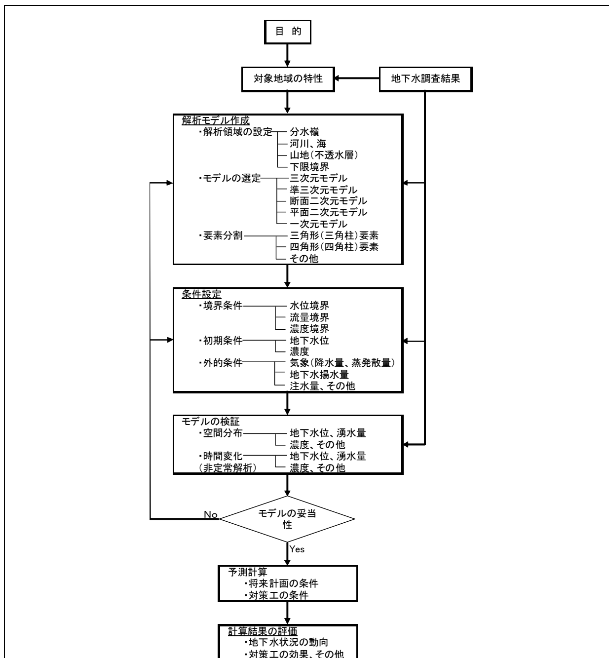
図3-3-2 地下水流動解析の流れ (「地下水調査及び観測指針(案)」に加筆)
