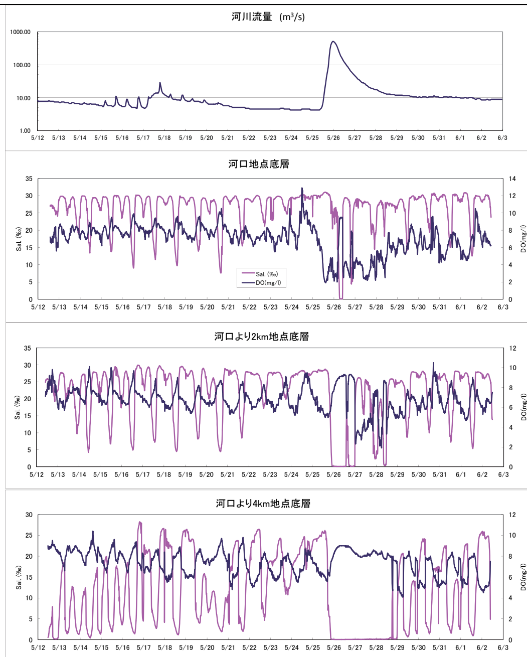
図14-2-7 汽水域における水質の連続観測結果の例
