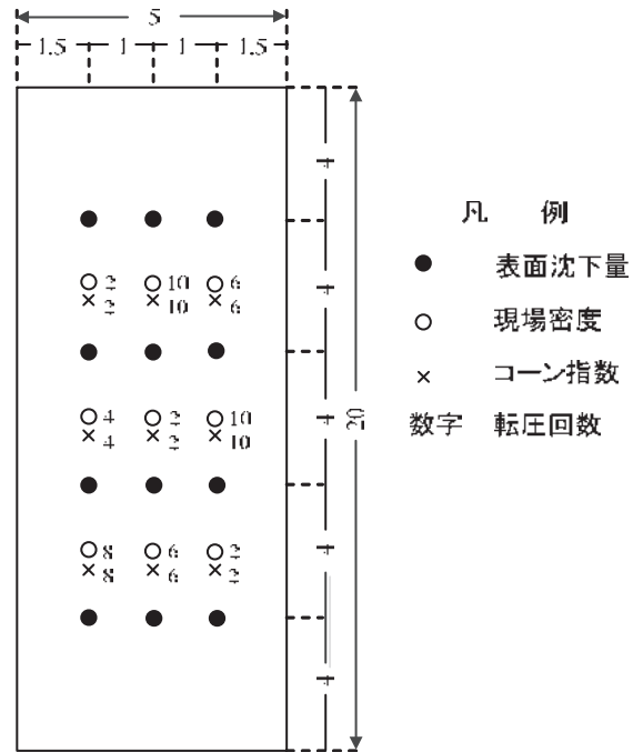
図15-2-2 試験施工の測定項目と測点位配置の一例
