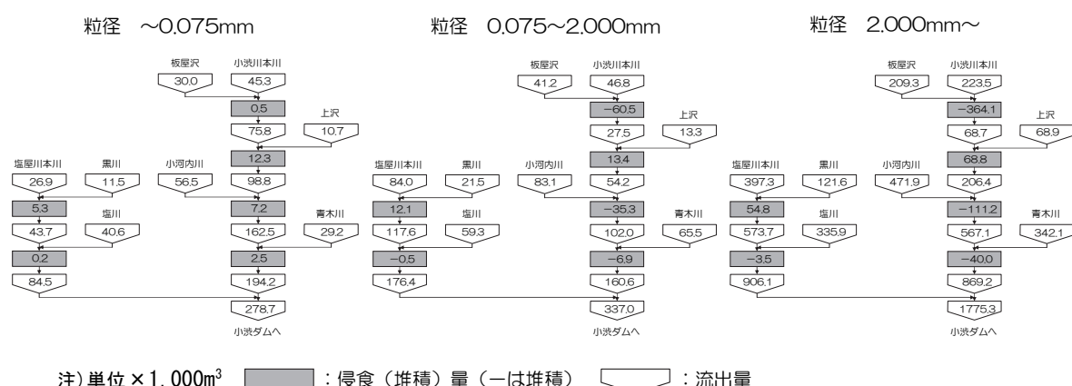
図16-2-2 山地部についての粒径別土砂収支図の作成例（小渋川流砂系：地形測量による1982年8月・9月出水前後の土砂収支）
