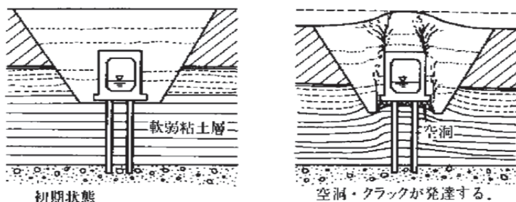
図15-3-1 支持杭基礎の場合の抜け上がりと空洞形成
