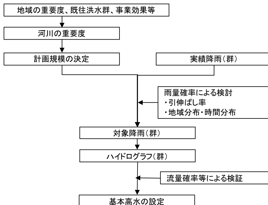
図2-2 基本高水の設定
