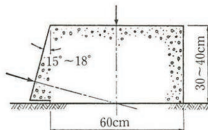
図2-6-2 ブロックせん断試験
