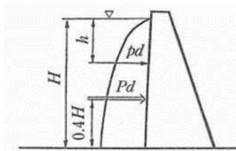
図2-3-3 Westergaard の式
