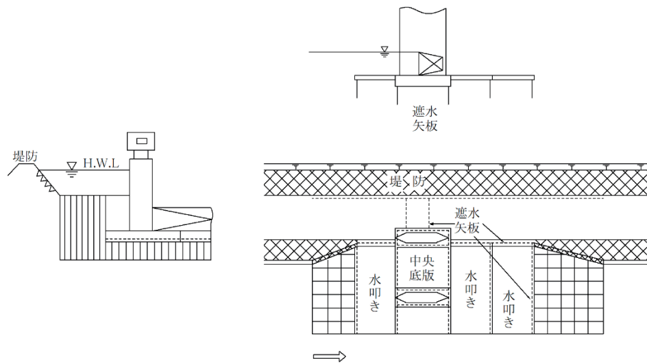
図7-28 遮水工（鋼矢板構造）
