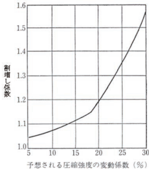
図2-4-2 一般の場合の割増し係数
