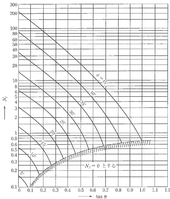
図6-11 支持力係数 N_\gamma を求めるグラフ
