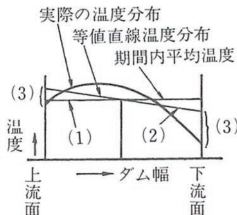
図2-3-6 ダム断面内温度分布
