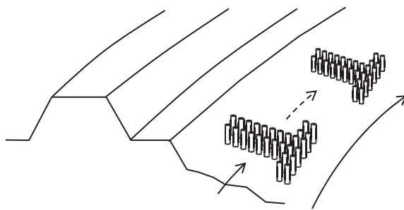
透過水制の例（杭出）
