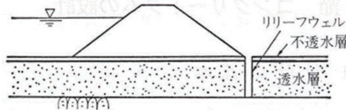
図2-6-19 リリーフウェルの配置
