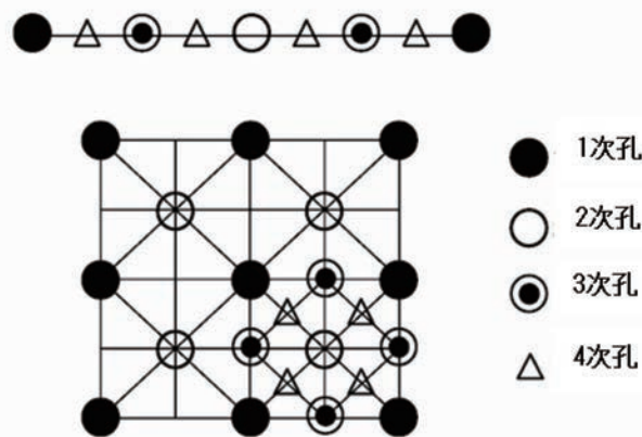
図2-6-11 中央内挿法の説明（平面配置）
