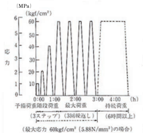
図2-6-4 荷重載荷方法の例
