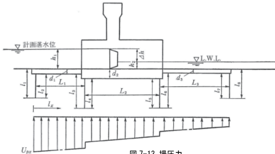
図 7-13 揚圧力
