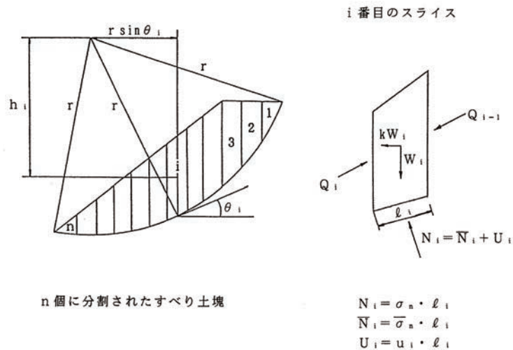
図2-5-17 スライス法
