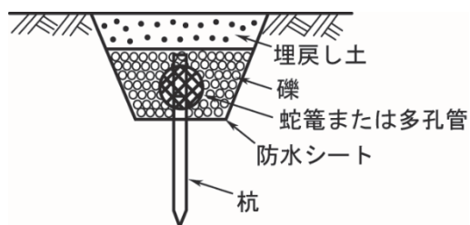
図 4-3-2 蛇籠暗渠
