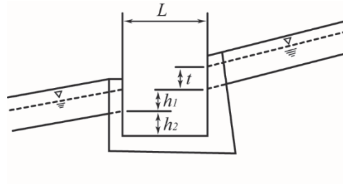
図 4-2-3 集水枡側面図
