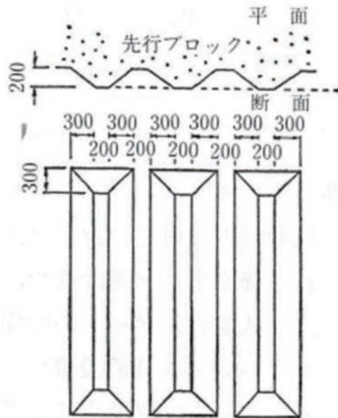
図2-4-13横継ぎ目のせん断キーの標準図
