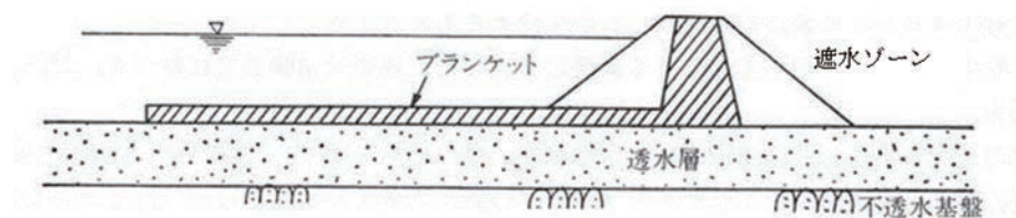
図2-6-17 ブランケットによる砂礫基礎の遮水
