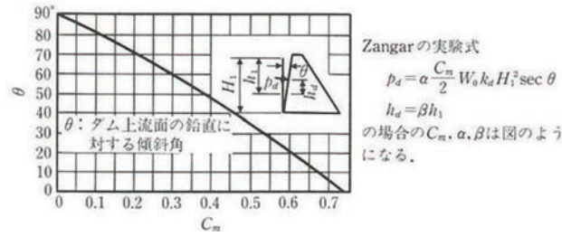
図2-3-4 Zangar の式の \theta — C_m 曲線
