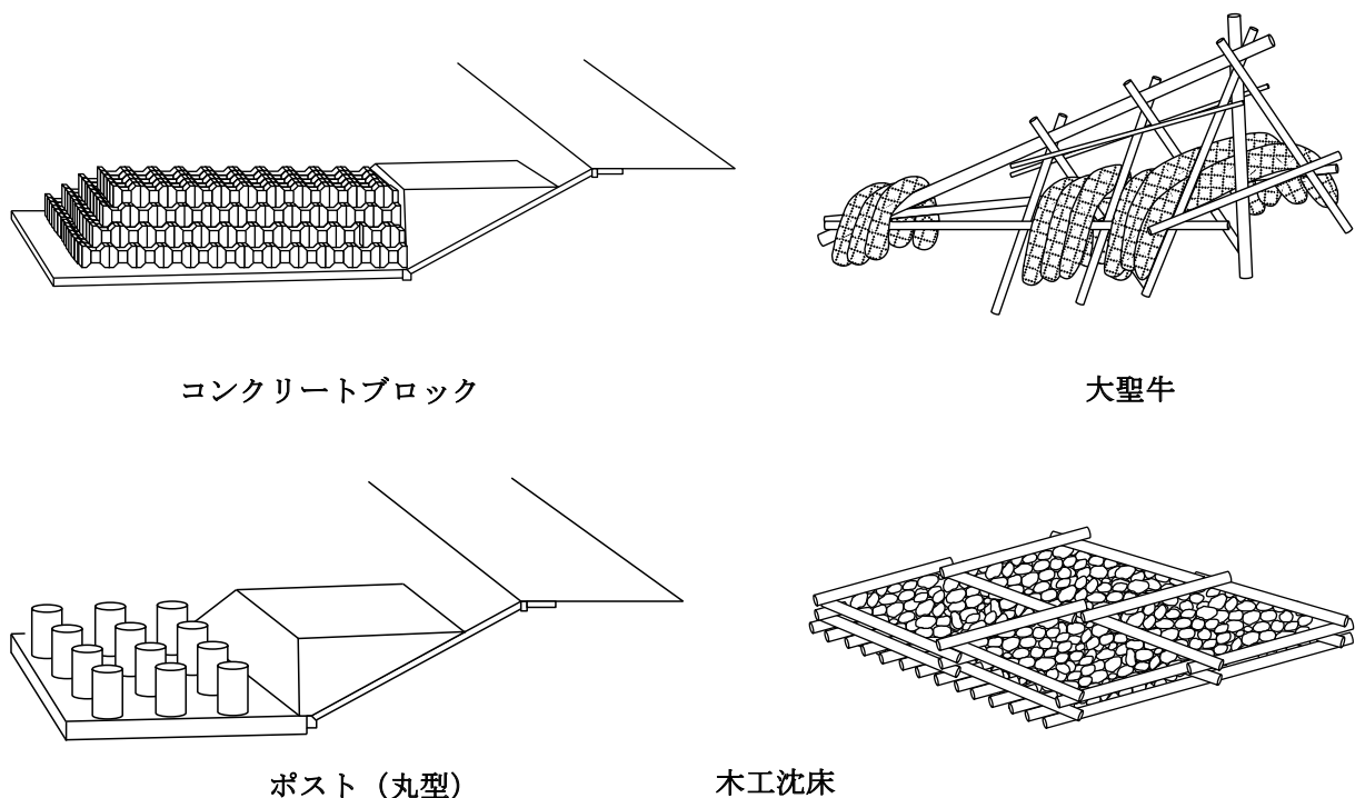
図 1-4-15 水制の工種の例
