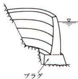
図2-4-11 プラグ
