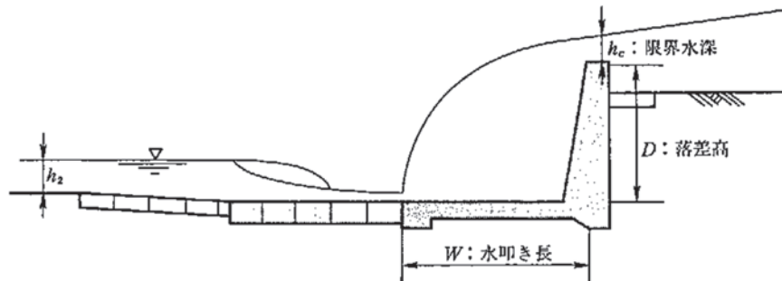
図6-16 完全越流時の水面形状
