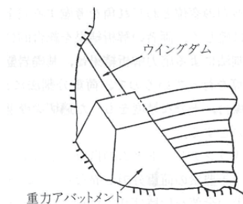
図2-4-10 重力式アバットメント及びウイングダム
