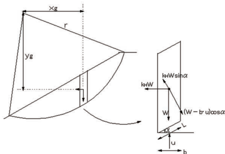
図2-12-15 滑動変位計算モデル
