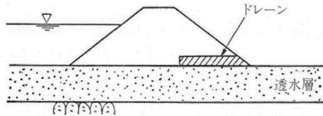
図2-6-18 ドレーンの配置
