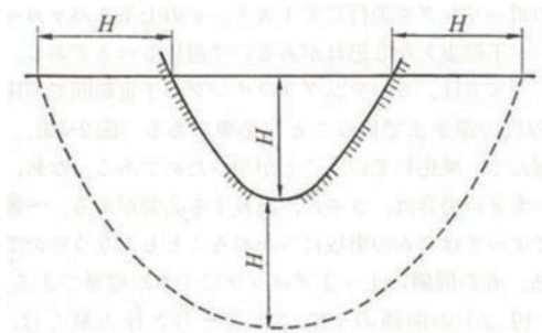
図2-6-6 ルジオンテストの範囲
