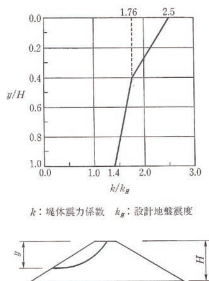
図2-5-16 堤体震力係数
