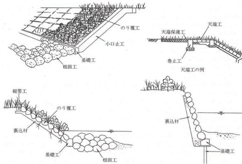
図 1-4-5 護岸の構成
