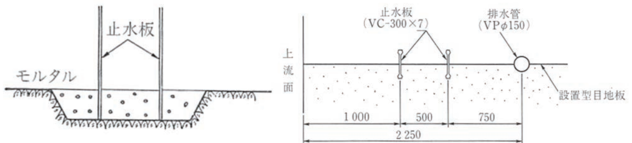
図2-4-15 止水装置の構造図
