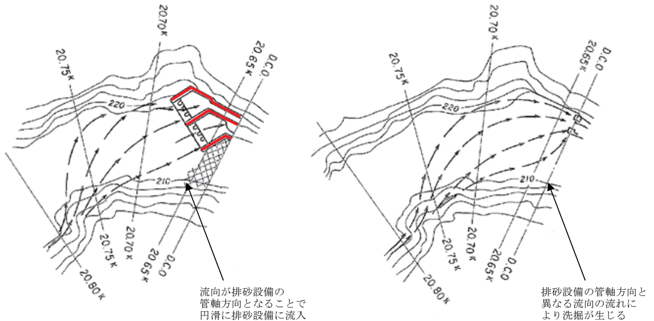
図2-7-3 流入部構造物有無のダム近傍の流れの比較
