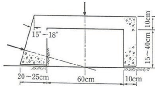
図2-6-3 ロックせん断試験
