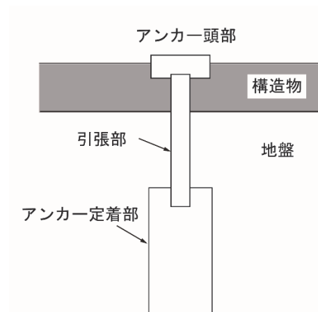
図 4-7-1 グラウンドアンカー工の構成要素
