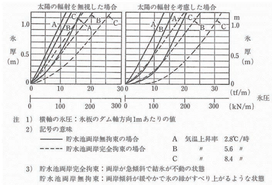
図2-3-1 氷厚と氷圧との関係
