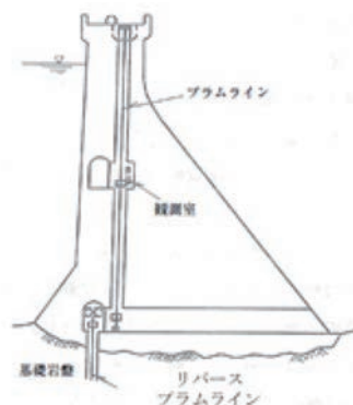
図2-4-17 重力式コンクリートダムに設置されたプライムライン
