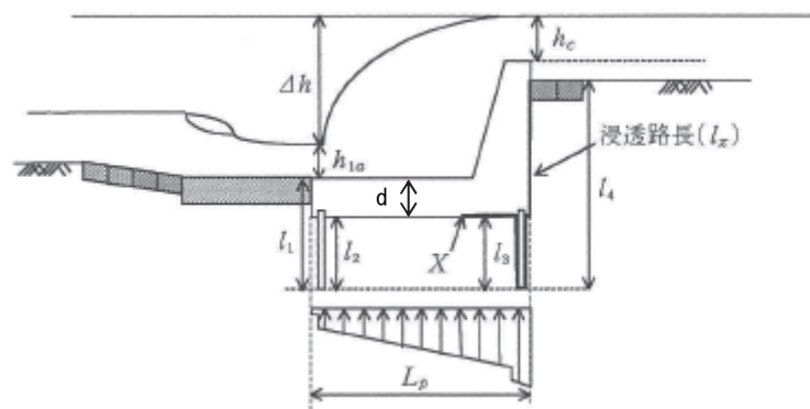
図6-15 床止め作用する揚圧力
