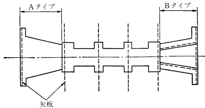
図8-17 遮水工
