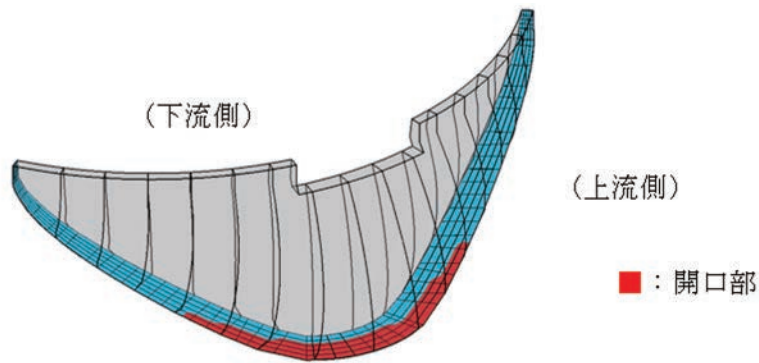
図2-12-13 アーチ式コンクリートダムの周辺継目の開口範囲の例
