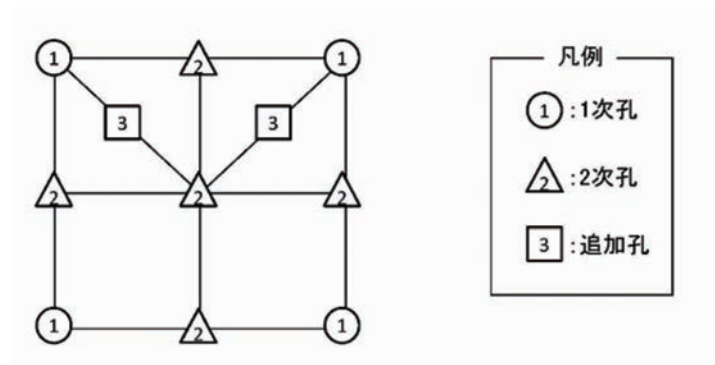
図2-6-12 孔の平面配置
