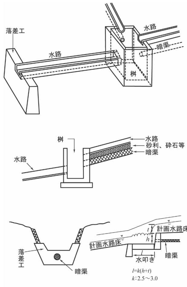
図 4-2-4 集水樹と落差工の例
