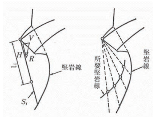
図2-2-7 所要堅岩線
