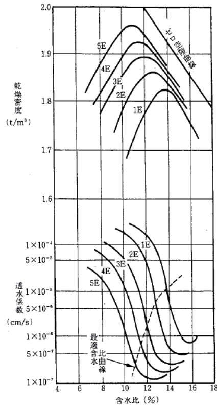
図2-5-8 締固めエネルギーを変えた場合の乾燥密度、透水係数－含水比曲線
