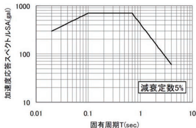
図2-12-8 下限加速度応答ベクトル図 水平地震動
