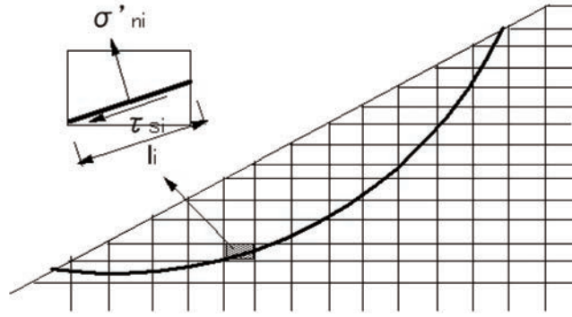
図2-12-16 すべり線上の要素の応力
