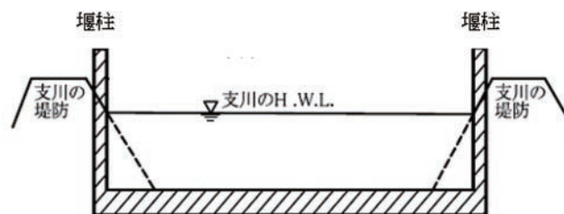
図9-2 水門の断面説明図（流下断面が1.3倍以内の場合）
