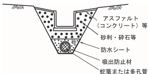
図 4-3-3 明暗渠工横断図
