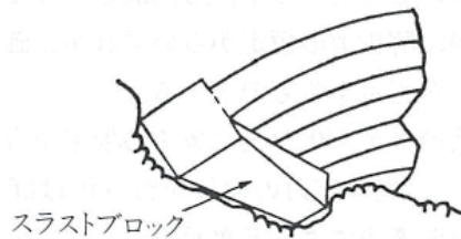
図2-4-9 スラストブロック
