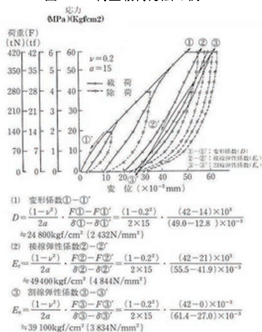
図2-6-5 荷重変位曲線の例
