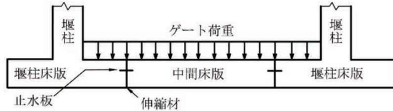
図9-9 本体の形式がT形の場合の床版
