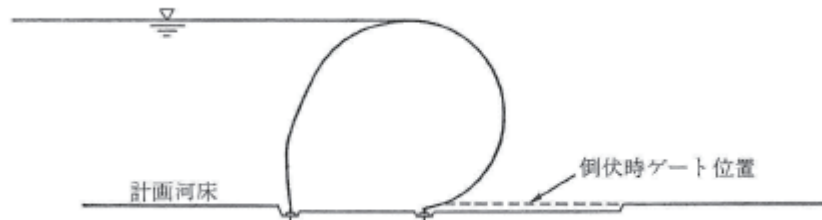
図7-15 ゴム引布製伏式ゲート
