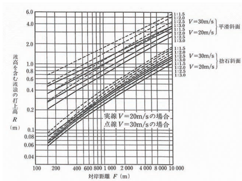
図2-2-4 S. M. B 法における Wilson の改良式と Saville の方法とを組み合わせる求めた打上げ高（波高を含む）
