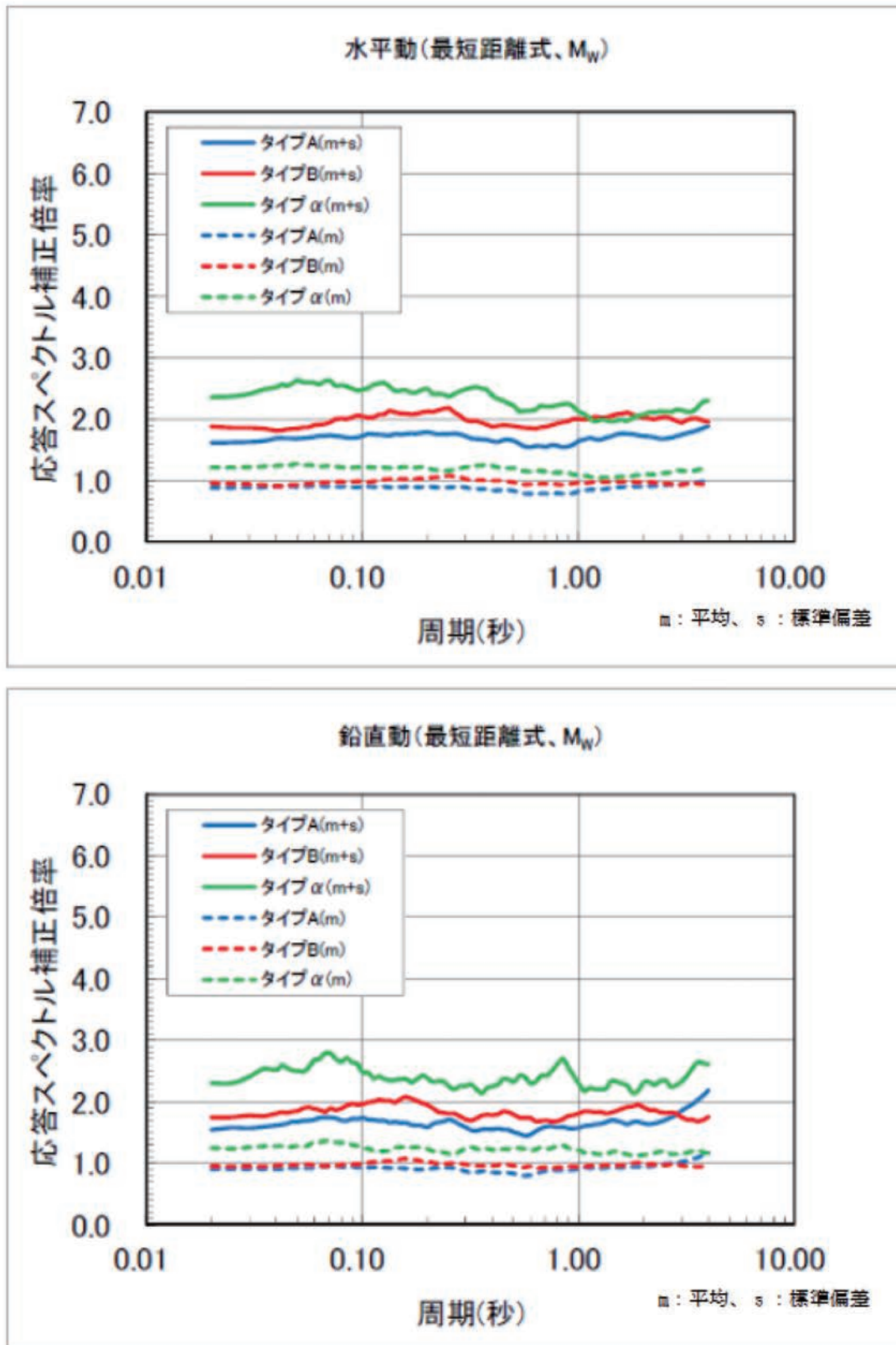
図2-12-6 最短距離式 地震タイプ別補正倍率
