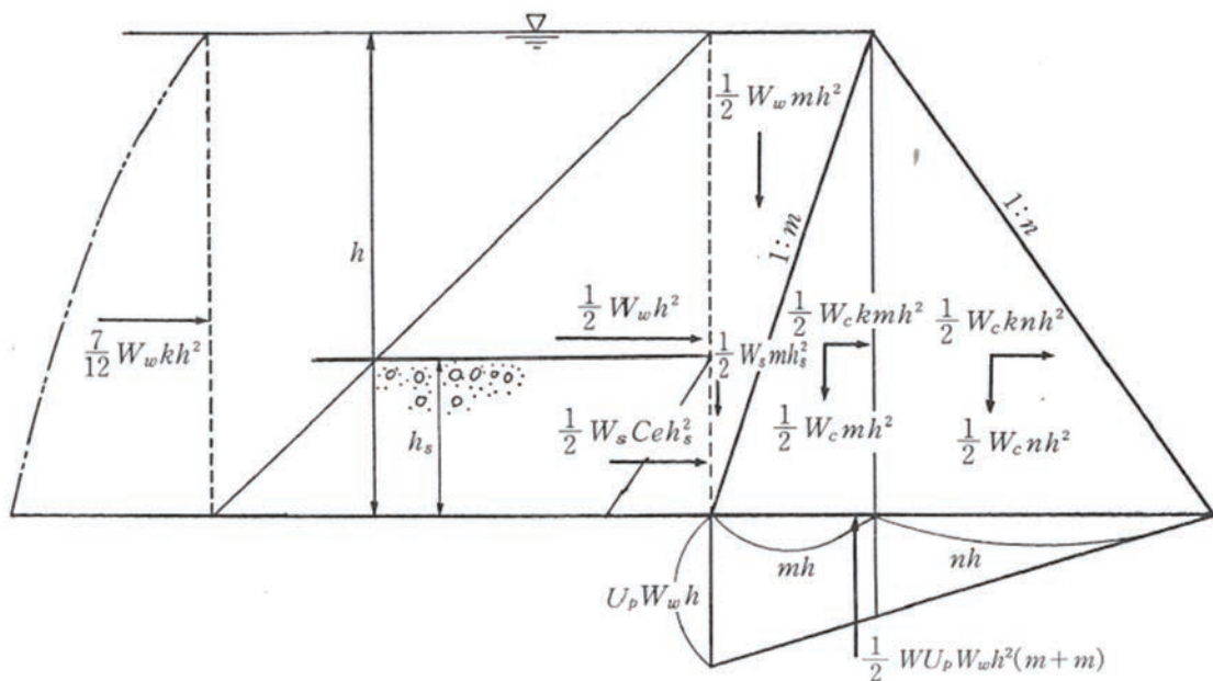
図2-4-4 外 力
