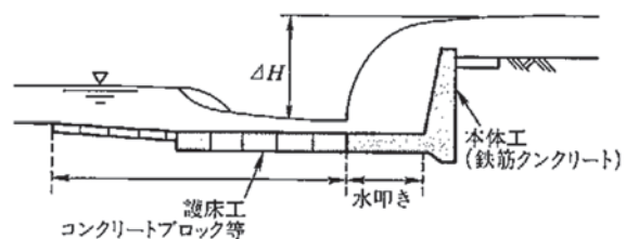
図6-7 一体式構造
