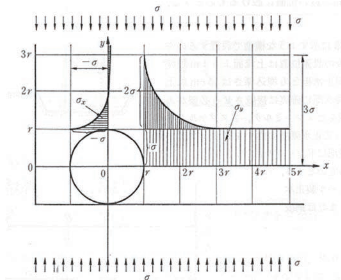
図2-4-16 空洞部周辺の応力分布
