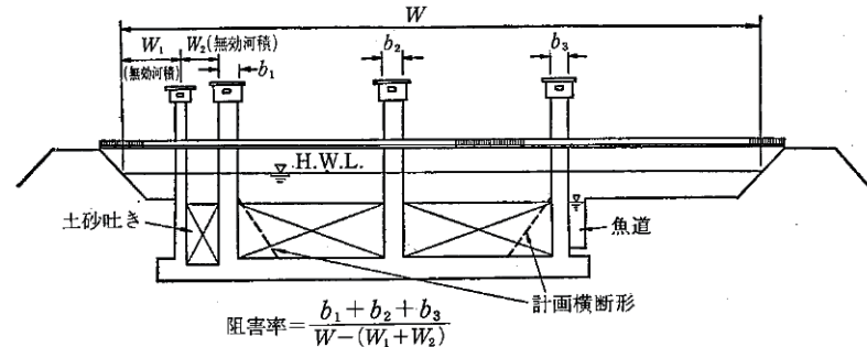
図7-3 堰の阻害率
