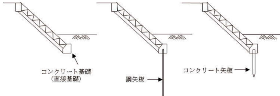
図 1-4-10 基礎工の例
