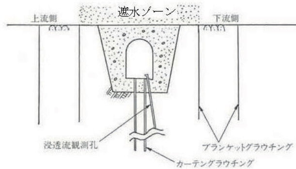
図2-5-20 通廊断面図
