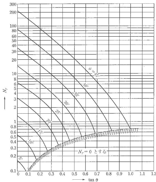
図7-10 支持力係数 N_r を求めるグラフ
