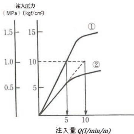
図2-6-7 P-Q 曲線とルジオン値の決め方
