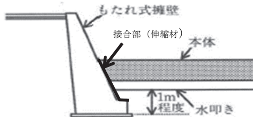
図6-23 取付擁壁
