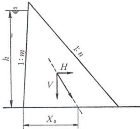
図2-4-5 重力式コンクリートダムに作用する合力の作用点
