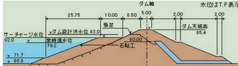
図2-11-2 アースダムのかさ上げ
