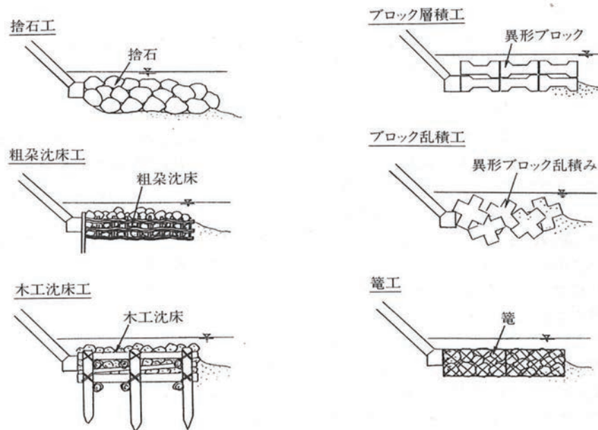
図1-4-11 代表的な根固工
