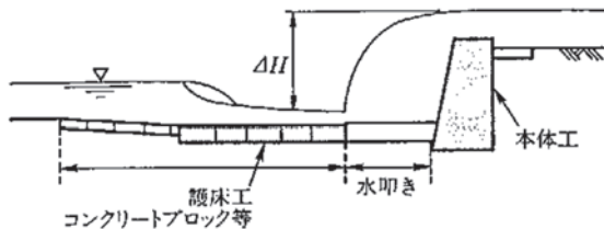
図6-6 分離式構造
