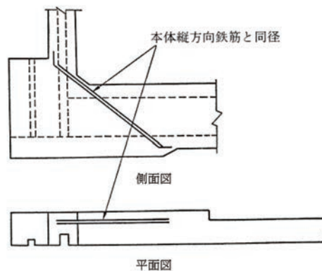
図8-13 門柱と函渠接続部の配筋
