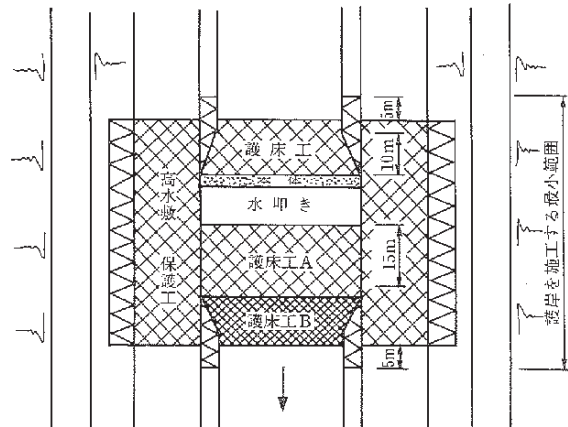
図6-21 床止めの設置に伴い必要となる護岸を設置する最小範囲
