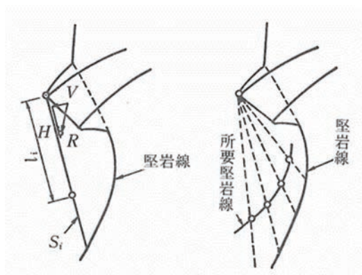
図2-2-7 所要堅岩線
