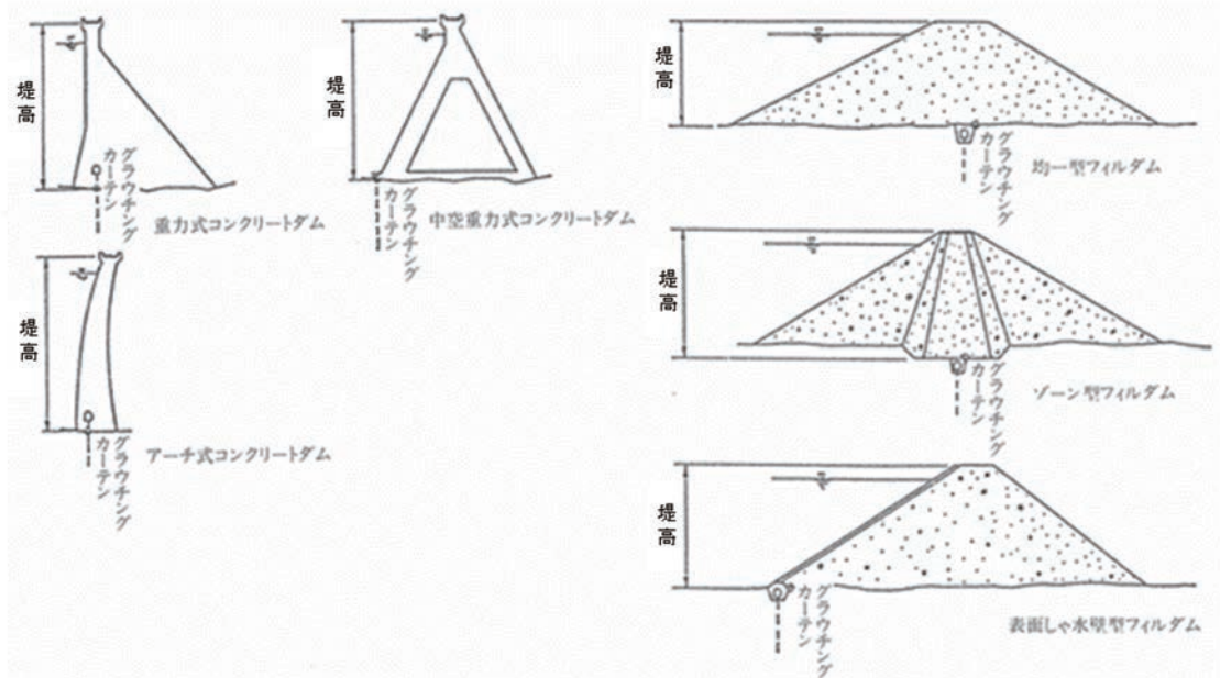
図2-1-1 各種のダムの高さ
