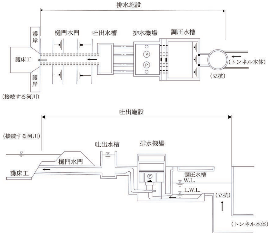
図10-8 排水施設の例
