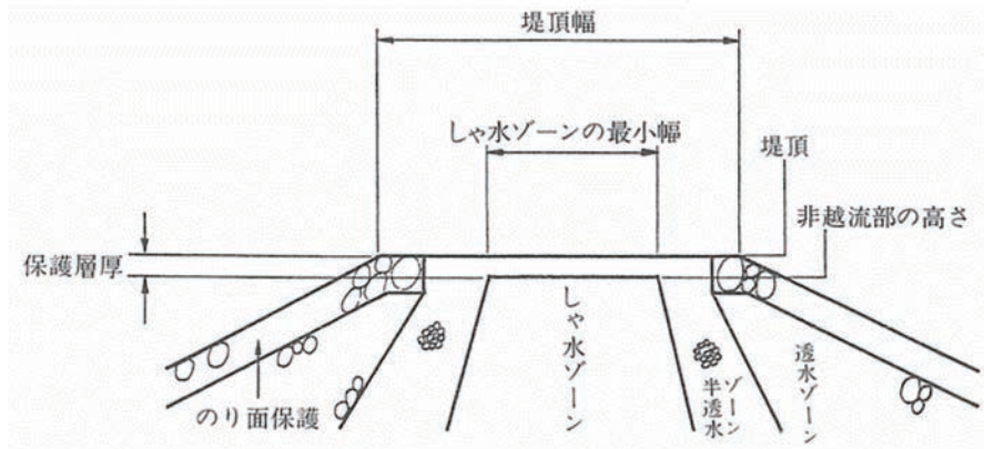
図2-2-1 ダム堤頂付近標準図
