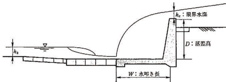
図6-16 完全越流時の水面形状
