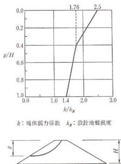
図2-5-16 堤体震力係数
