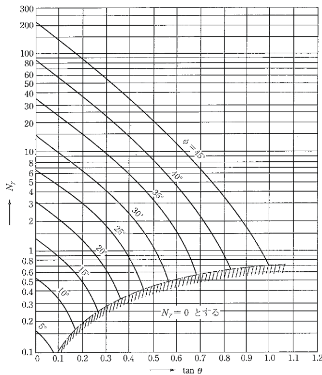
図7-10 支持力係数 N_γ を求めるグラフ
