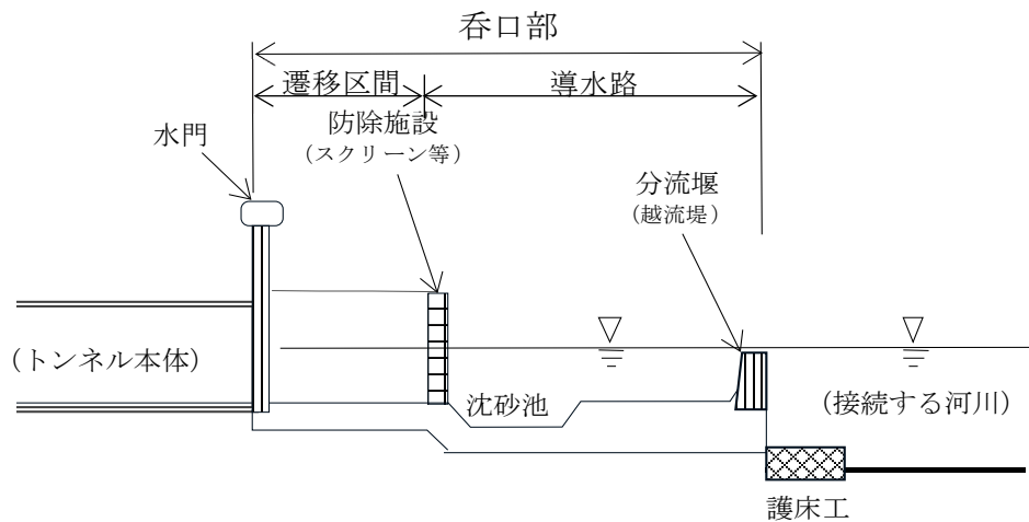
図10-5 呑口部の例
