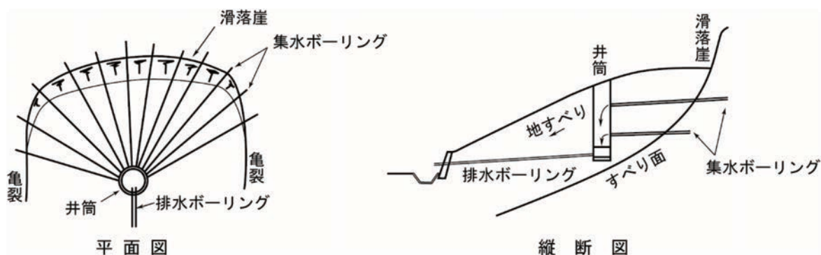
図 4-3-9 集水井工
