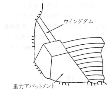
図2-4-10 重力式アバットメント及びウイングダム
