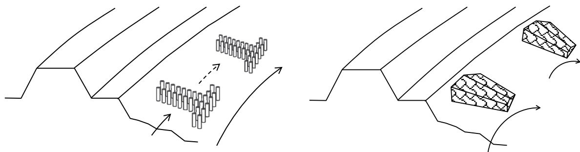
透過水制の例（杭出）
