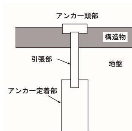
図 4-7-1 グラウンドアンカー工の構成要素
