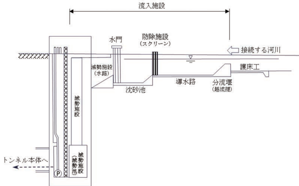
図10-6 流入施設の例
