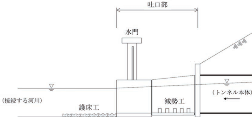
図10-7 吐口部の例
