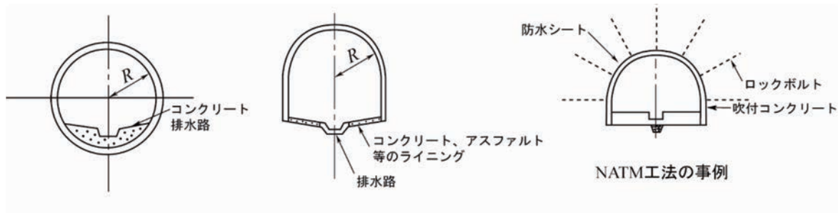
図 4-3-13 排水トンネルの断面形状の事例
