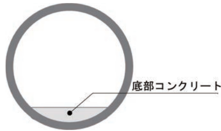
図10-3 維持管理に配慮した断面設定のイメージ
