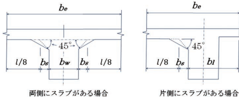
図10-4 T形ばりの圧縮突縁の有効幅
