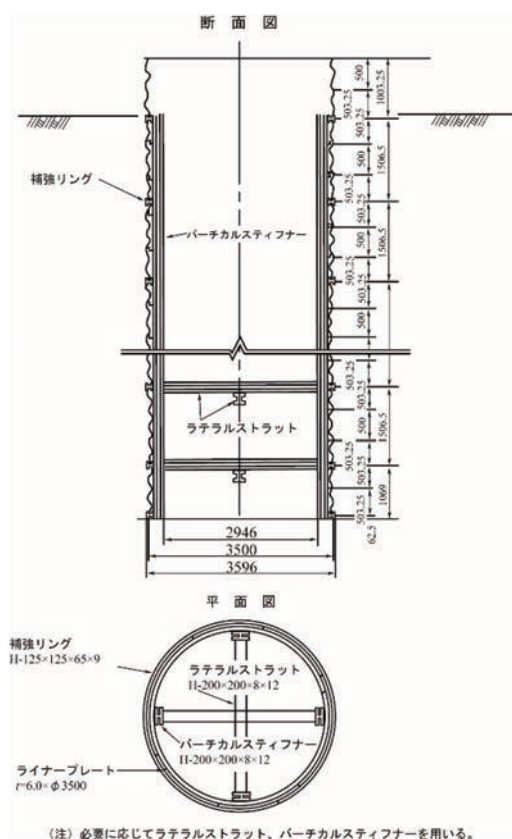
図 4-3-10 ライナープレートによる井筒の例（単位：mm）
