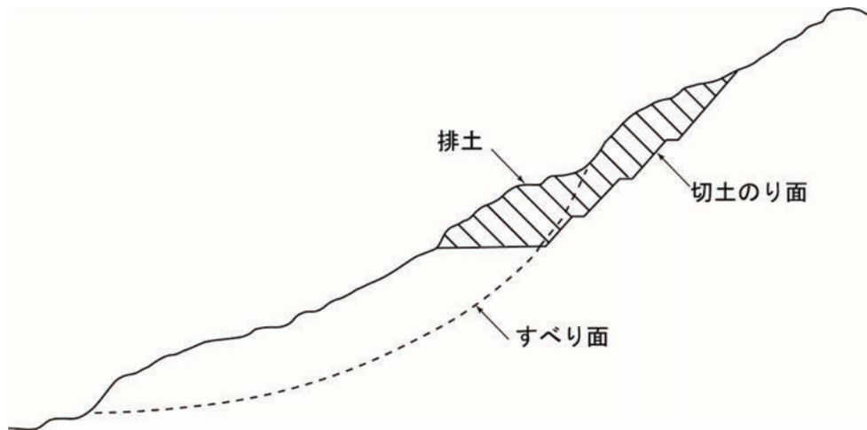
図 4-4-1 排土工と切土のり面の例
