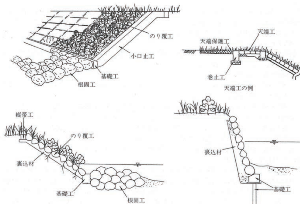
図 1-4-5 護岸の構成
