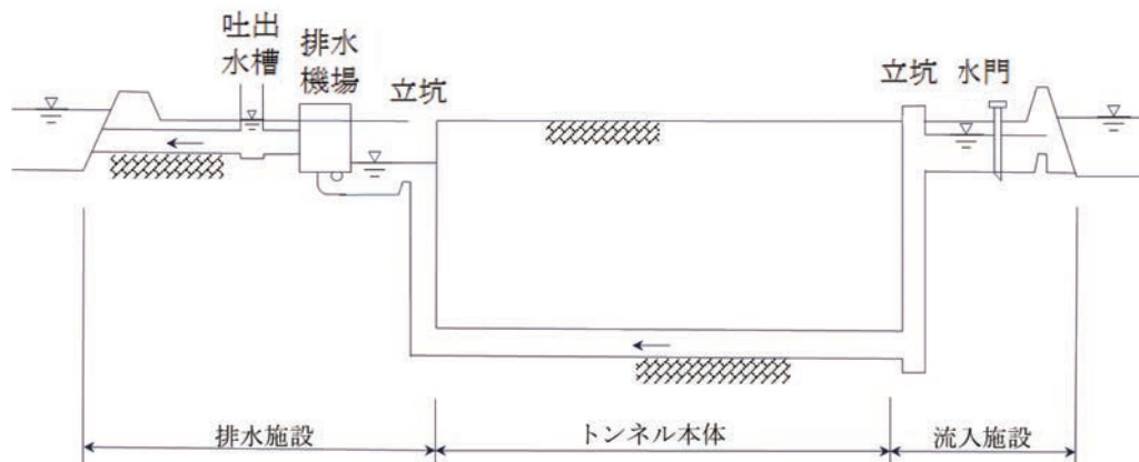
図10-2 各構造の名称（圧力管形式）
