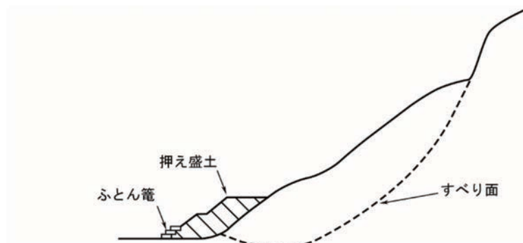
図 4-4-2 押え盛土工
