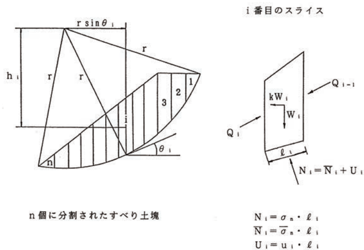
図2-5-17 スライス法
