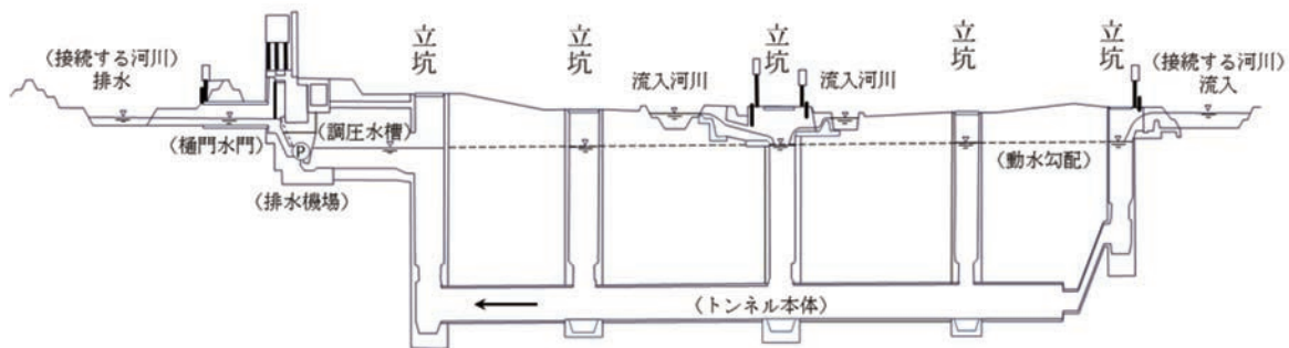
図10-10 シールド工法の立坑の例
