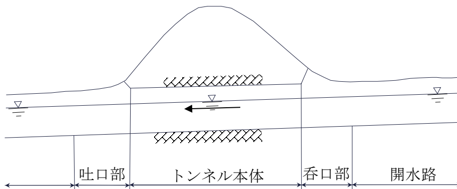
図10-1 各構造の名称（開水路形式）
