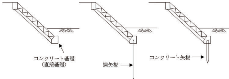
図 1-4-10 基礎工の例
